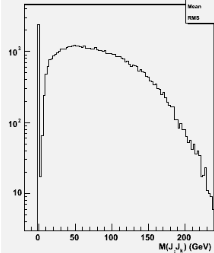
2jets mass(All comb)w103156 e1a_e1n2e2e2n2_o
