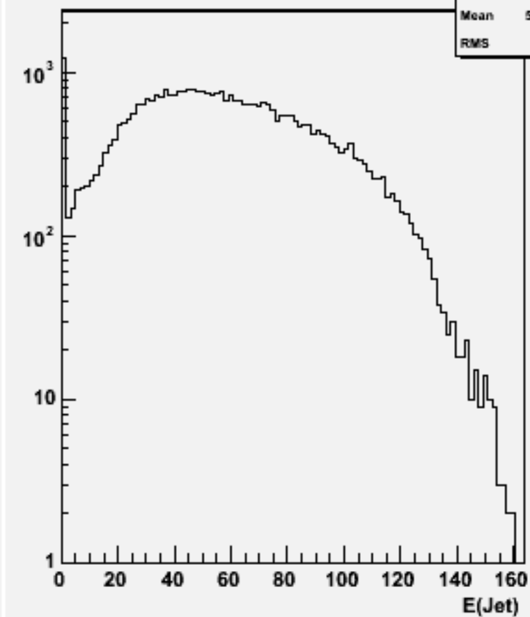
Jet energies(All jets)w103156 e1a_e1n2e2e2n2_o
