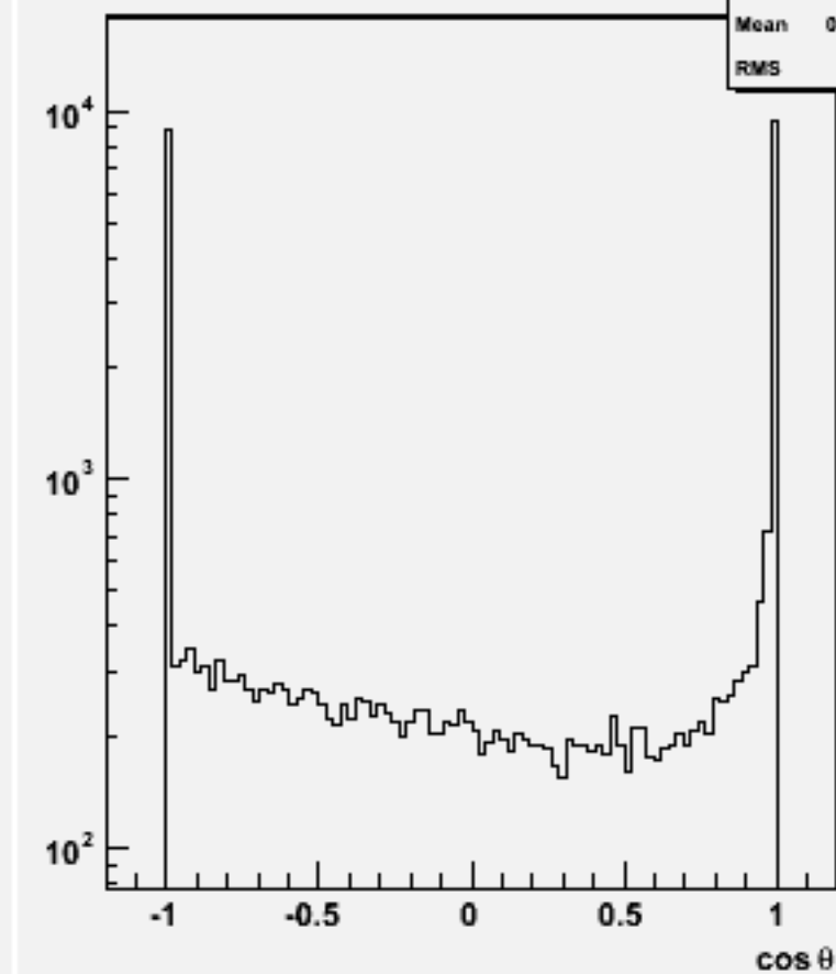
Jet cos \theta (All jets)w103156 e1a_e1n2e2e2n2_o
