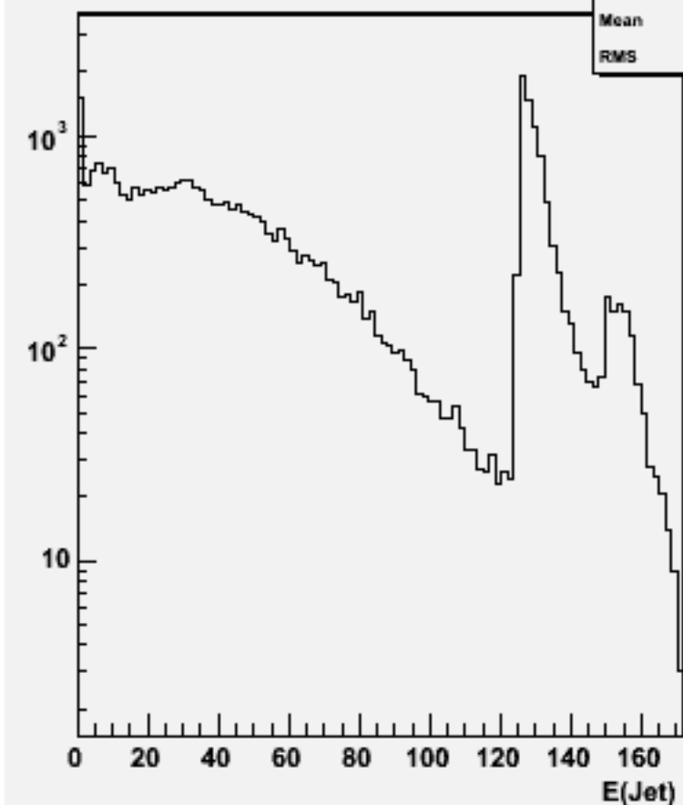
Jet energies(All jets)w103155 e1a_e1n2e2e2n2_o
