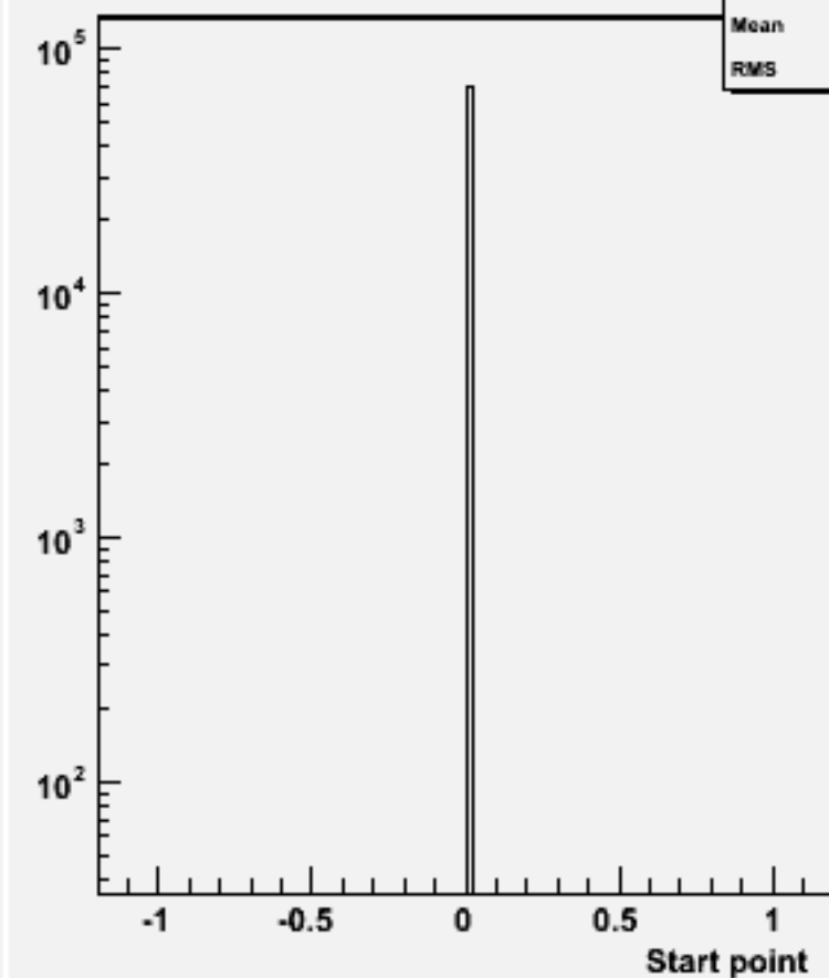
Start point Z : w103155 e1a_e1n2e2e2n2_o
