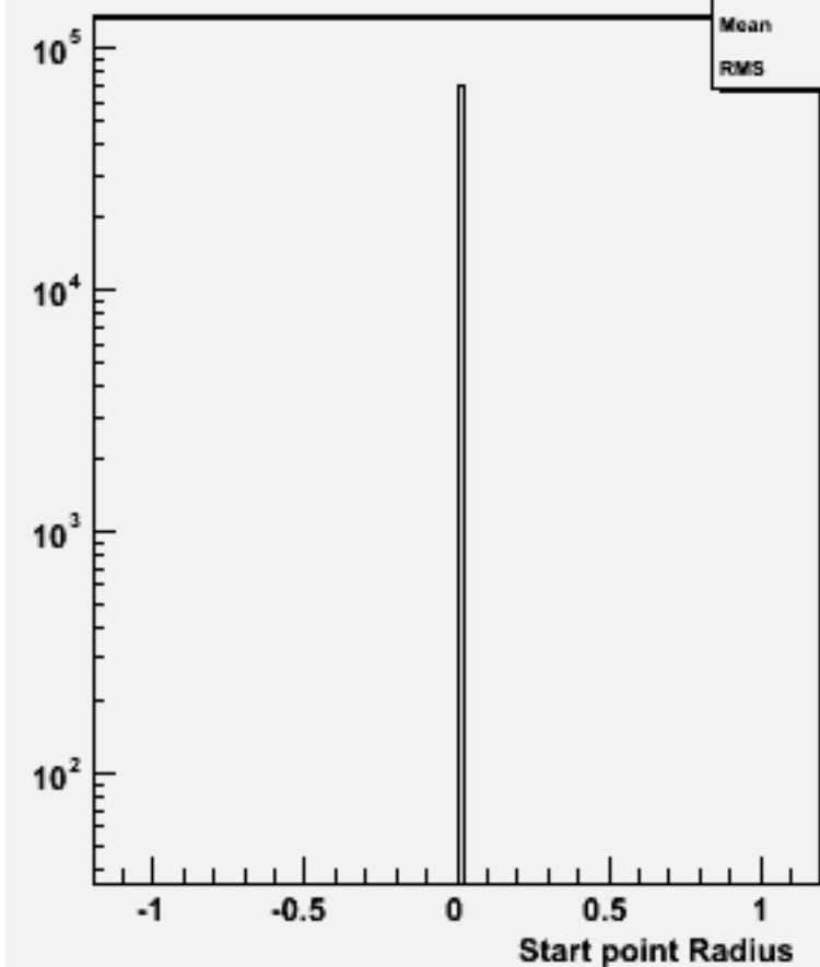
Start point R : w103155 e1a_e1n2e2e2n2_o
