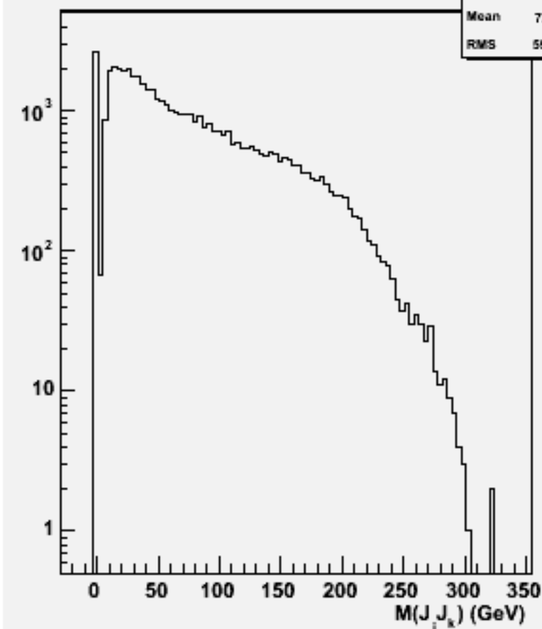
2jets mass(All comb)w103155 e1a_e1n2e2e2n2_o
