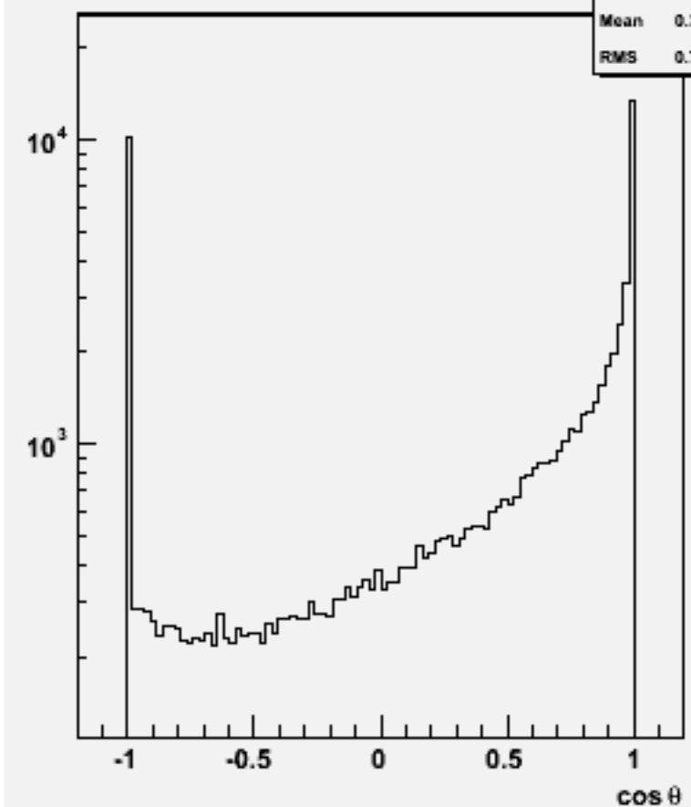
Particle cos \theta : w103155 e1a_e1n2e2e2n2_o
