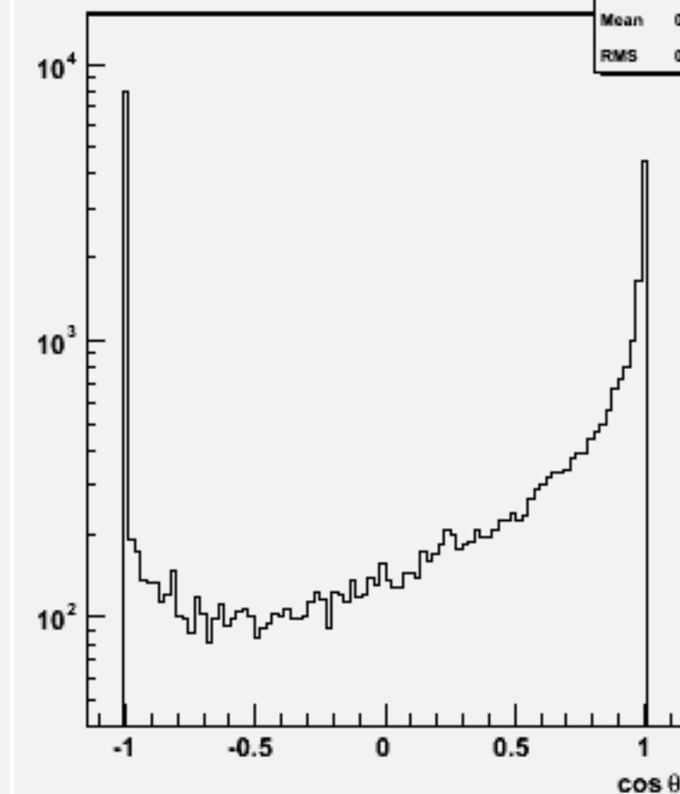
Jet cos \theta (All jets)w103155 e1a_e1n2e2e2n2_o
