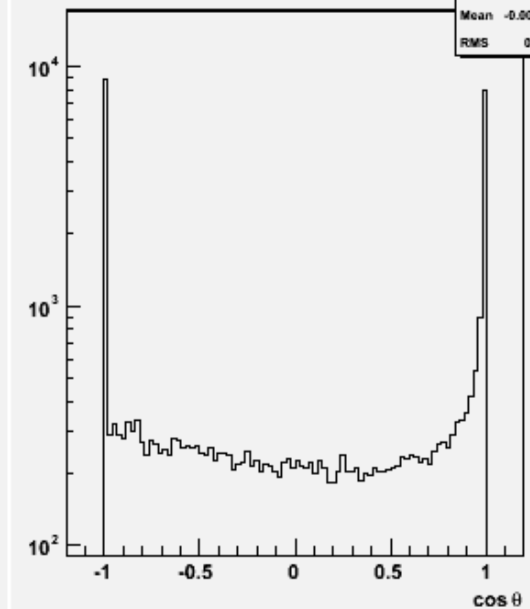
Jet cos \theta (All jets)w103154 e1a_e1n2e2e2n2_o
