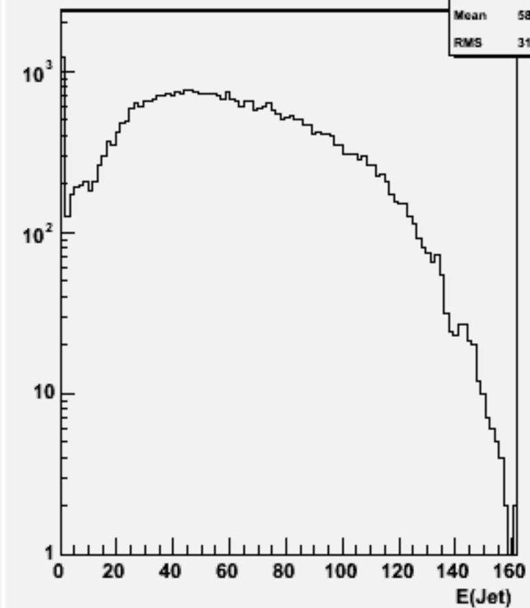
Jet energies(All jets)w103154 e1a_e1n2e2e2n2_o
