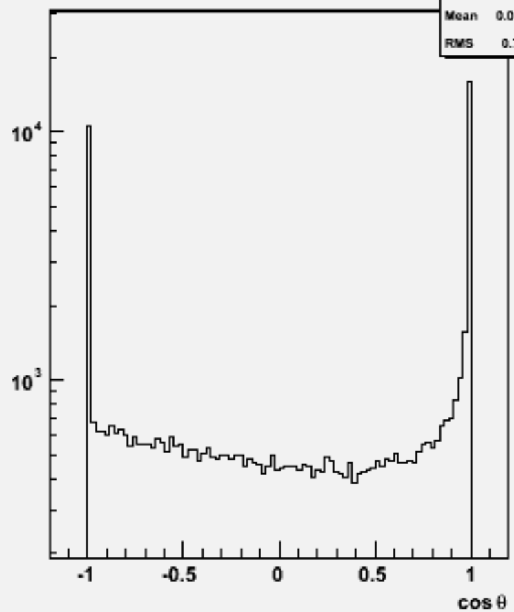
Particle cos \theta : w103154 e1a_e1n2e2e2n2_o
