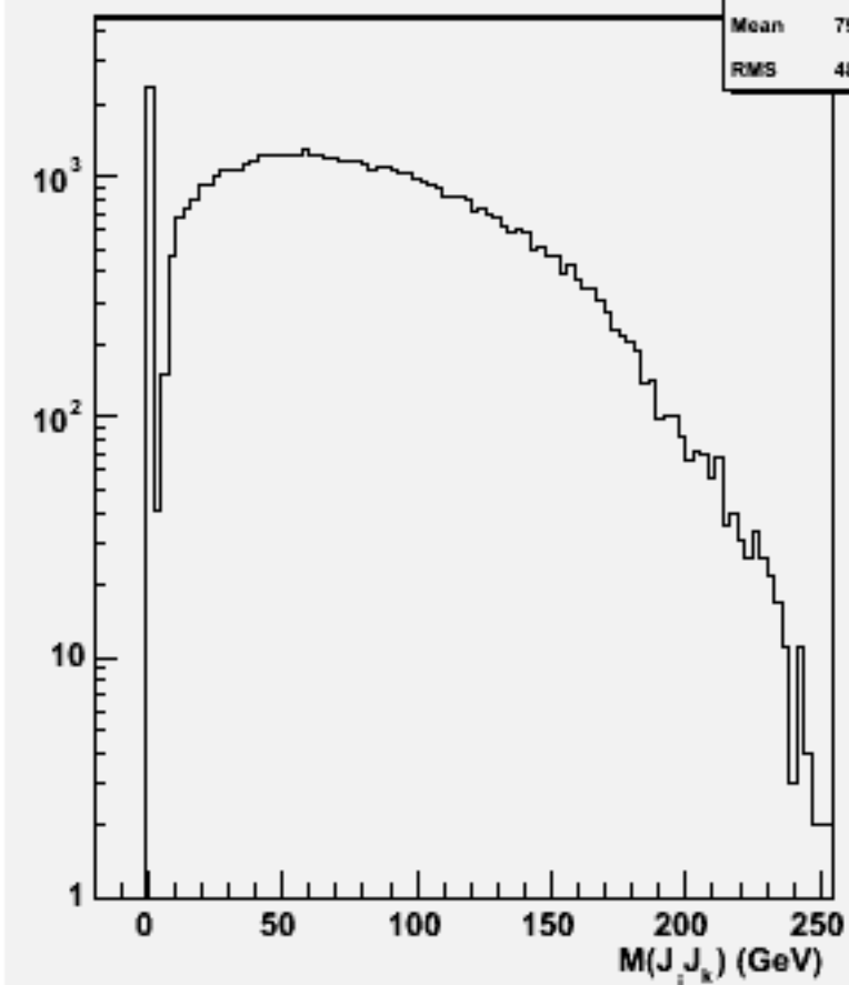
2jets mass(All comb)w103154 e1a_e1n2e2e2n2_o
