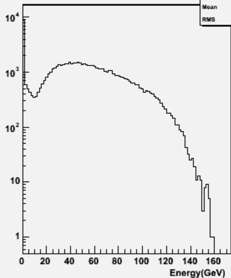
Start point R : w103154 e1a_e1n2e2e2n2_o
