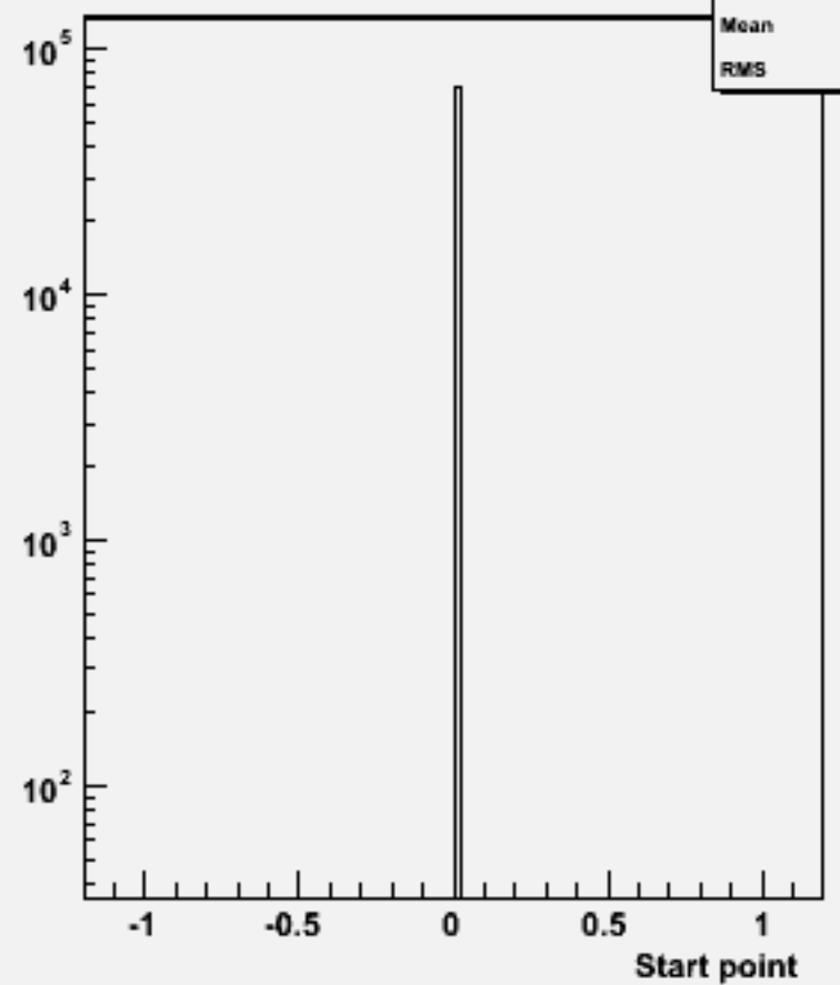
Start point Z : w103154 e1a_e1n2e2e2n2_o
