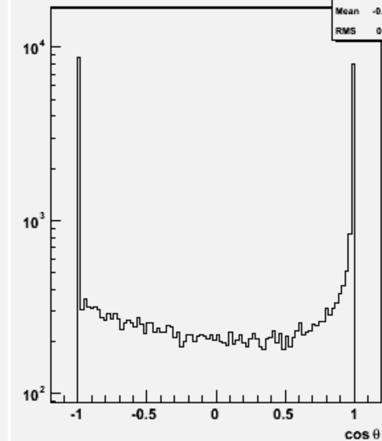
Jet cos \theta (All jets)w103150 e1a_e1n2e2e1n1_o
