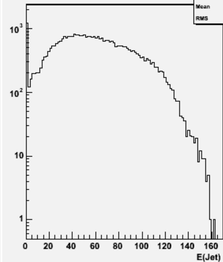
Jet energies(All jets)w103150 e1a_e1n2e2e1n1_o
