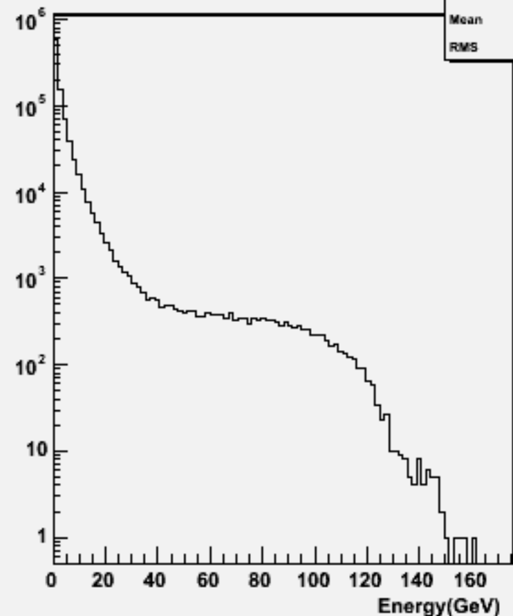
Particle Energy : w103146 e1a_n1bbsc_o
