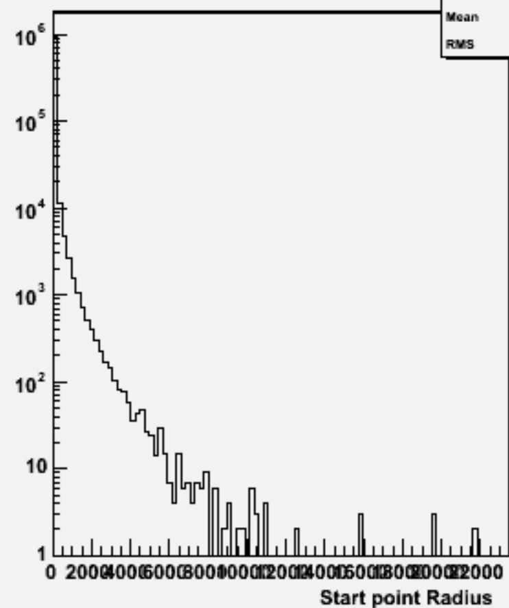
Start point R : w103146 e1a_n1bbsc_o
