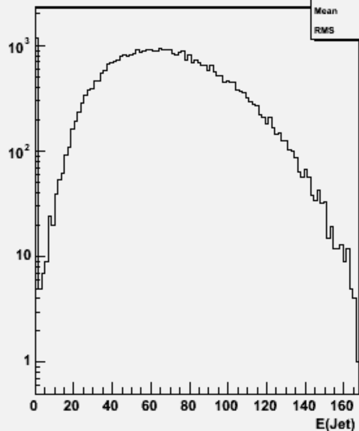
Jet energies(All jets)w103146 e1a_n1bbsc_o
