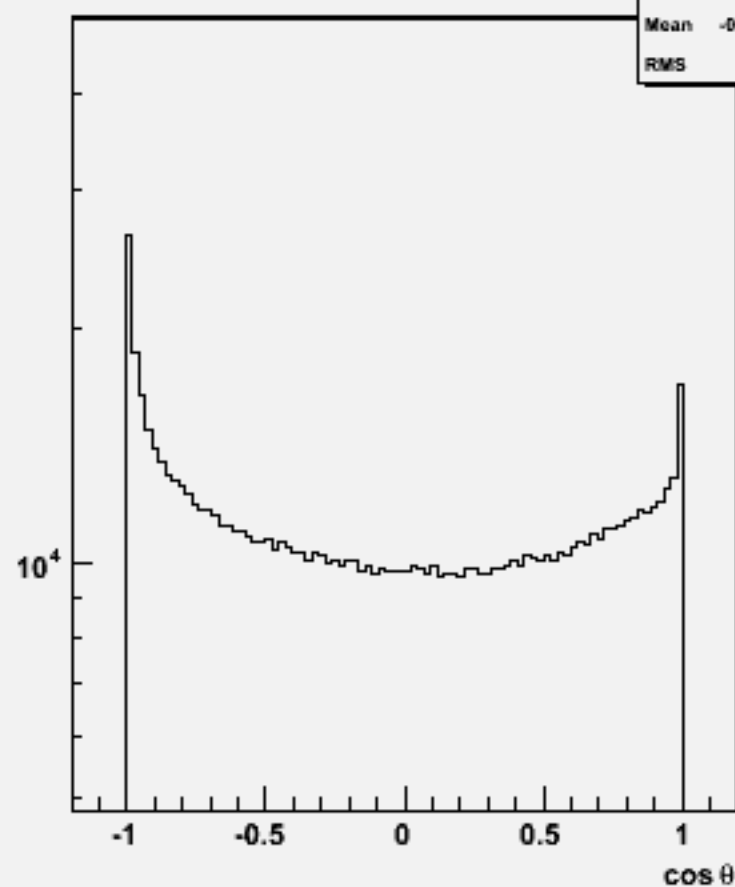
Particle cosθ : w103146 e1a_n1bbsc_o
