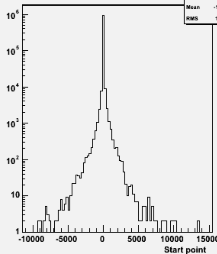
Start point Z : w103146 e1a_n1bbsc_o
