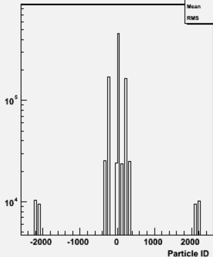
Particle ID : w103146 e1a_n1bbsc_o
