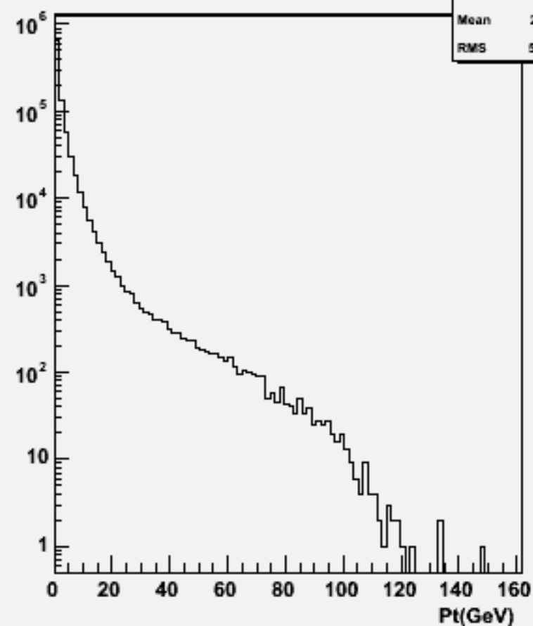
Particle Pt : w103146 e1a_n1bbsc_o
