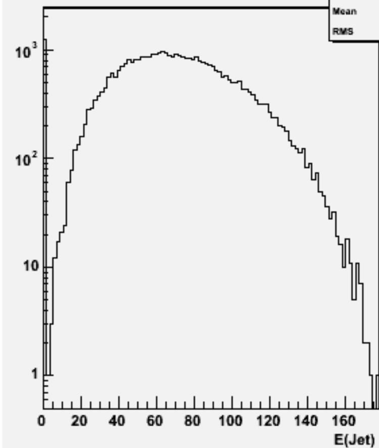
Jet energies(All jets)w103126 e1a_n1sssc_o
