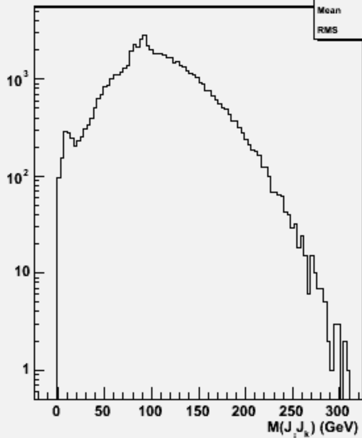
2jets mass(All comb)w103102 e1a_n1dd1du_o
