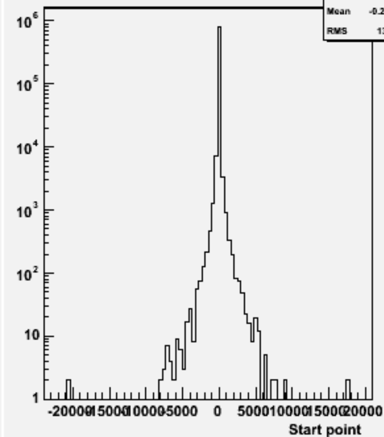
Start point Z : w103102 e1a_n1dd1du_o
