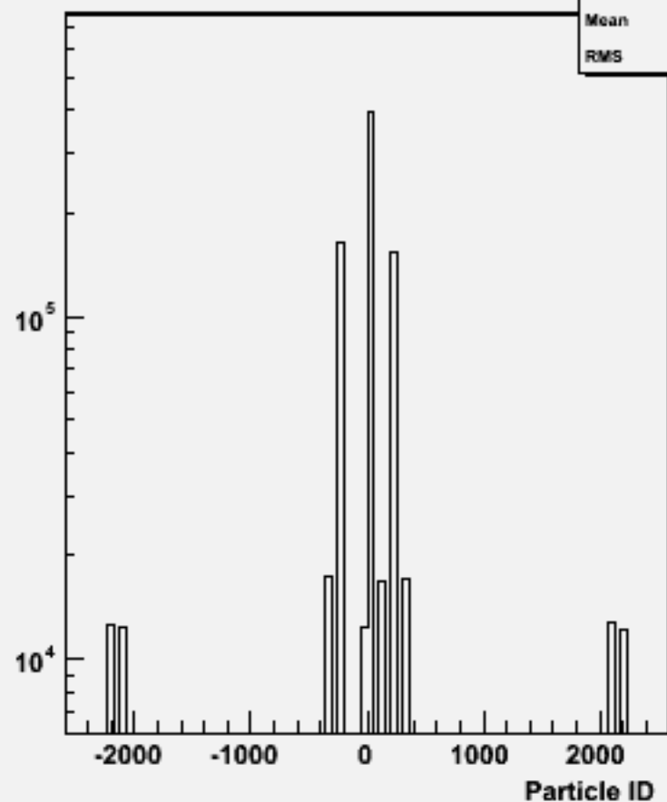
Particle ID : w103102 e1a_n1dd1du_o
