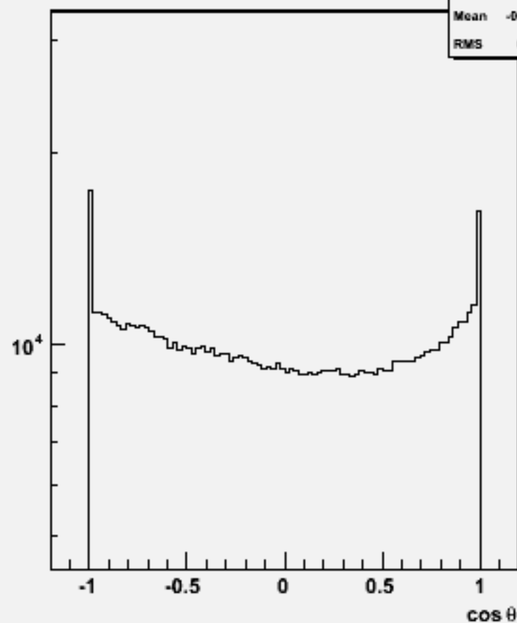
Particle cos \theta : w103102 e1a_n1dd1du_o
