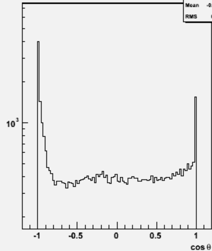
Jet cosθ (All jets)w103102 e1a_n1dd1du_o
