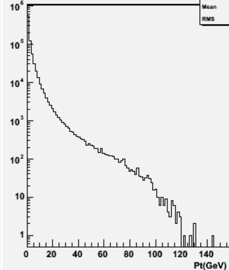
Particle Pt : w103102 e1a_n1dd1du_o
