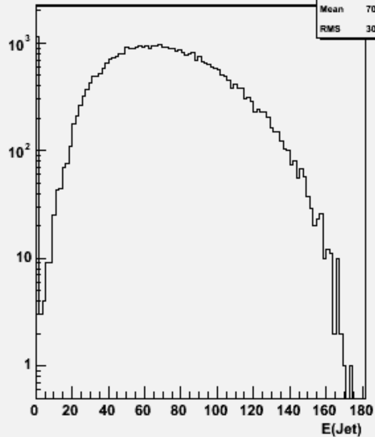
Jet energies(All jets)w103102 e1a_n1dd1du_o
