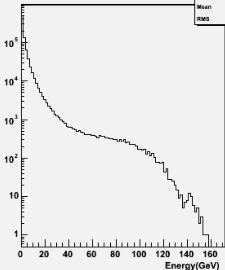
Particle Energy : w103102 e1a_n1dd1du_o
