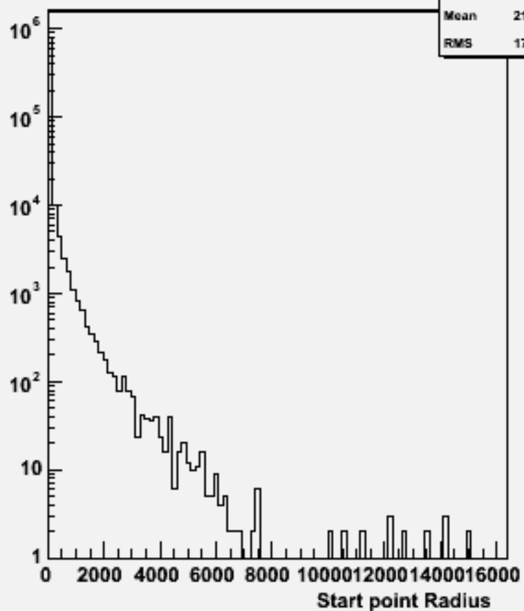
Start point R : w103102 e1a_n1dd1du_o
