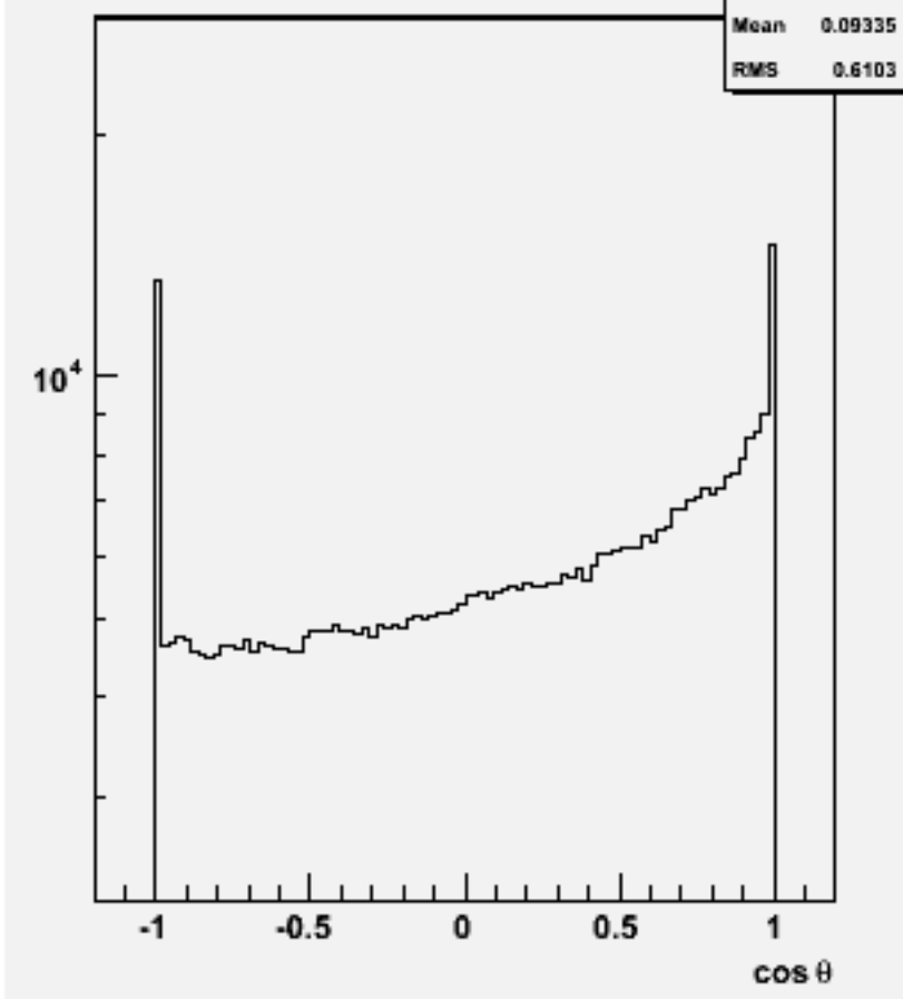
Particle cos \theta : w103098 e1a_n1dde3n3_o
