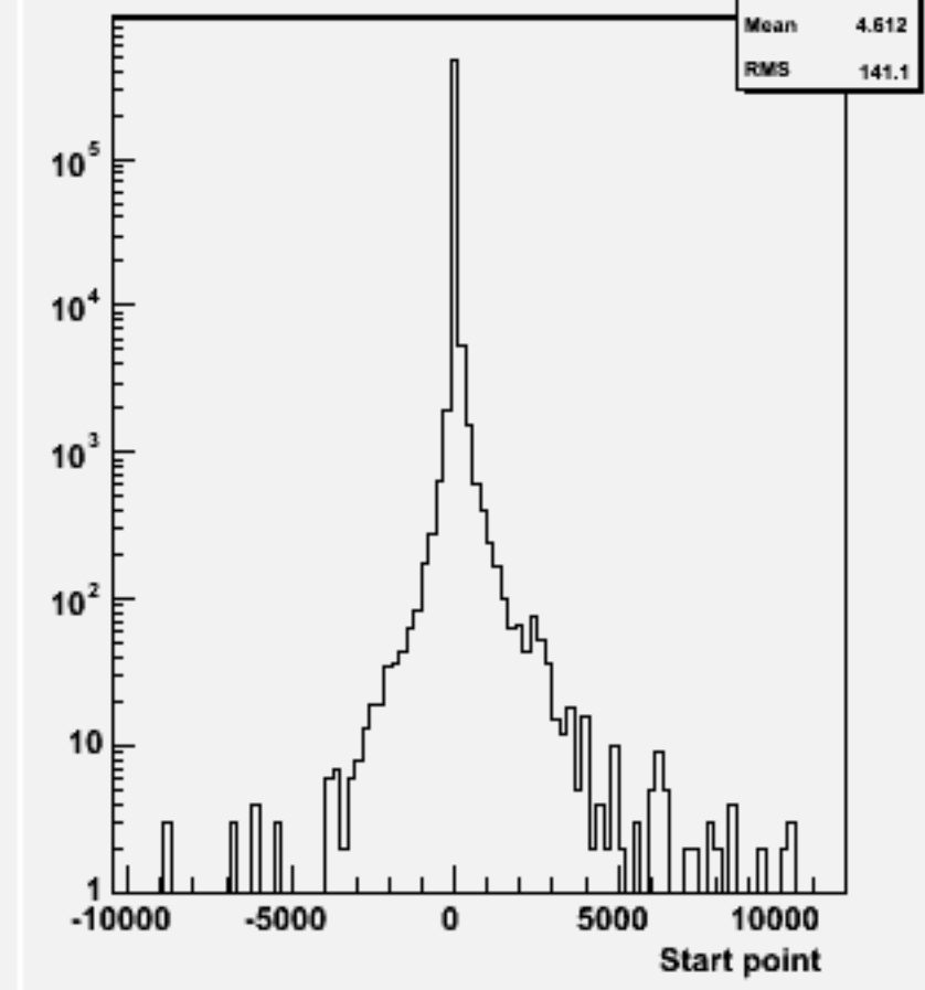
Start point Z : w103098 e1a_n1dde3n3_o
