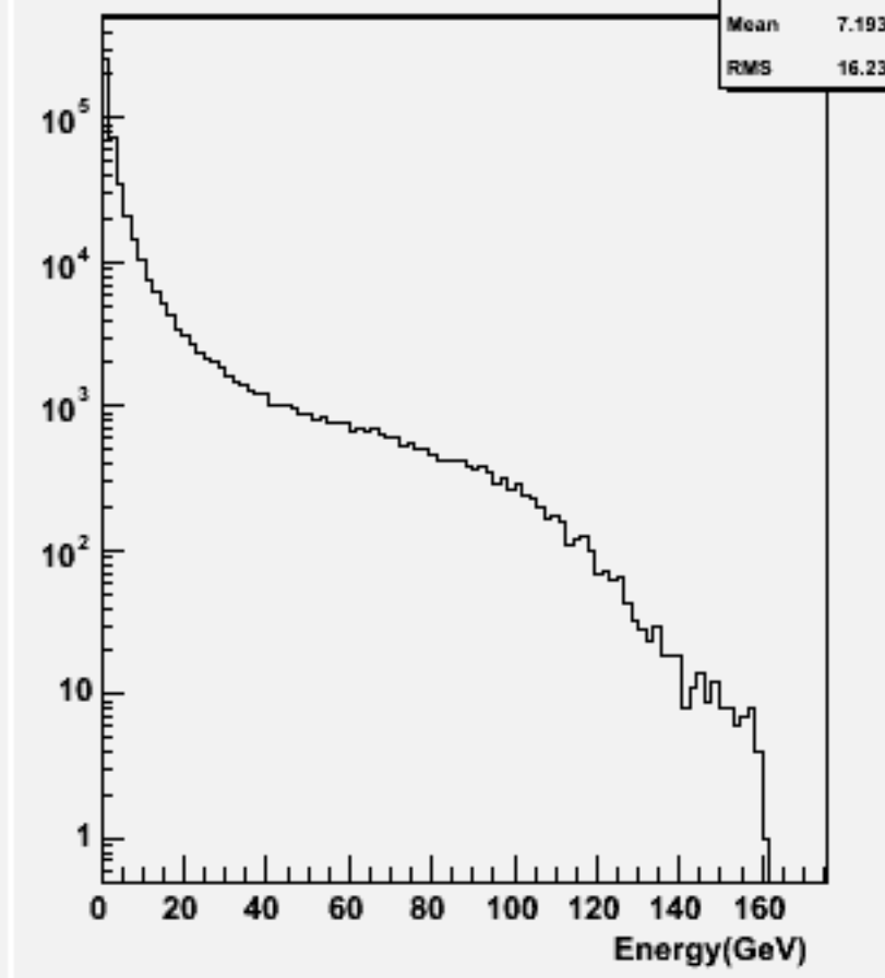
Start point R : w103098 e1a_n1dde3n3_o
