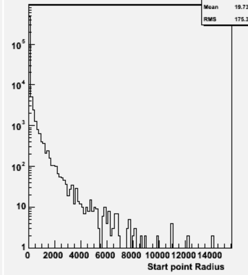
Start point R : w103098 e1a_n1dde3n3_o
