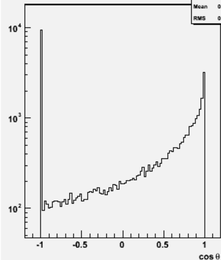
Jet cos theta (All jets)w103087 e1a_n1e3e3sc_o
