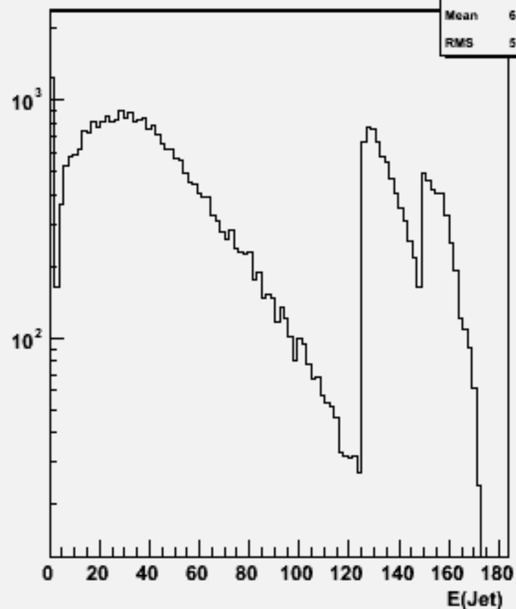
Jet energies(All jets)w103087 e1a_n1e3e3sc_o
