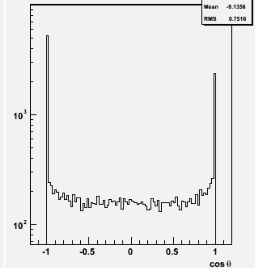
Jet cos \theta (All jets)w103078 e1a_n1e3e3e3n3_o
