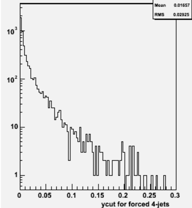
Ycut for 4-jets :w103078 e1a_n1e3e3e3n3_o
