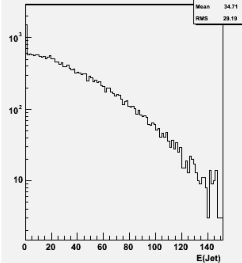
Jet energies(All jets)w103078 e1a_n1e3e3e3n3_o
