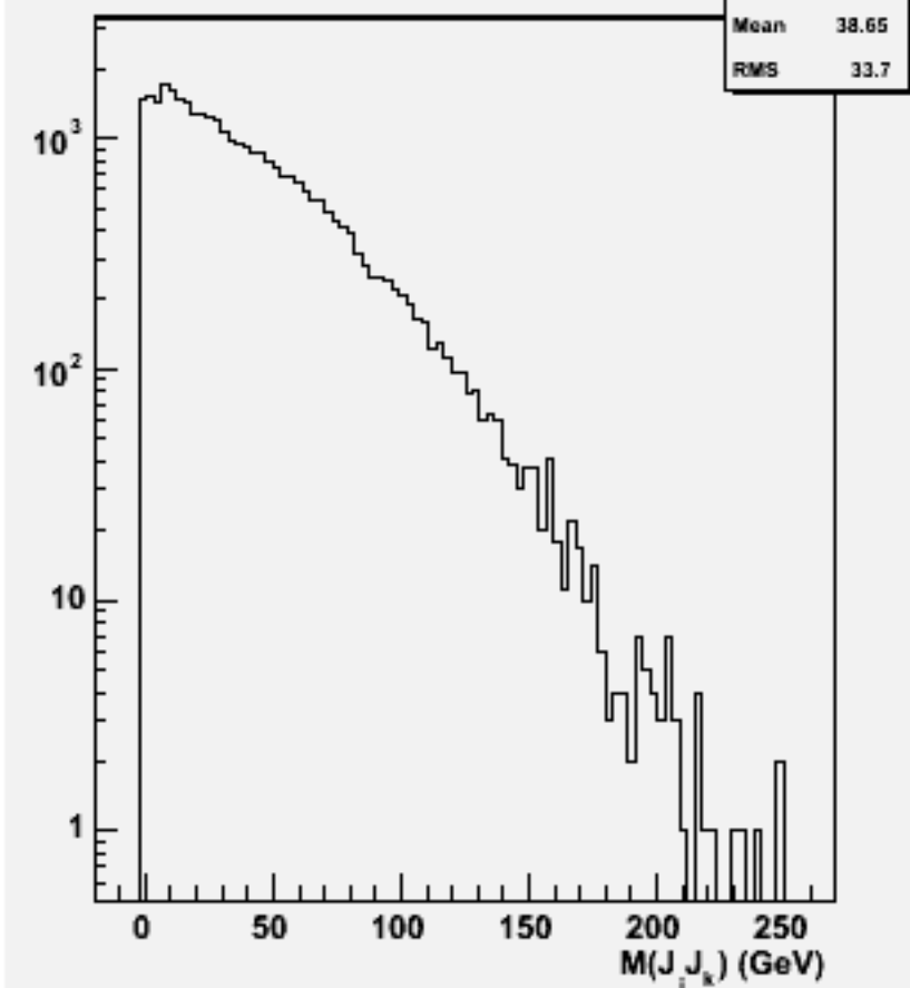
2jets mass(All comb)w103078 e1a_n1e3e3e3n3_o
