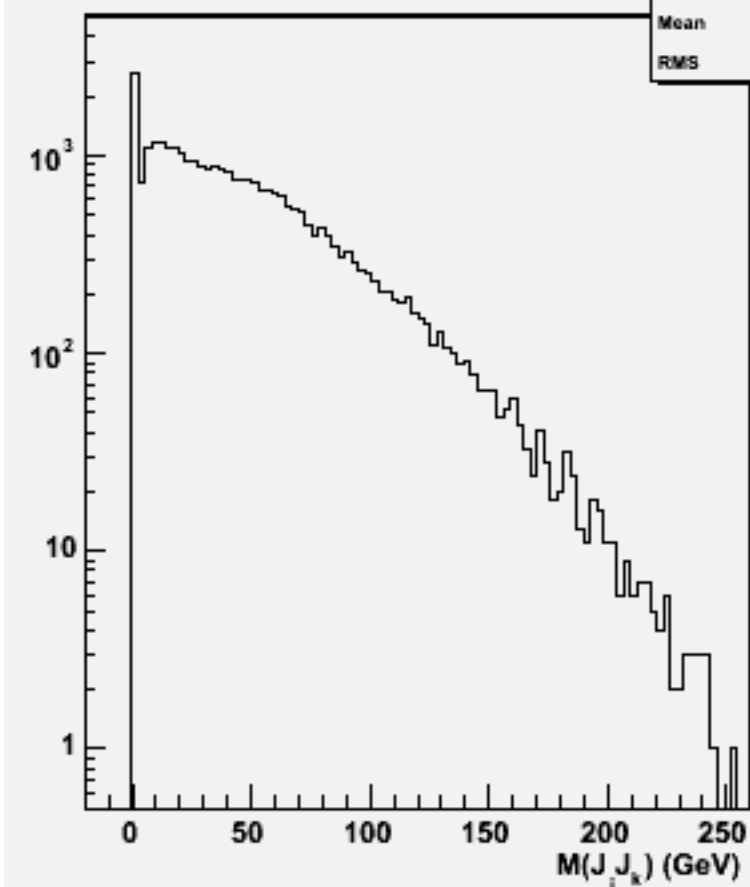
2jets mass(All comb)w103070 e1a_n1e3e3e1n1_o
