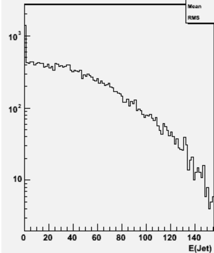
Jet energies(All jets)w103070 e1a_n1e3e3e1n1_o
