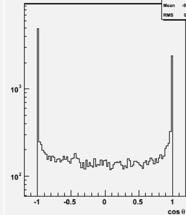
Jet cos \theta (All jets)w103070 e1a_n1e3e3e1n1_o
