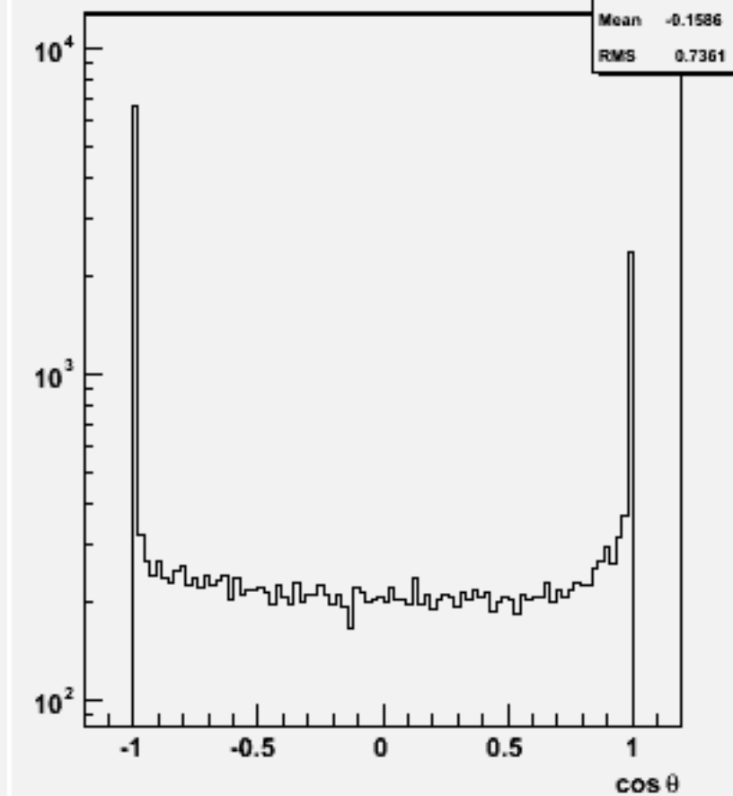
Jet cos \theta (All jets)w103054 e1a_n1e2e2n2_o
