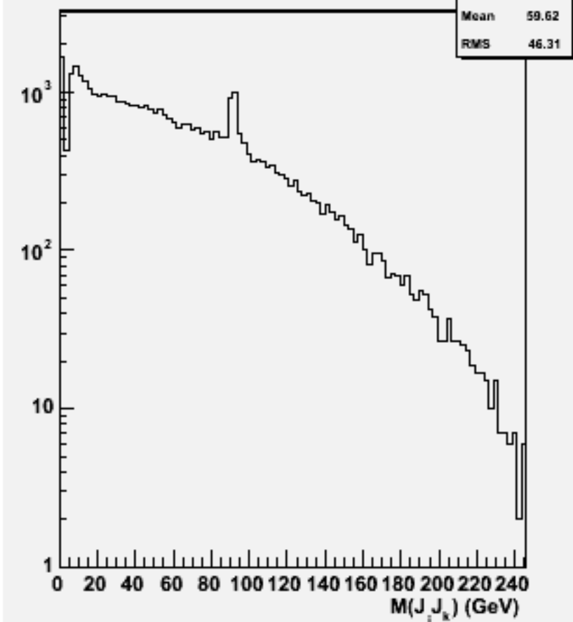
2jets mass(All comb)w103054 e1a_n1e2e2n2_o
