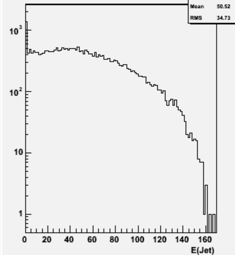
Jet energies(All jets)w103054 e1a_n1e2e2n2_o
