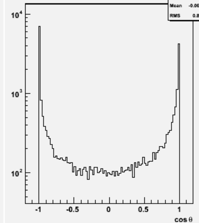
Jet cos \theta (All jets)w103052 e1a_n1e2e1n1_o
