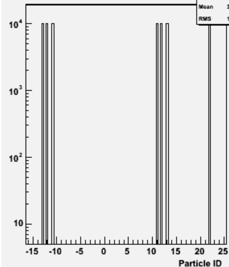
Particle ID : w103052 e1a_n1e2e2e1n1_o
