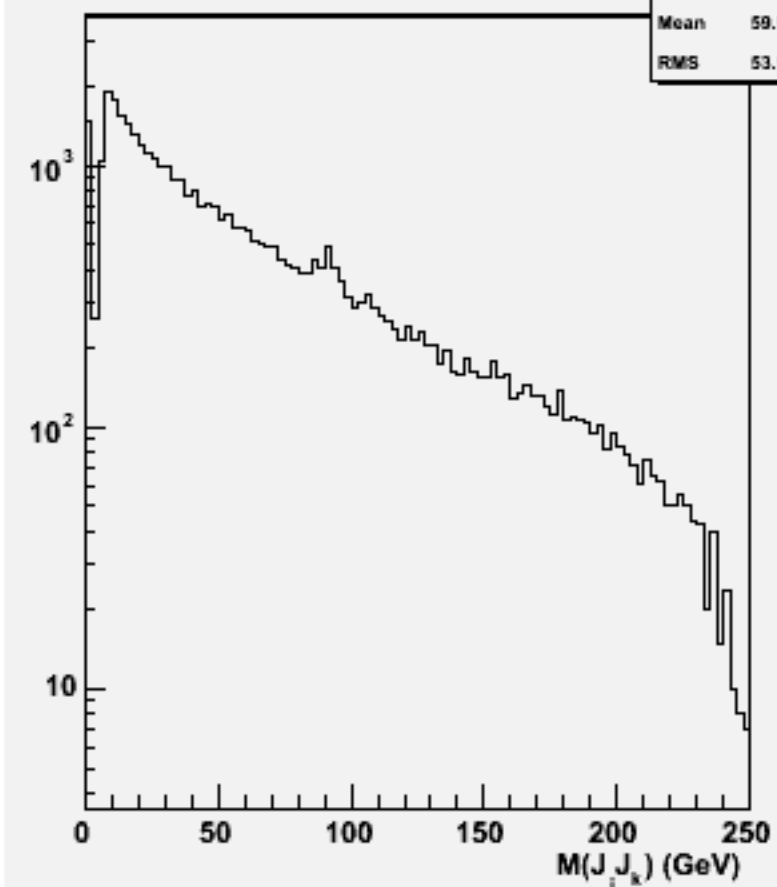
2jets mass(All comb)w103052 e1a_n1e2e1n1_o
