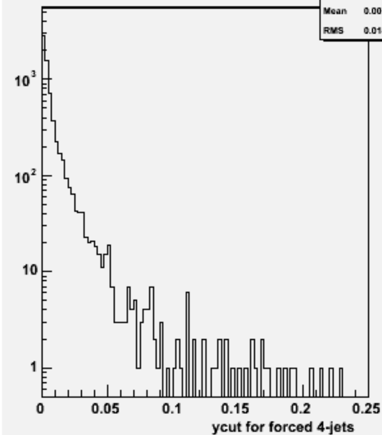
Ycut for 4-jets :w103052 e1a_n1e2e1n1_o
