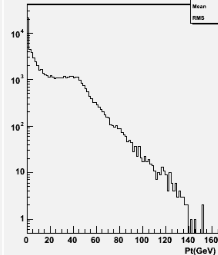
Particle Pt : w103052 e1a_n1e2e2e1n1_o
