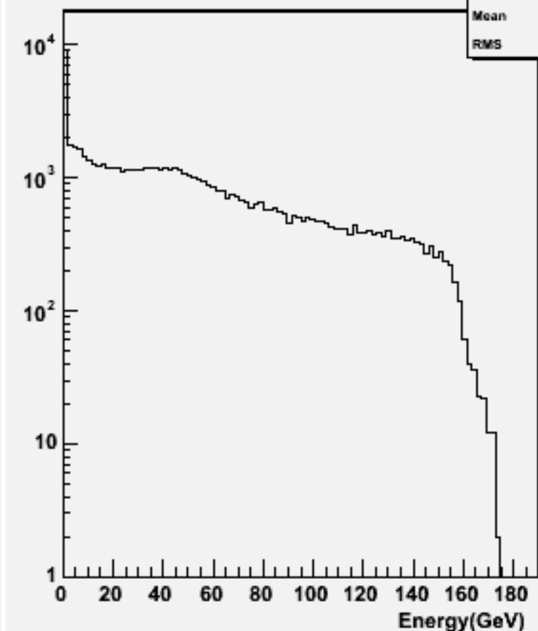
Particle Energy : w103052 e1a_n1e2e2e1n1_o
