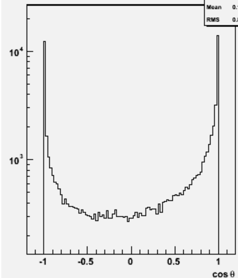
Particle cos \theta : w103052 e1a_n1e2e2e1n1_o
