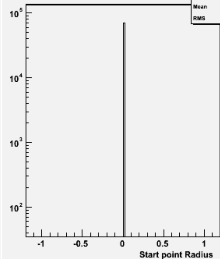
Start point R : w103052 e1a_n1e2e2e1n1_o
