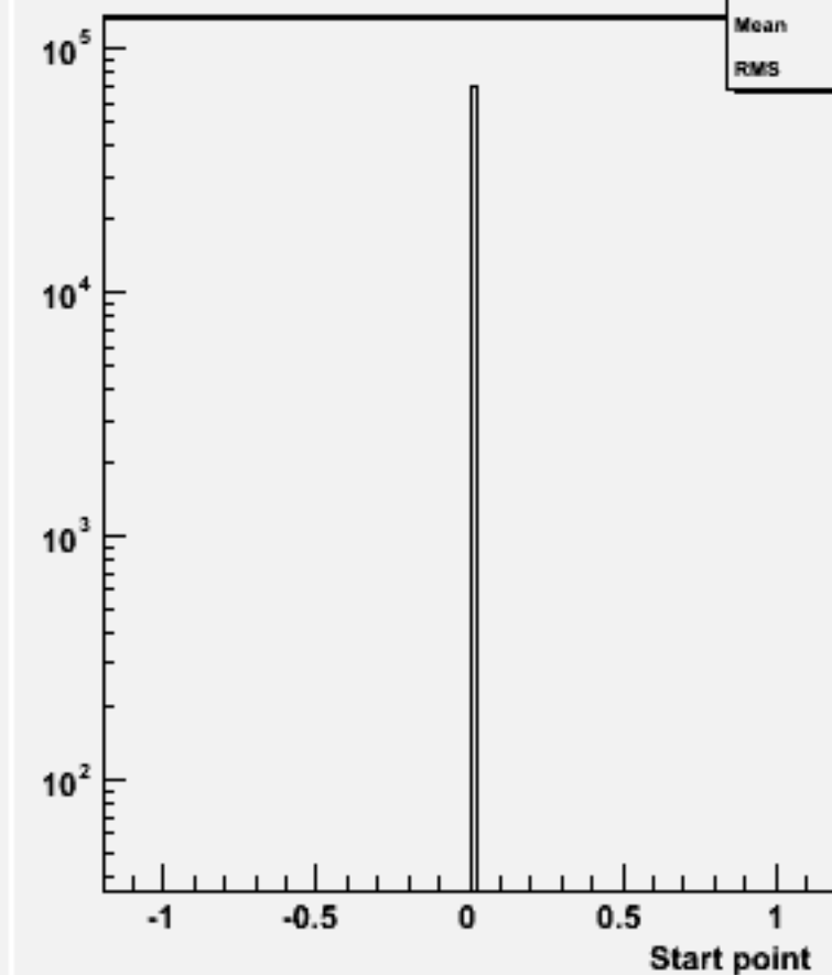
Start point Z : w103052 e1a_n1e2e2e1n1_o
