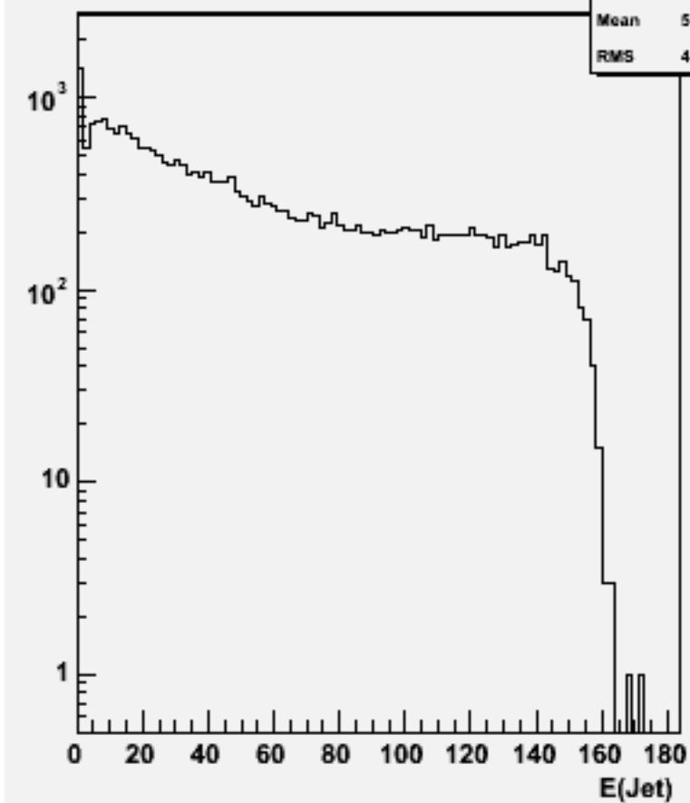
Jet energies(All jets)w103052 e1a_n1e2e1n1_o
