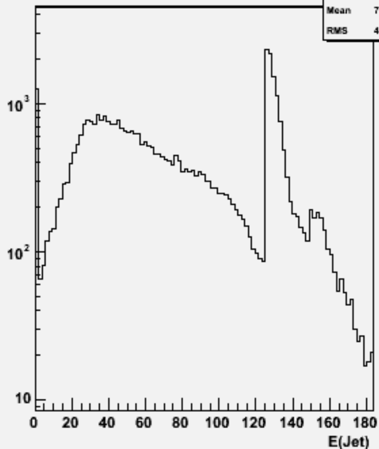
Jet energies(All jets)w103045 e1a_n1e1e1du_o
