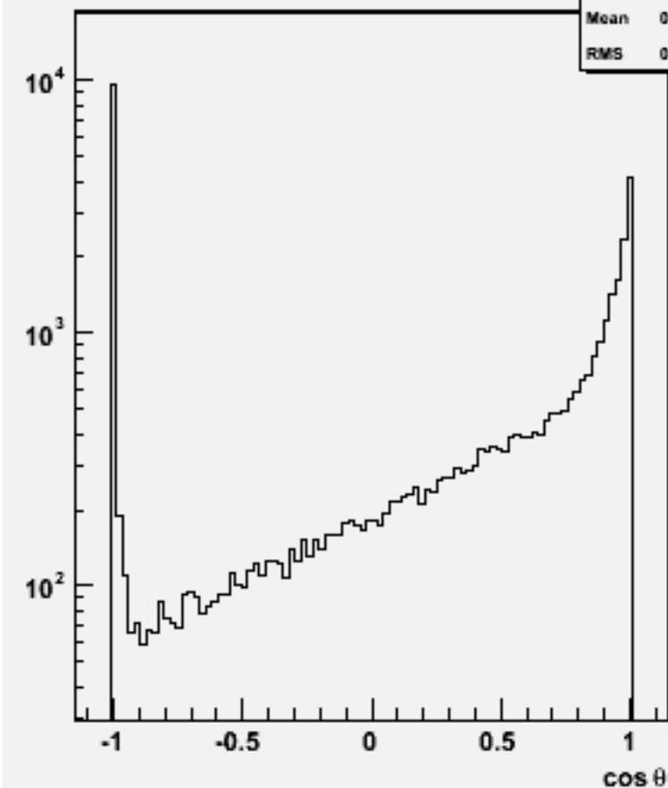
Jet cos \theta (All jets)w103045 e1a_n1e1e1du_o
