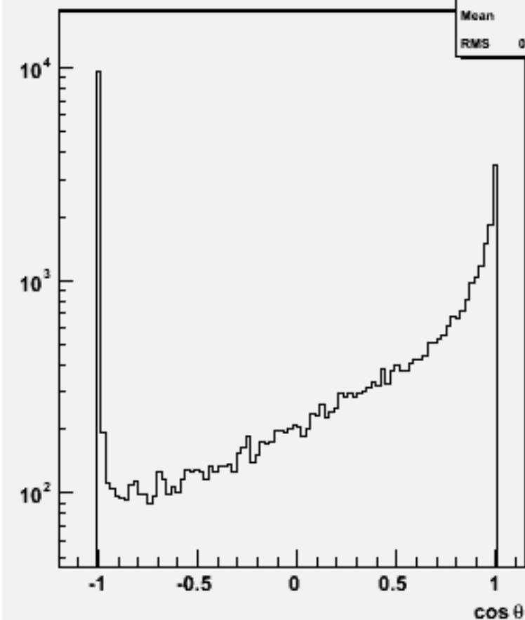
Jet cos \theta (All jets)w103043 e1a_n1e1e1du_o
