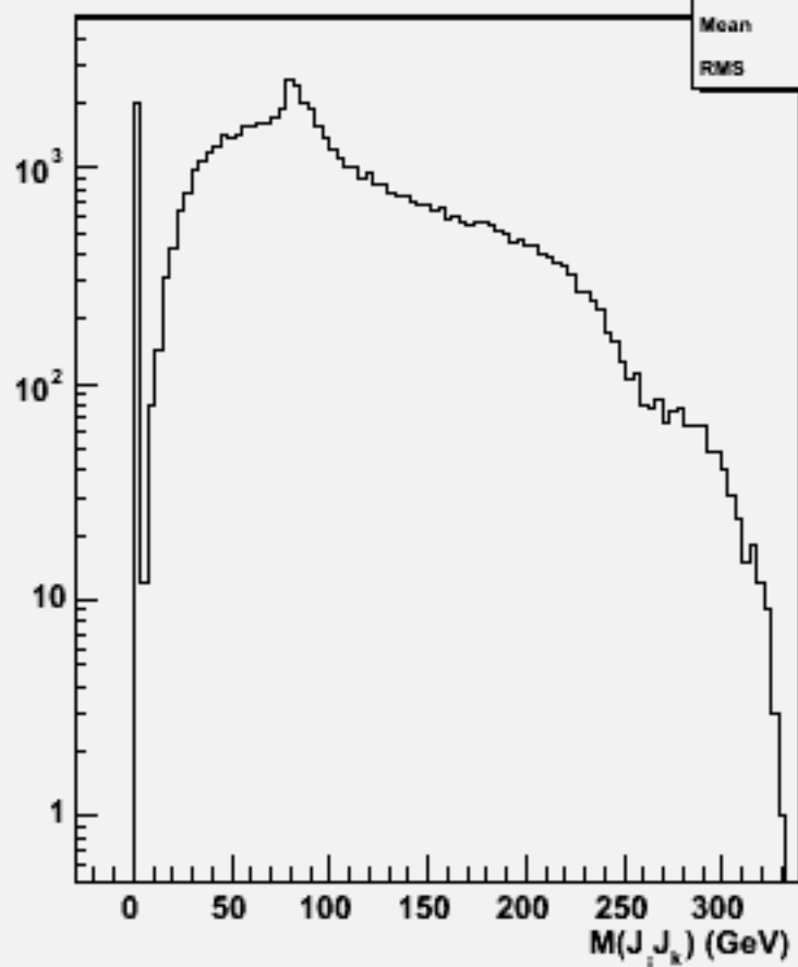
2jets mass(All comb)w103043 e1a_n1e1e1du_o
