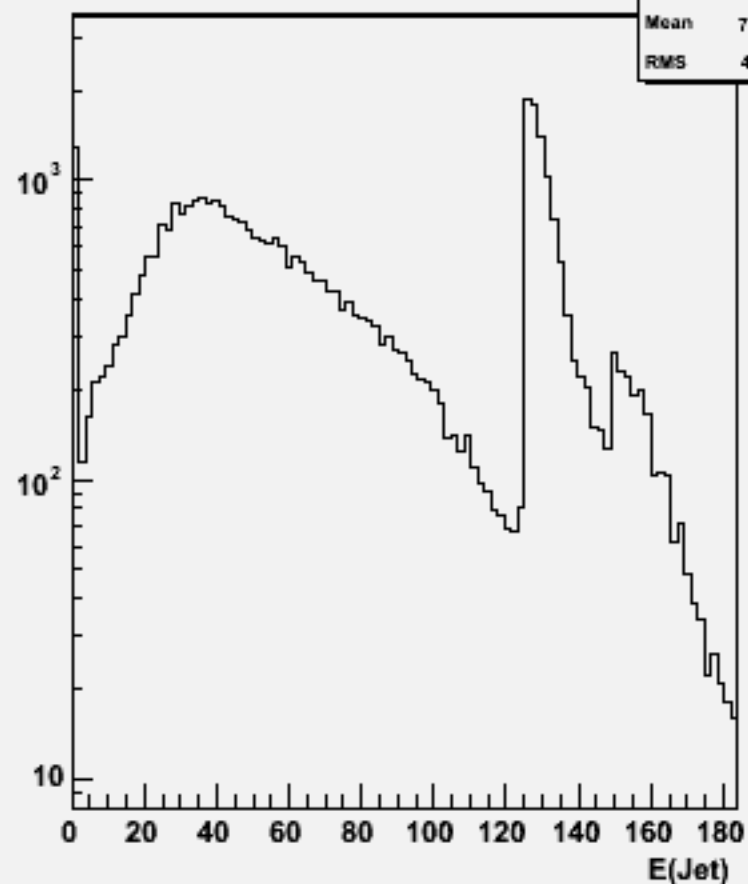
Jet energies(All jets)w103043 e1a_n1e1e1du_o
