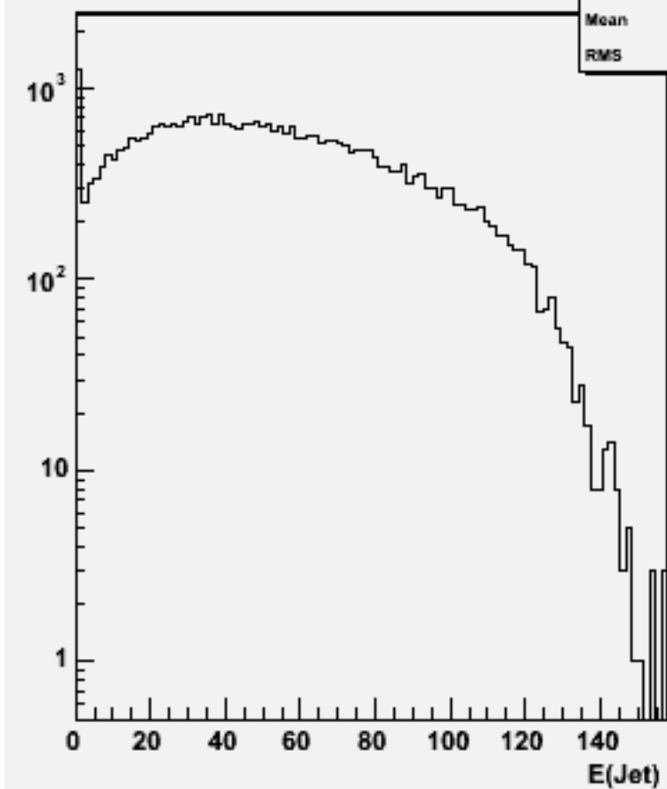
Jet energies(All jets)w103040 e1a_n1e1e1e3n3_o
