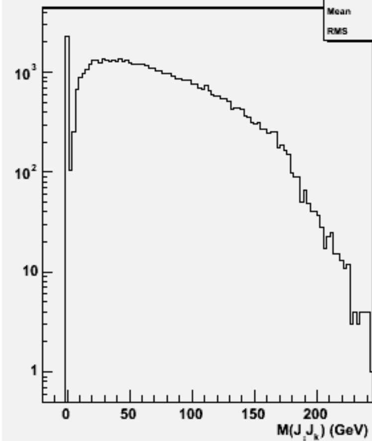
2jets mass(All comb)w103040 e1a_n1e1e1e3n3_o
