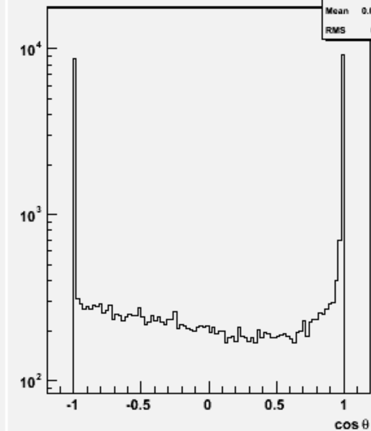
Jet cos \theta (All jets)w103040 e1a_n1e1e1e3n3_o
