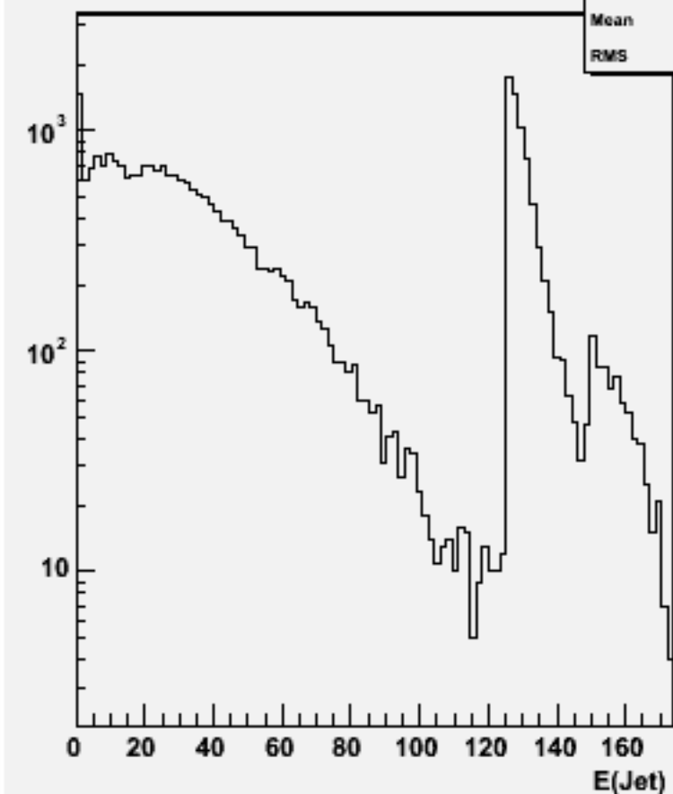
Jet energies(All jets)w103039 e1a_n1e1e1e3n3_o
