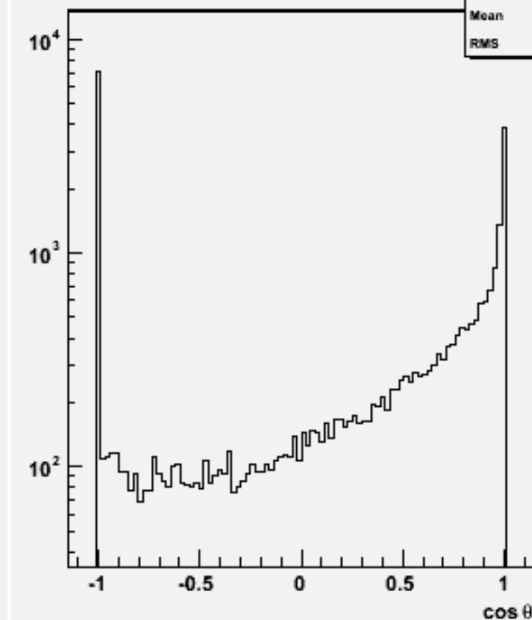
Jet cos \theta (All jets)w103039 e1a_n1e1e1e3n3_o
