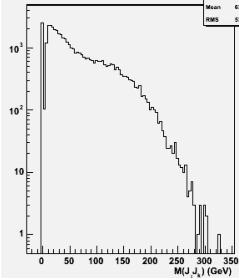
2jets mass(All comb)w103039 e1a_n1e1e1e3n3_o
