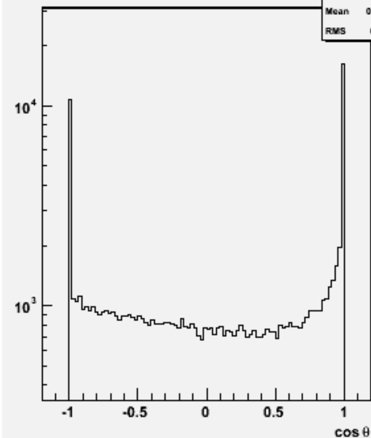
Particle cos \theta : w103038 e1a_n1e1e1e3n3_o
