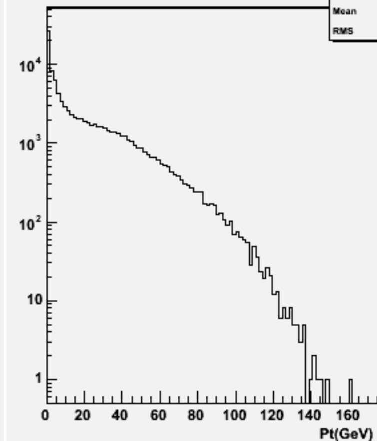
Particle Pt : w103038 e1a_n1e1e1e3n3_o
