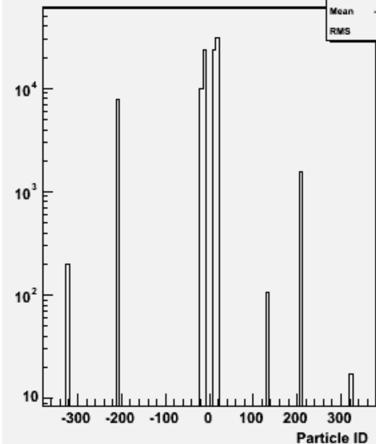
Particle ID : w103038 e1a_n1e1e1e3n3_o
