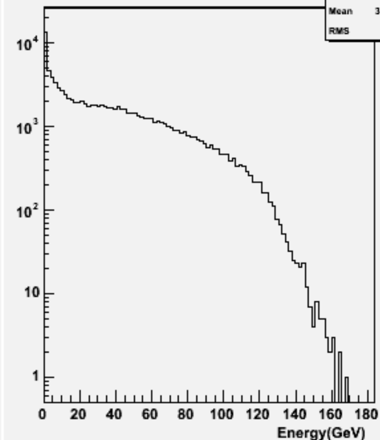
Particle Energy : w103038 e1a_n1e1e1e3n3_o
