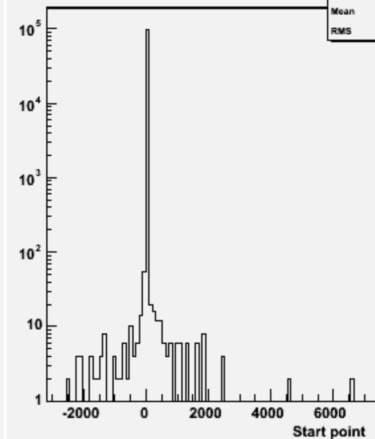
Start point Z : w103038 e1a_n1e1e1e3n3_o
