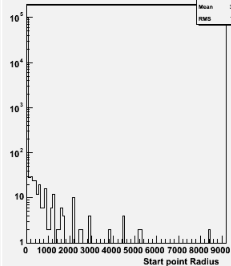
Start point R : w103038 e1a_n1e1e1e3n3_o
