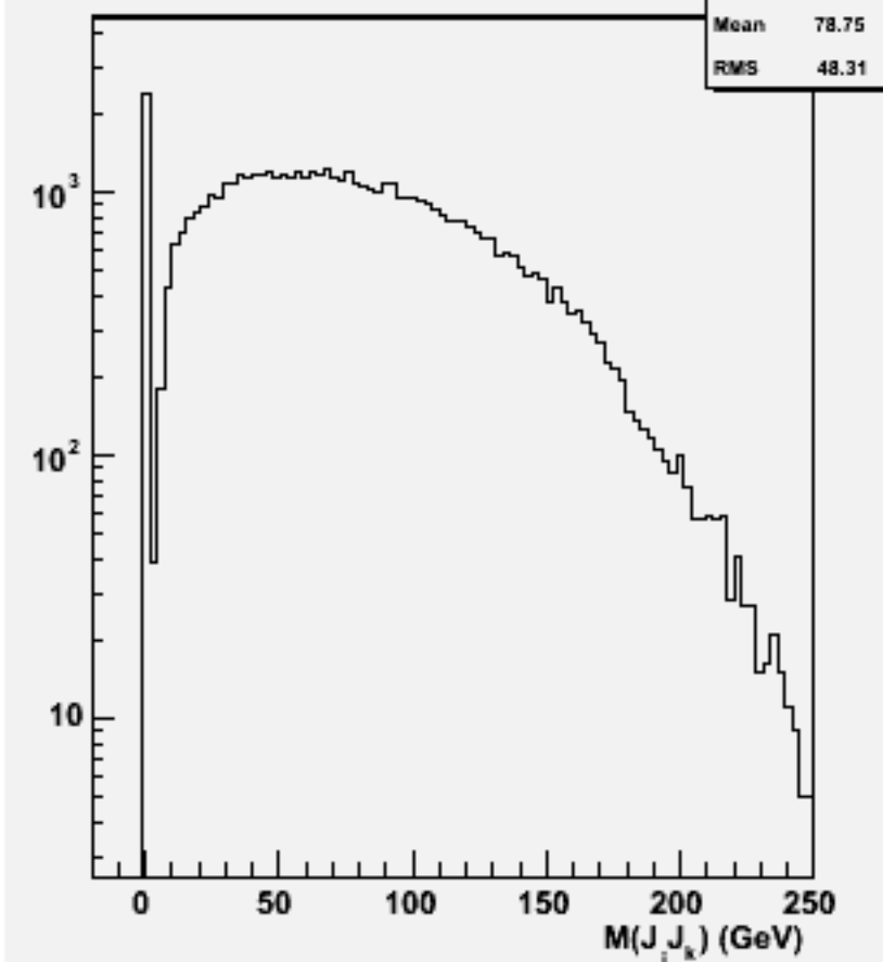
2jets mass(All comb)w103034 e1a_n1e1e1e2n2_o
