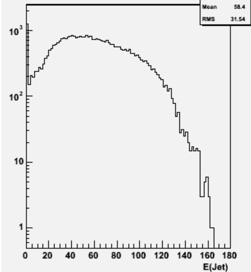
Jet energies(All jets)w103034 e1a_n1e1e1e2n2_o
