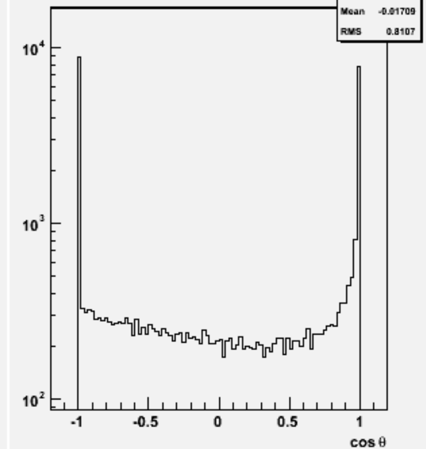
Jet cos \theta (All jets)w103034 e1a_n1e1e1e2n2_o
