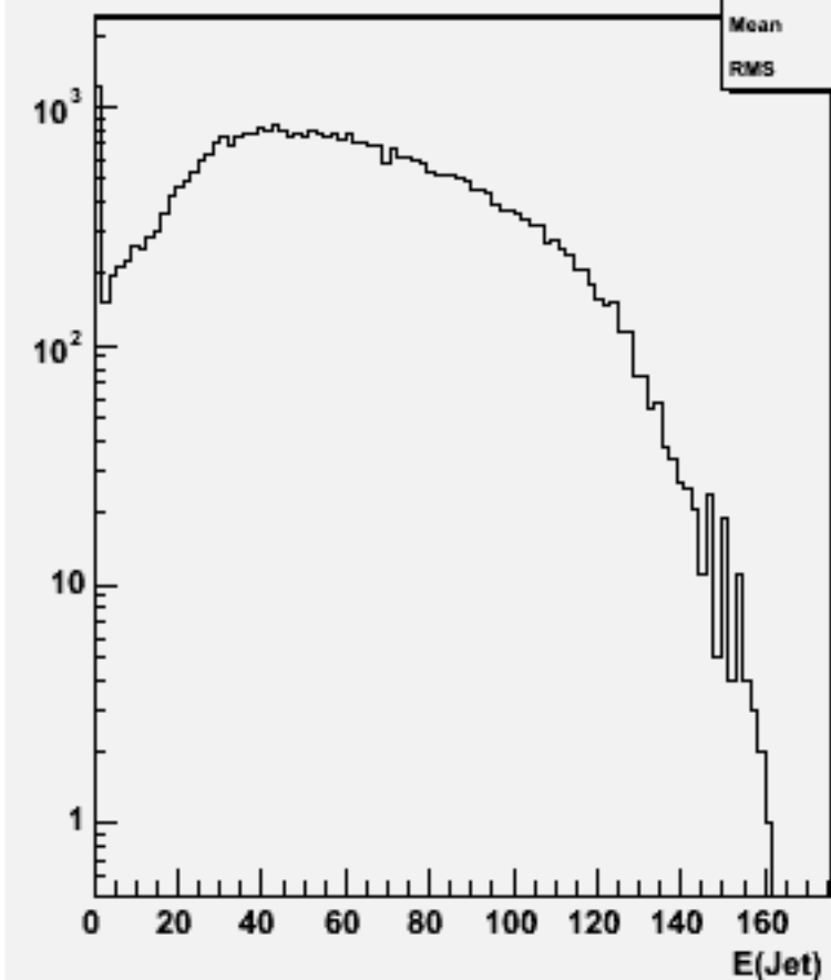
Jet energies(All jets)w103030 e1a_n1e1e1n1_o
