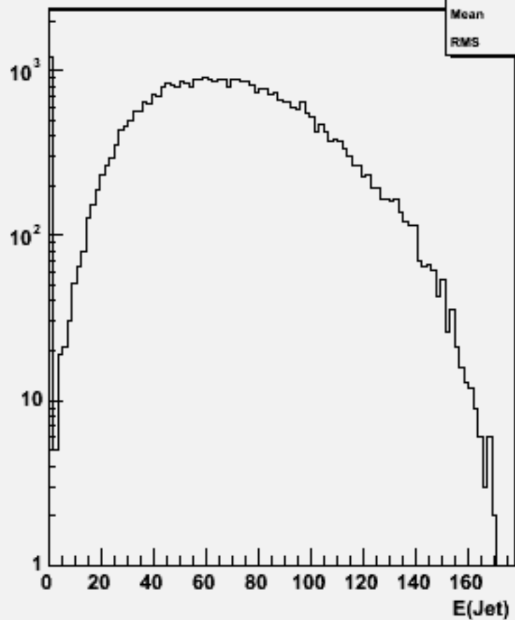
Jet energies(All jets)w103026 e1a_n1ccsc_o
