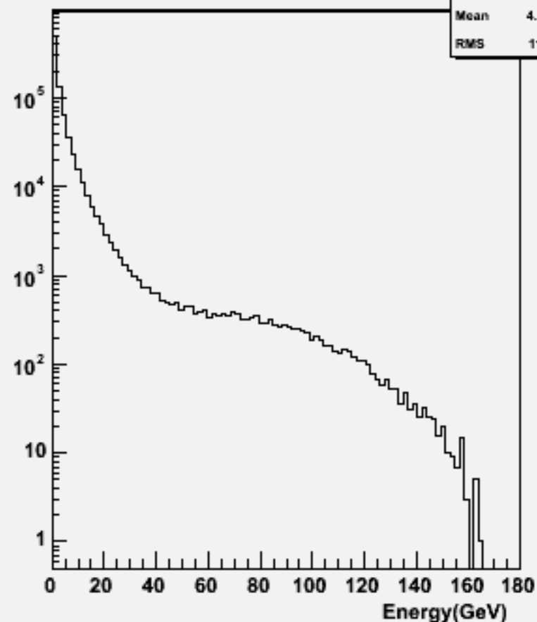
Particle Energy : w103022 e1a_n1ccdu_o
