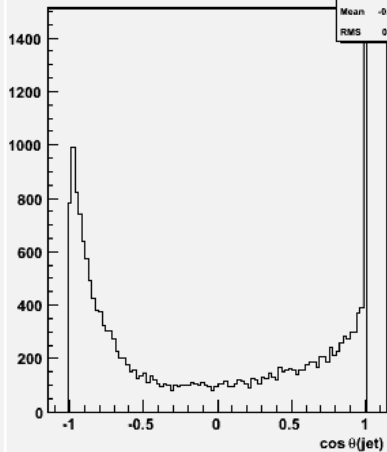
cos \Theta for 2-jets :w103022 e1a_n1ccdu_o
