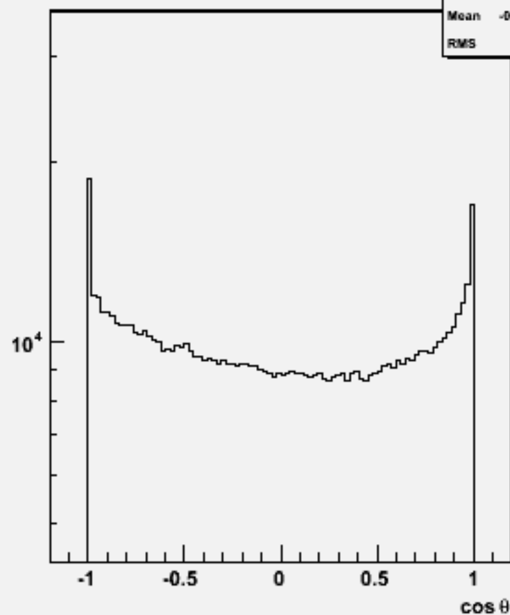
Particle cosθ : w103022 e1a_n1ccdu_o
