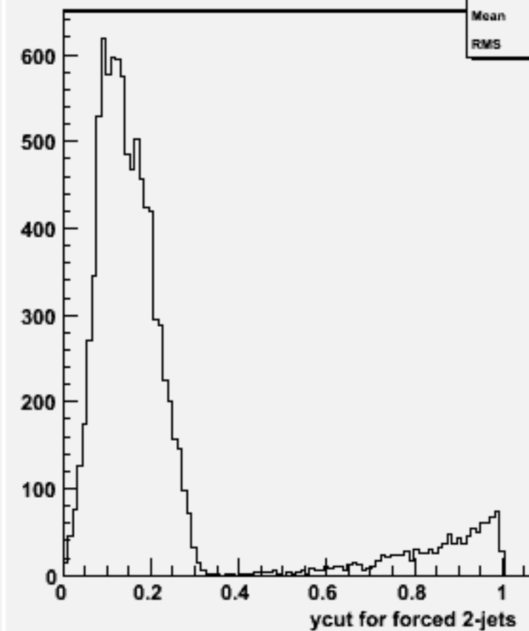
Ycut for 2-jets :w103022 e1a_n1ccdu_o
