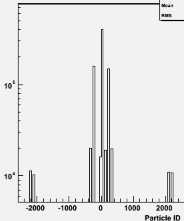
Particle ID : w103022 e1a_n1ccdu_o
