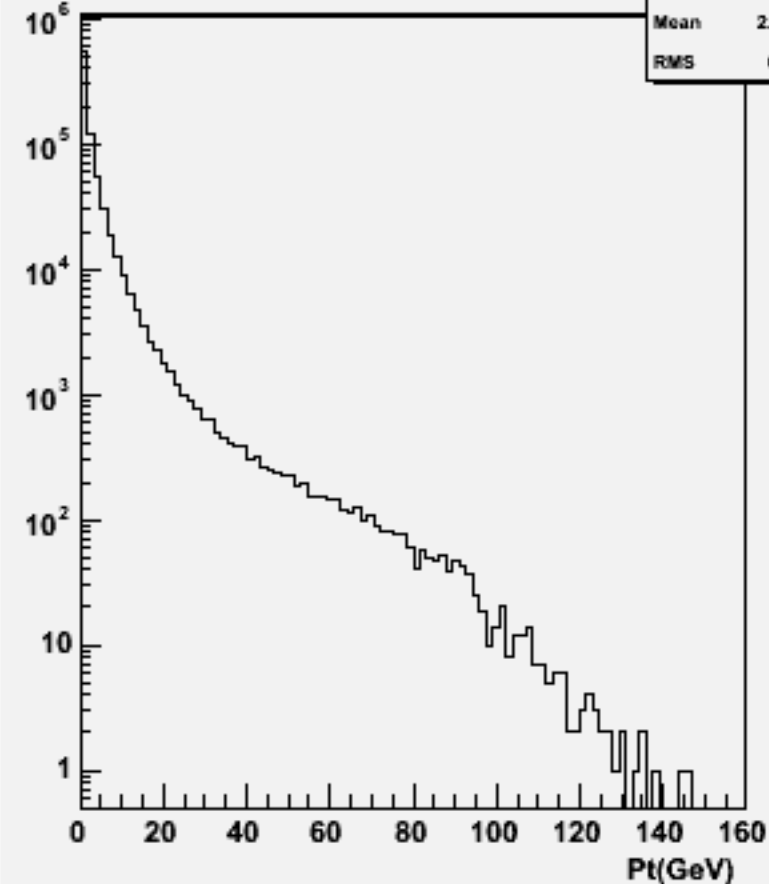
Particle Pt : w103022 e1a_n1ccdu_o
