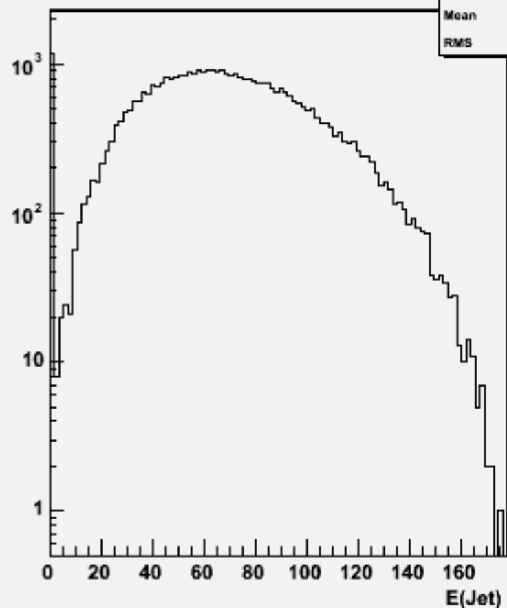
Jet energies(All jets)w103022 e1a_n1ccdu_o
