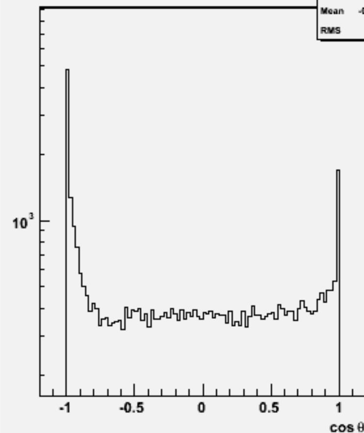
Jet cos \theta (All jets)w103022 e1a_n1ccdu_o
