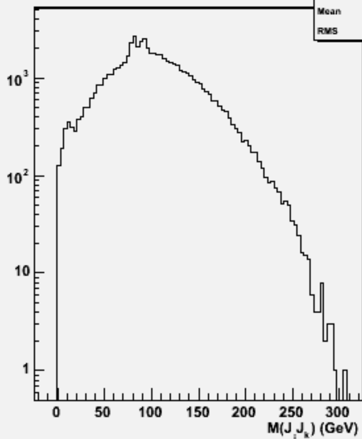
2jets mass(All comb)w103022 e1a_n1ccdu_o
