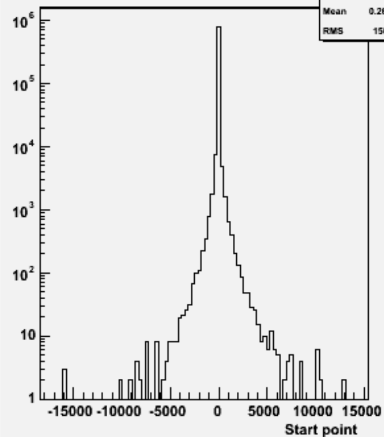
Start point Z : w103022 e1a_n1ccdu_o
