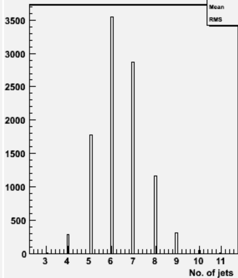
No. jets (ycut=0.001) : w103022 e1a_n1ccdu_o
