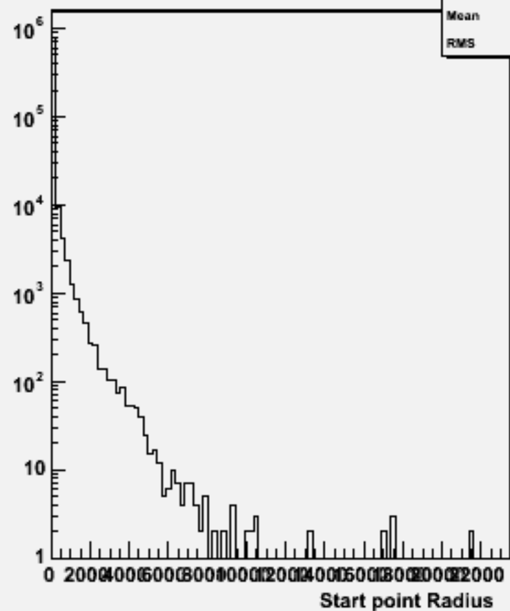
Start point R : w103022 e1a_n1ccdu_o
