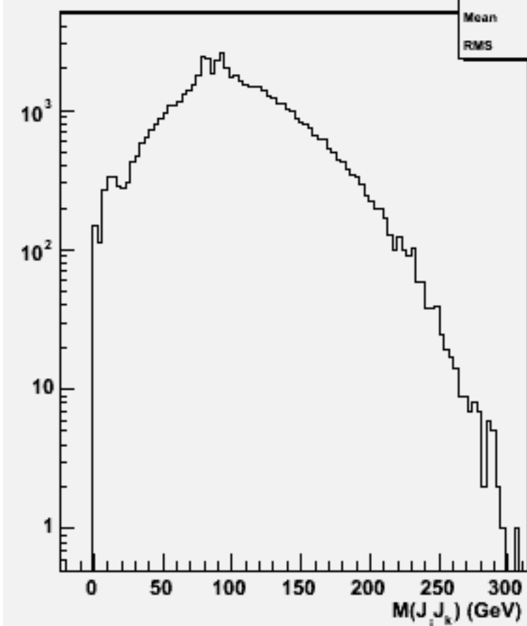
2jets mass(All comb)w103006 e1a_n1uusc_o
