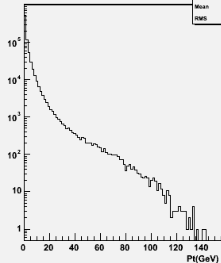
Particle Pt : w103006 e1a_n1uusc_o
