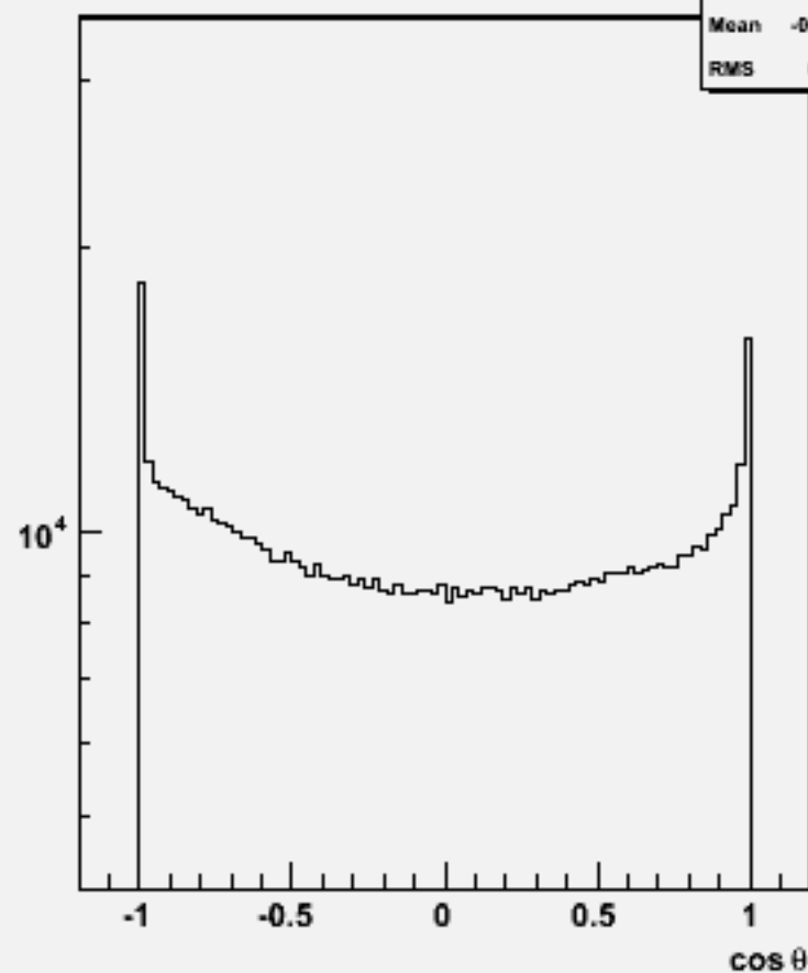
Particle cosθ : w103006 e1a_n1uusc_o
