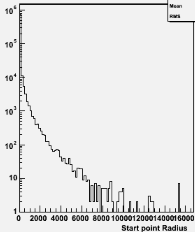
Start point R : w103006 e1a_n1uusc_o
