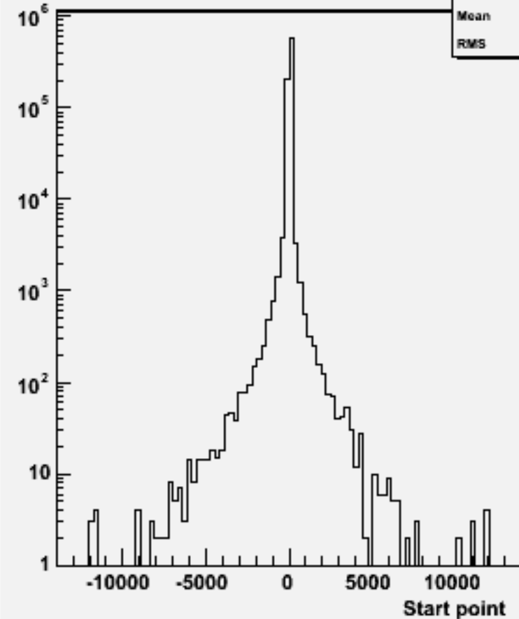
Start point Z : w103006 e1a_n1uusc_o
