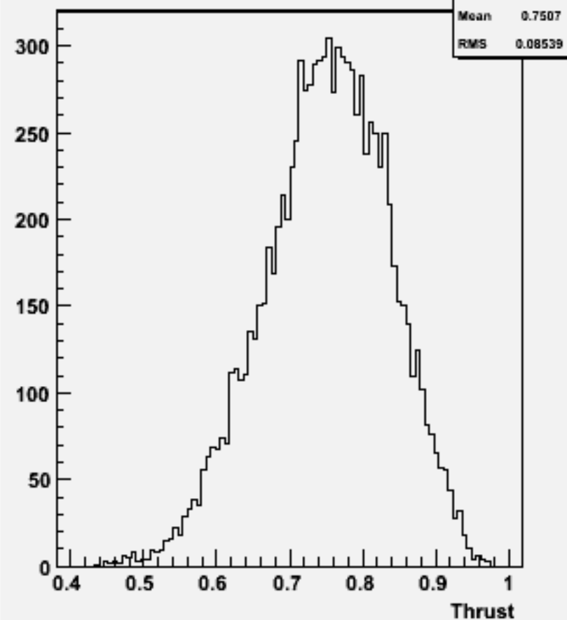
Thrust w103006 e1a_n1uusc_o
