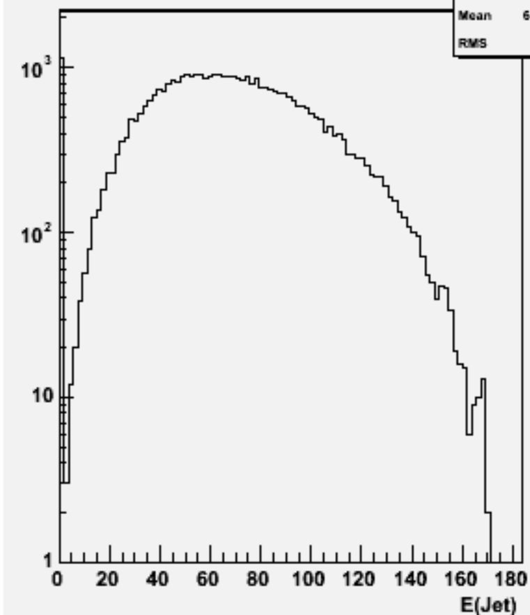
Jet energies(All jets)w103006 e1a_n1uusc_o
