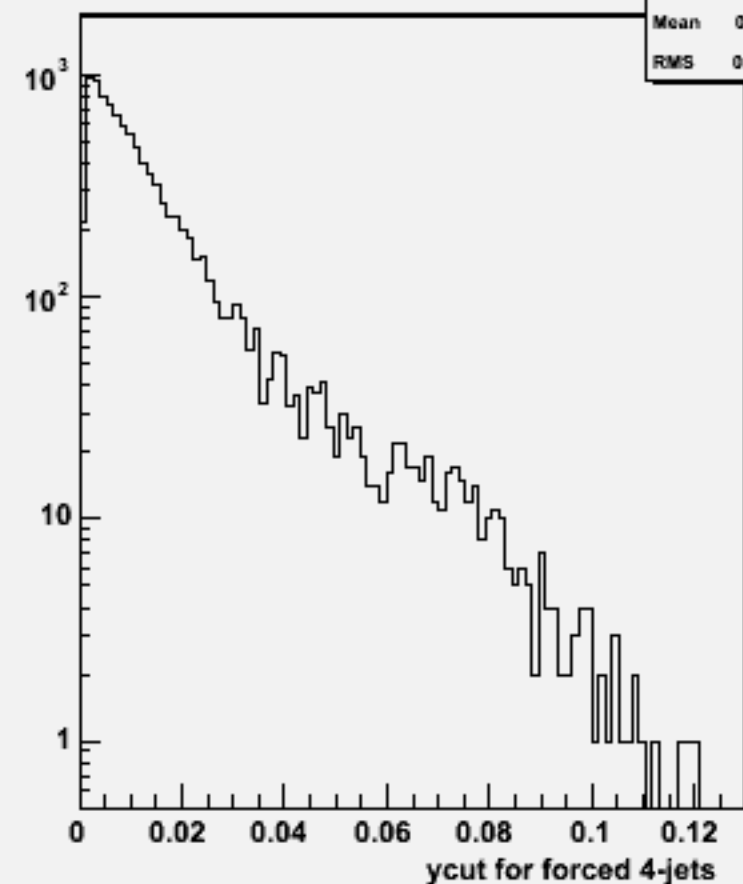
Ycut for 4-jets :w103006 e1a_n1uusc_o
