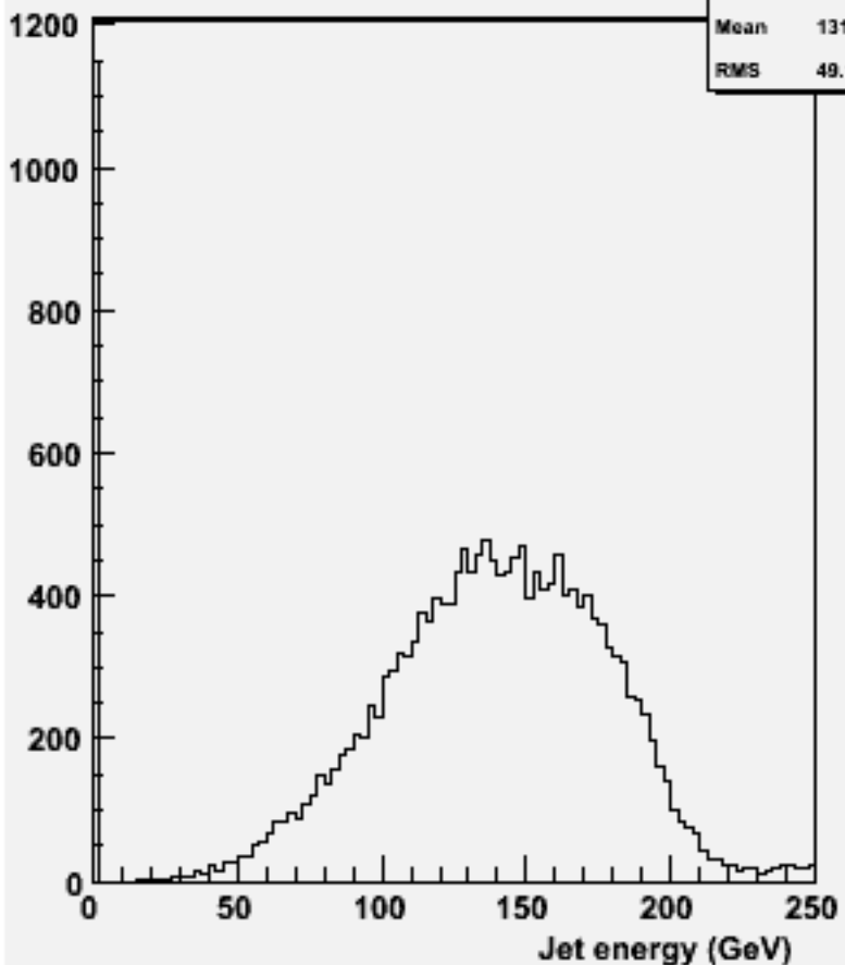
energy for 2-jets :w103006 e1a_n1uusc_o
