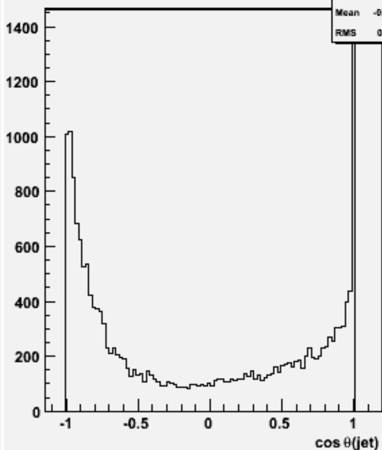
cos \theta for 2-jets :w103006 e1a_n1uusc_o
