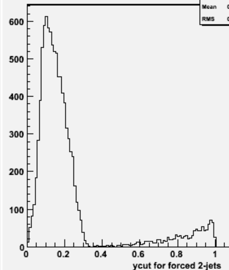
Ycut for 2-jets :w103006 e1a_n1uusc_o
