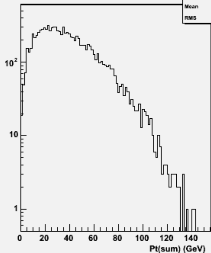
Pt Sum: w103006 e1a_n1uusc_o
