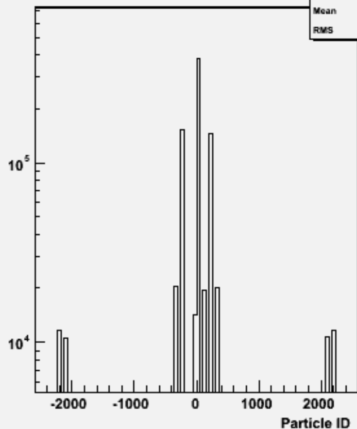
Particle ID : w103006 e1a_n1uusc_o
