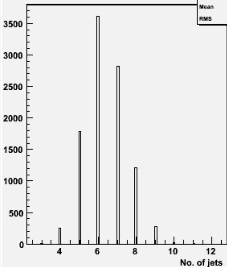
No. jets (ycut=0.001) : w103006 e1a_n1uusc_o
