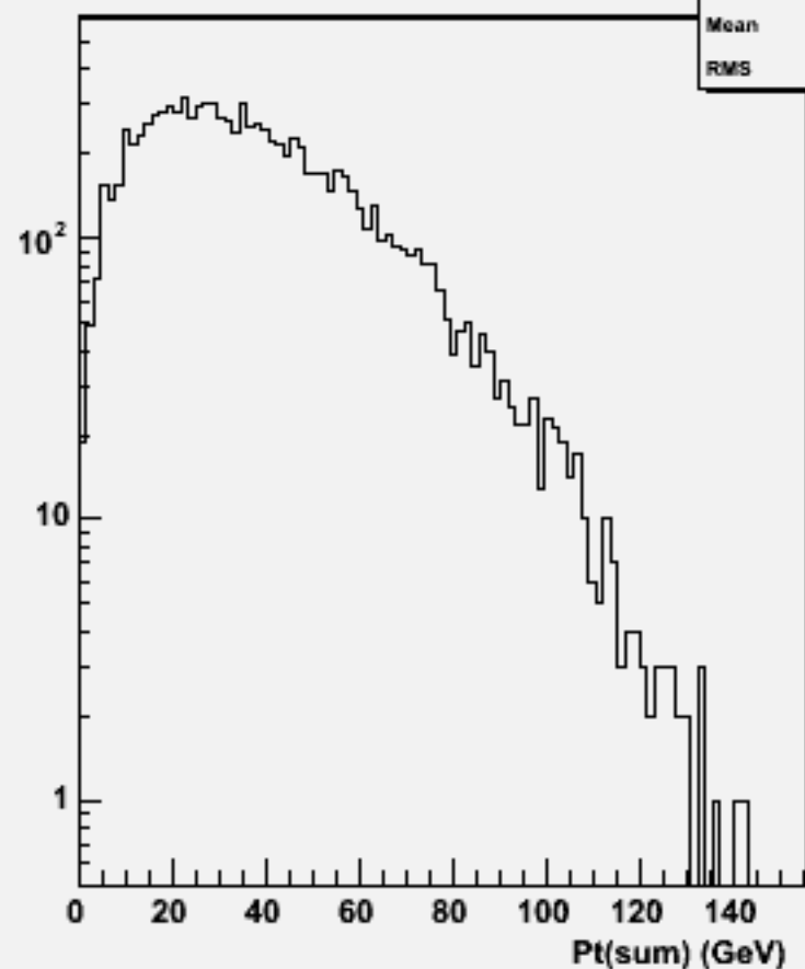
Pt Sum: w103006 e1a_n1uusc_o
