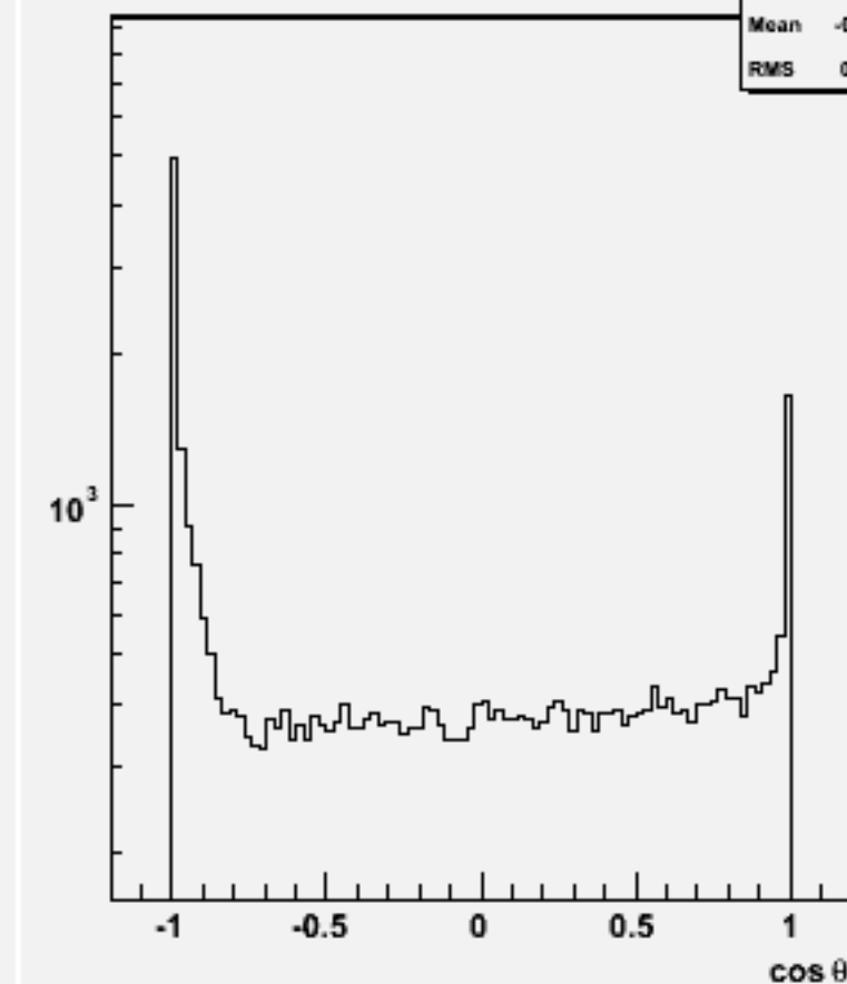
Jet cos \theta (All jets)w103006 e1a_n1uusc_o
