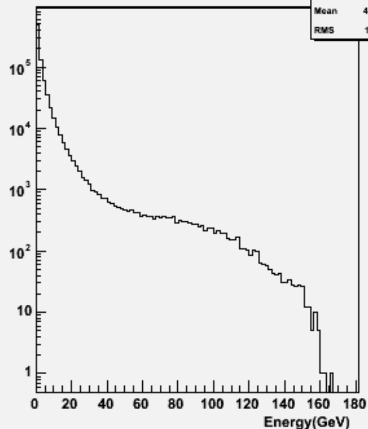
Particle Energy : w103006 e1a_n1uusc_o
