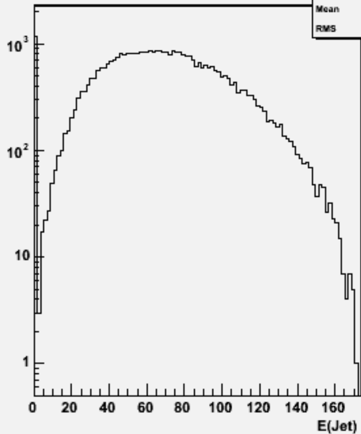
Jet energies(All jets)w103002 e1a_n1uu1du_o
