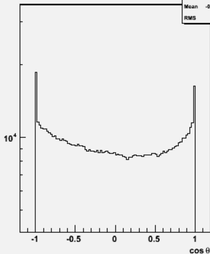
Particle cos \theta : w103002 e1a_n1uu1du_o
