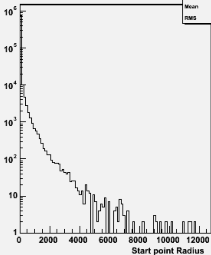
Start point R : w103002 e1a_n1uu1du_o
