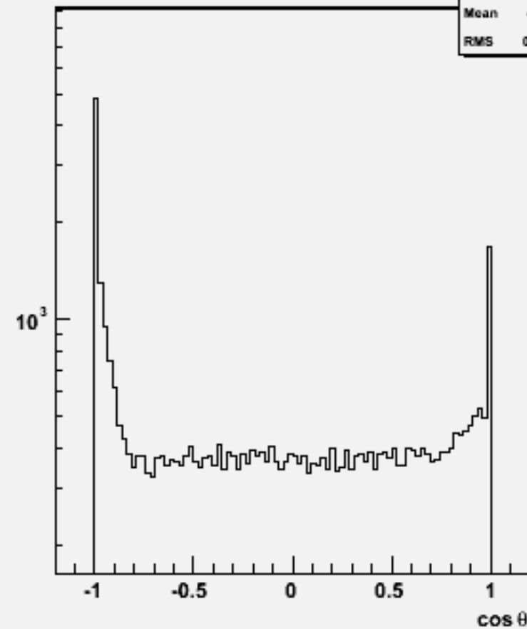
Jet cosθ (All jets)w103002 e1a_n1uu1du_o
