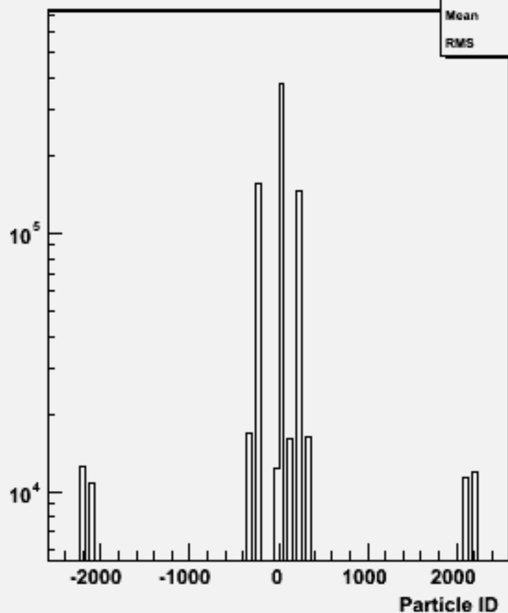
Particle ID : w103002 e1a_n1uu1du_o
