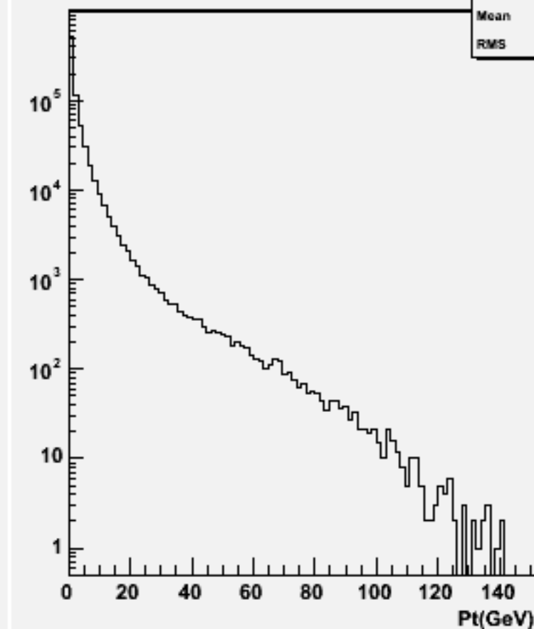
Particle Pt : w103002 e1a_n1uu1du_o
