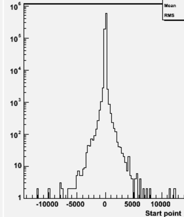
Start point Z : w103002 e1a_n1uu1du_o
