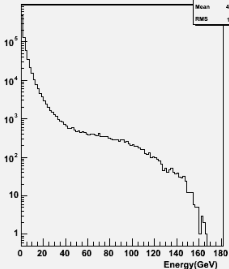
Particle Energy : w103002 e1a_n1uu1du_o
