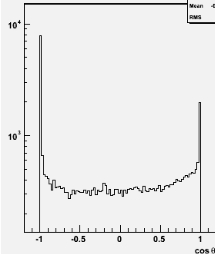
Jet cos \theta (All jets)w102998 e1a_n1uue3n3_o
