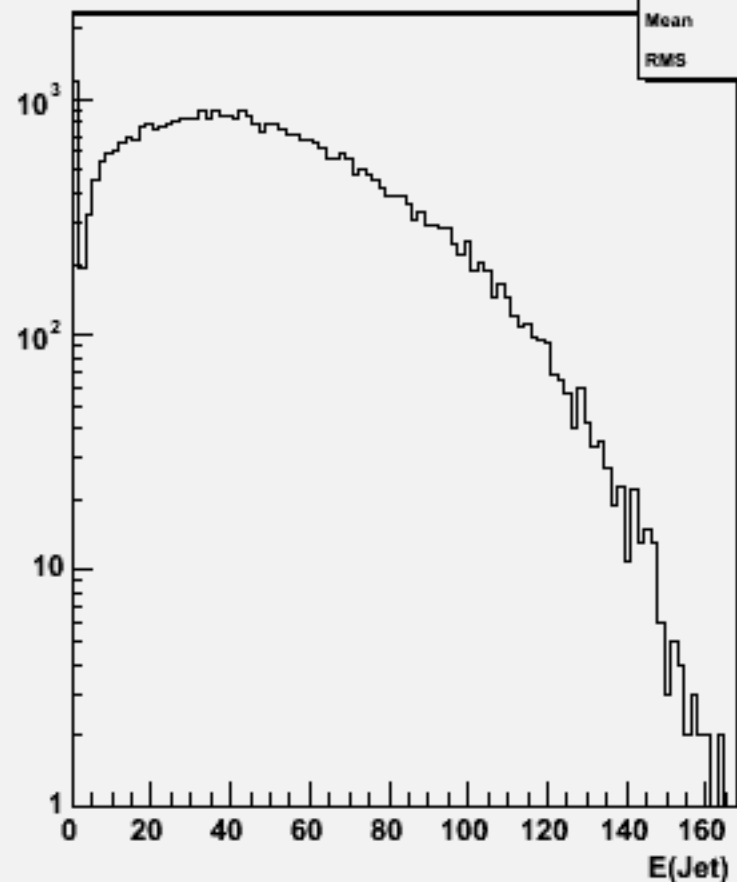
Jet energies(All jets)w102998 e1a_n1uue3n3_o
