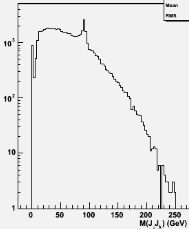
2jets mass(All comb)w102998 e1a_n1uue3n3_o
