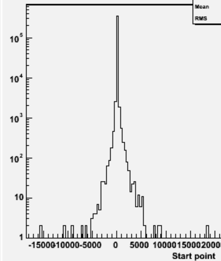
Start point Z : w102992 e1a_n1uue1n1_o
