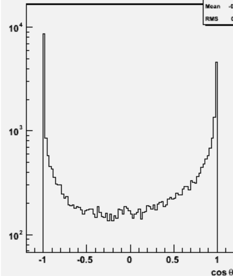
Jet cos \theta (All jets)w102992 e1a_n1uue1n1_o
