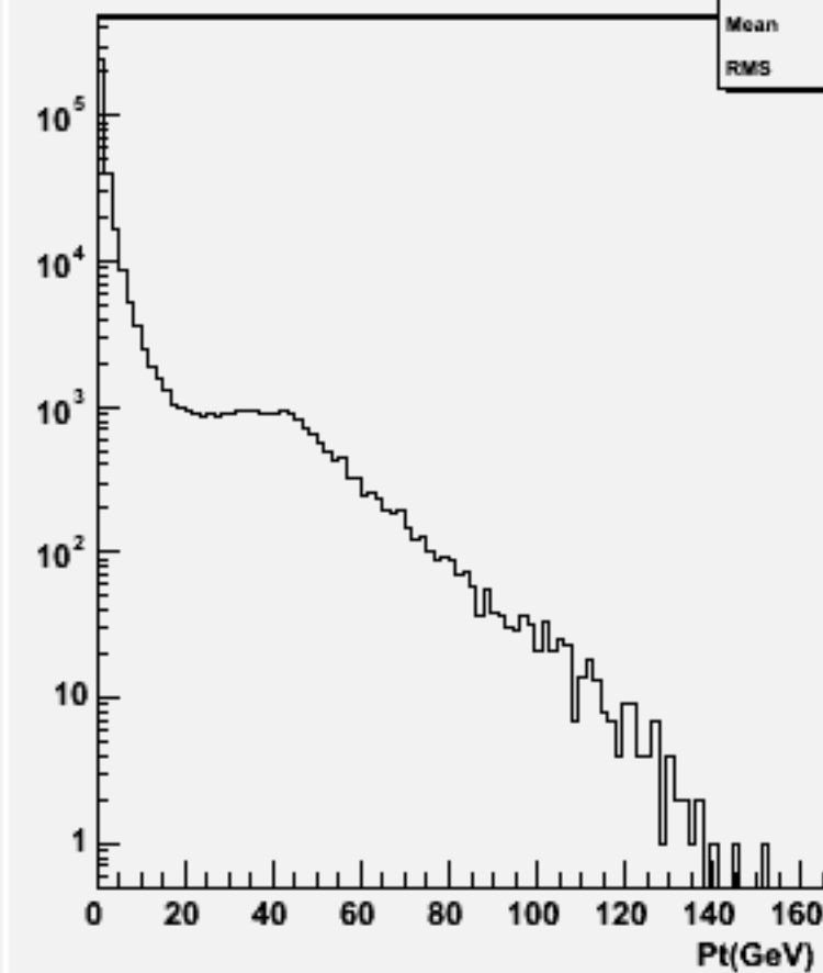
Particle Pt : w102992 e1a_n1uue1n1_o
