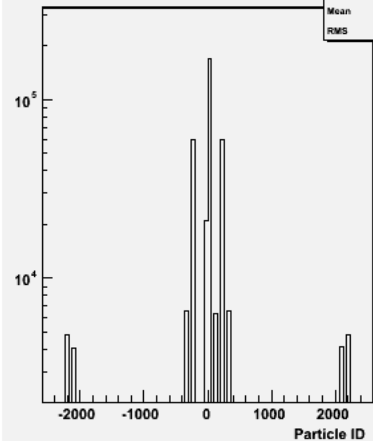
Particle ID : w102992 e1a_n1uue1n1_o
