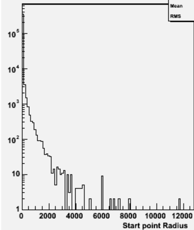
Start point R : w102992 e1a_n1uue1n1_o
