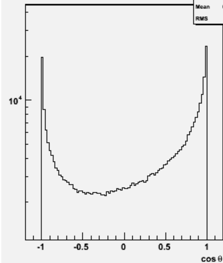
Particle cos \theta : w102992 e1a_n1uue1n1_o
