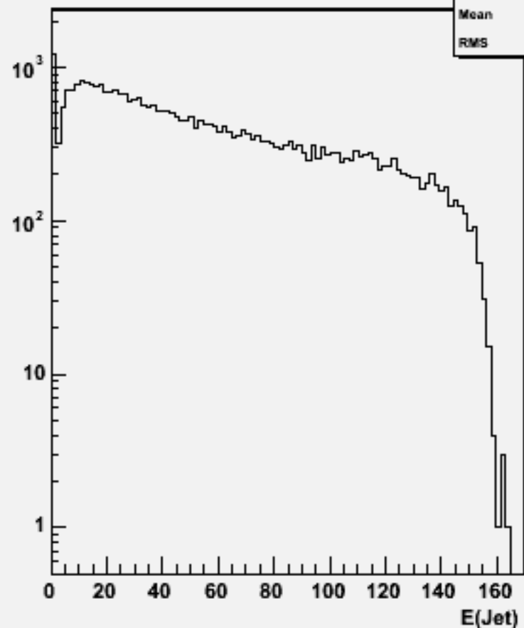
Jet energies(All jets)w102992 e1a_n1uue1n1_o
