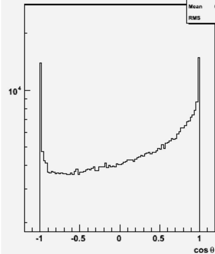
Particle cos \theta : w102990 e1a_n1uue1n1_o
