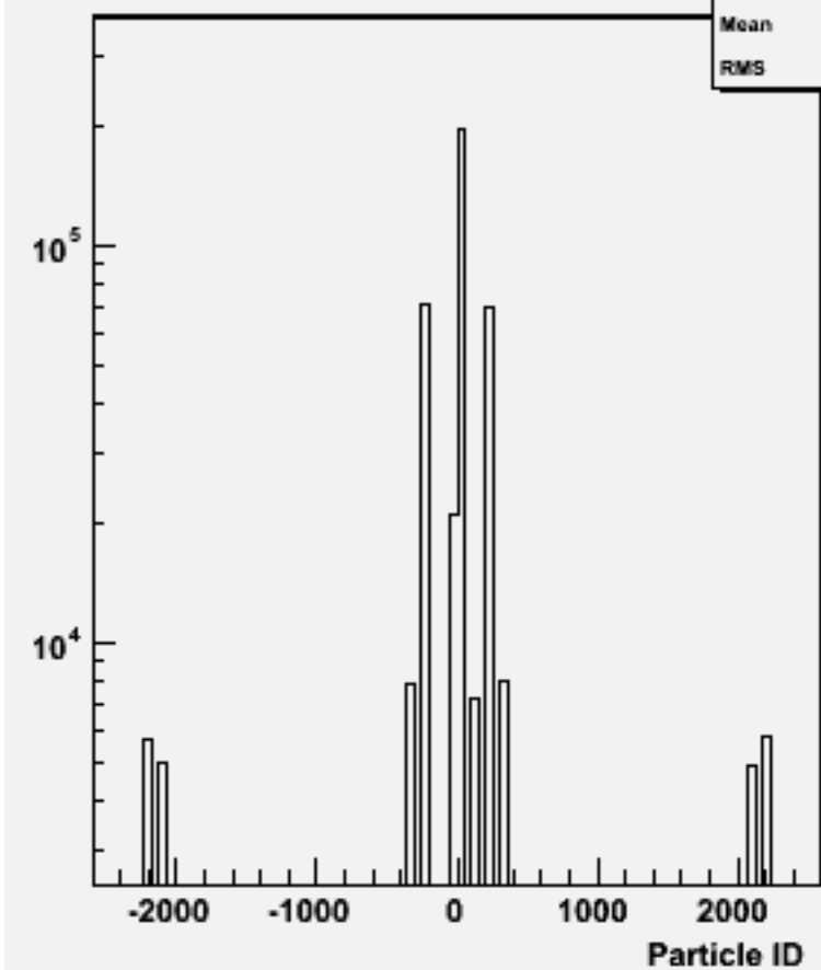
Particle ID : w102990 e1a_n1uue1n1_o
