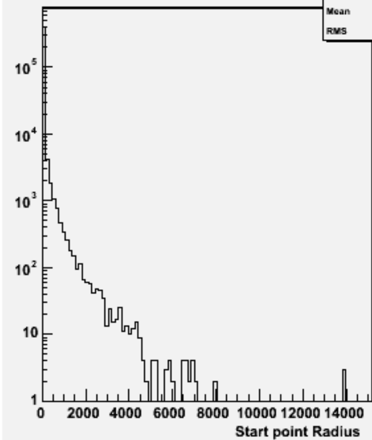
Start point R : w102990 e1a_n1uue1n1_o
