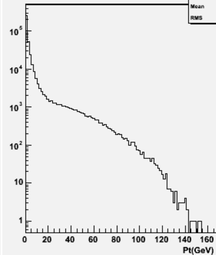
Particle Pt : w102990 e1a_n1uue1n1_o
