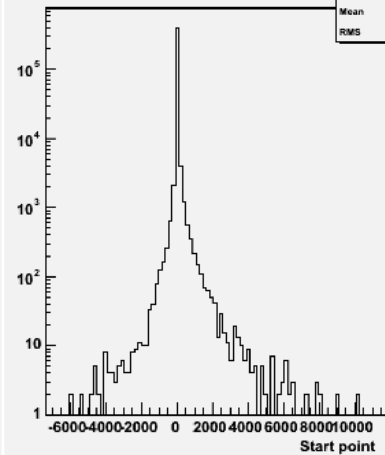
Start point Z : w102990 e1a_n1uue1n1_o
