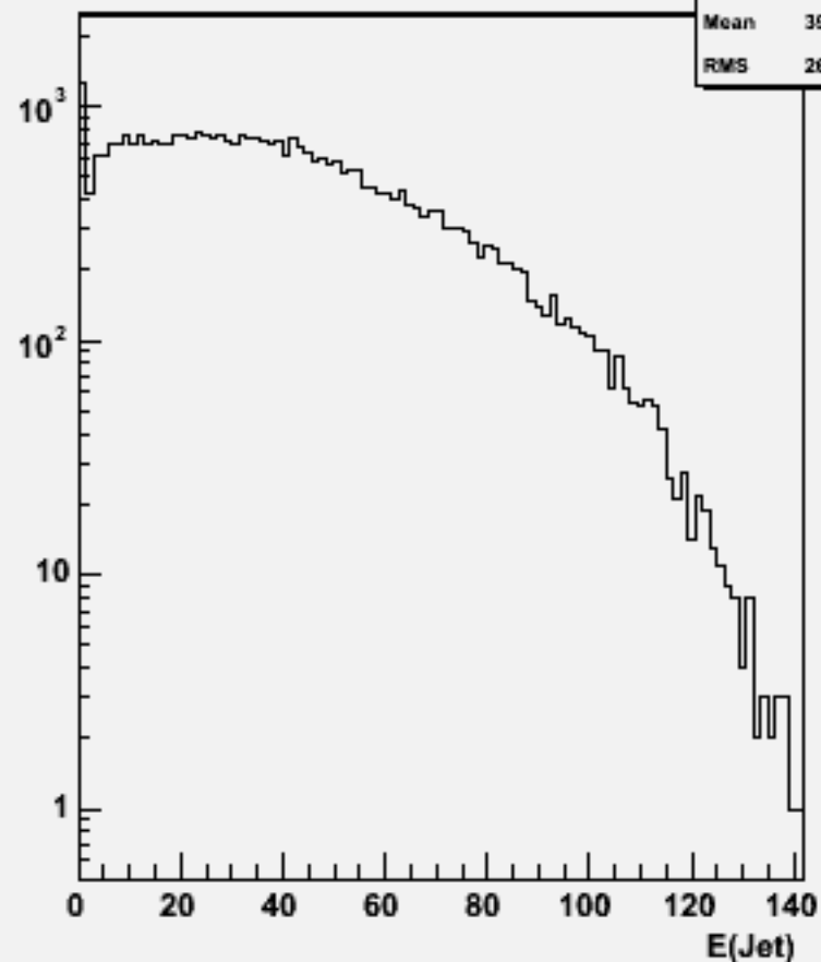
Jet energies(All jets)w102986 e1a_n1n3n3sc_o
