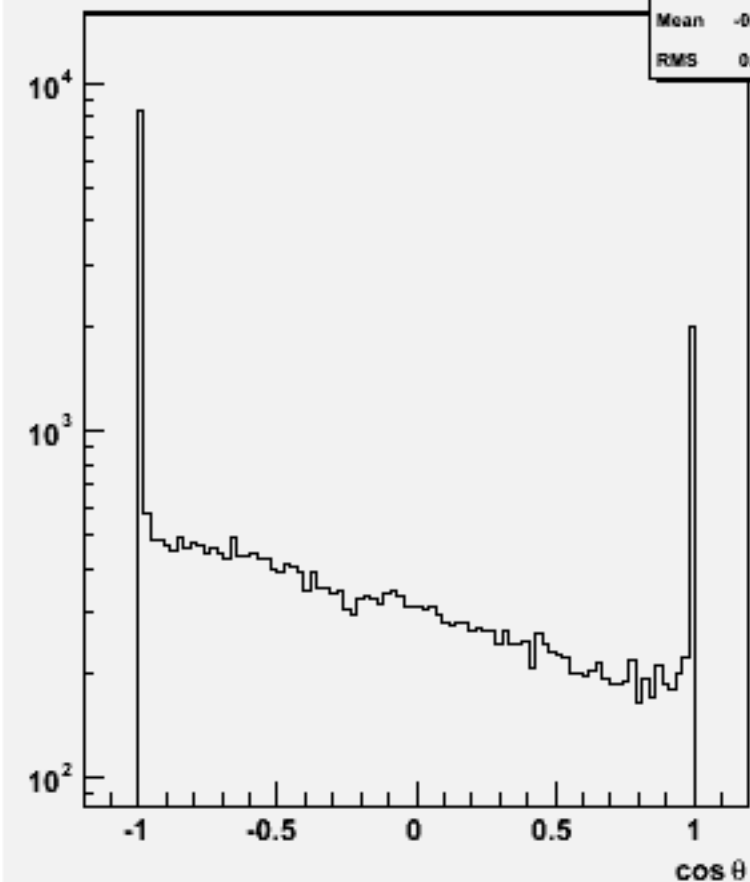
Jet cos \theta (All jets)w102986 e1a_n1n3n3sc_o
