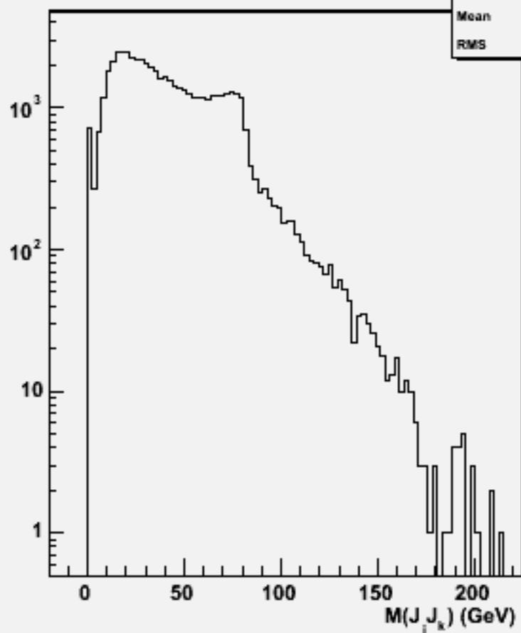
2jets mass(All comb)w102986 e1a_n1n3n3sc_o
