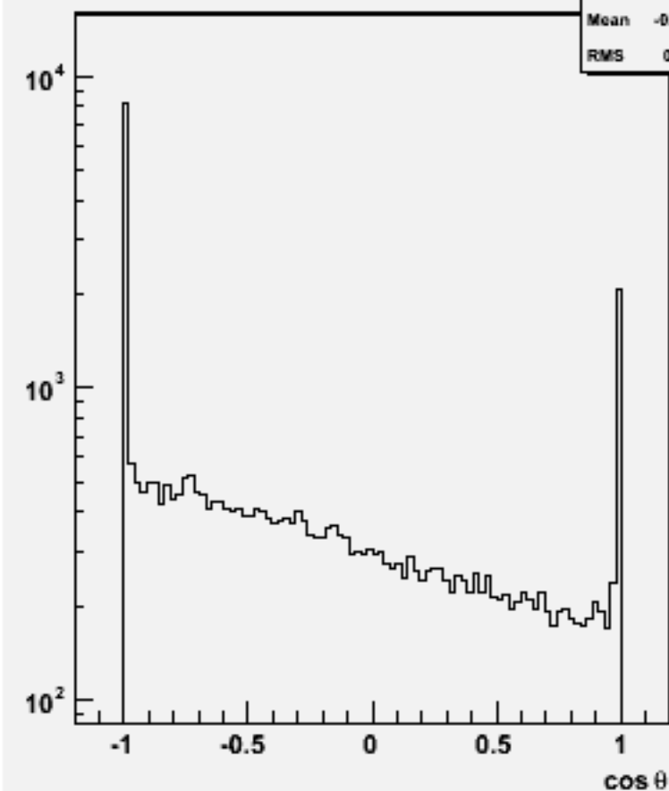
Jet cos \theta (All jets)w102982 e1a_n1n3n3du_o
