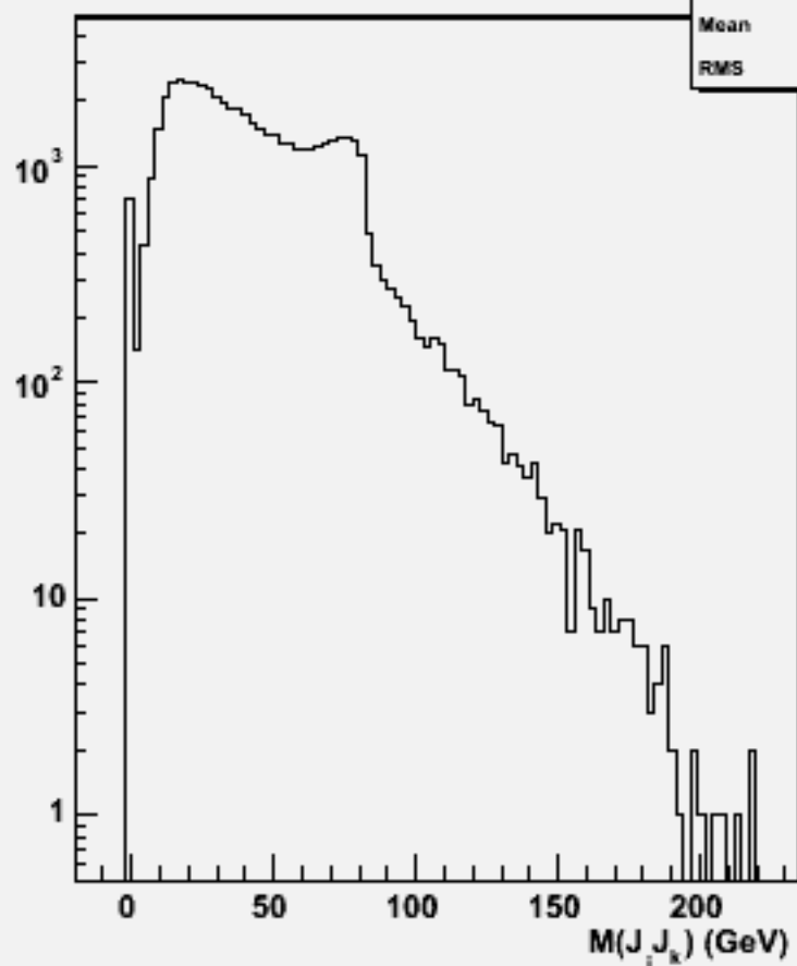
2jets mass(All comb)w102982 e1a_n1n3n3du_o
