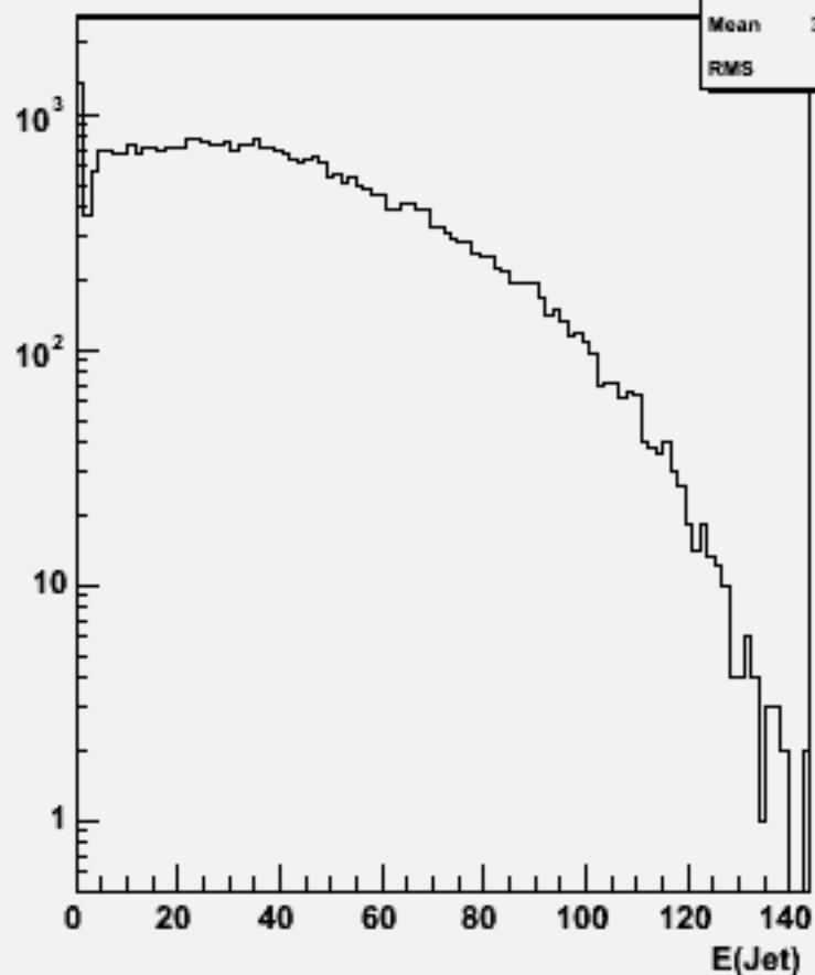
Jet energies(All jets)w102982 e1a_n1n3n3du_o
