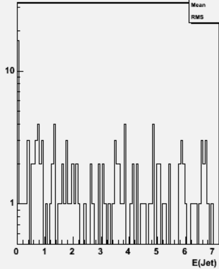
Jet energies(All jets)w102978 e1a_n1n3n3e3n3_o
