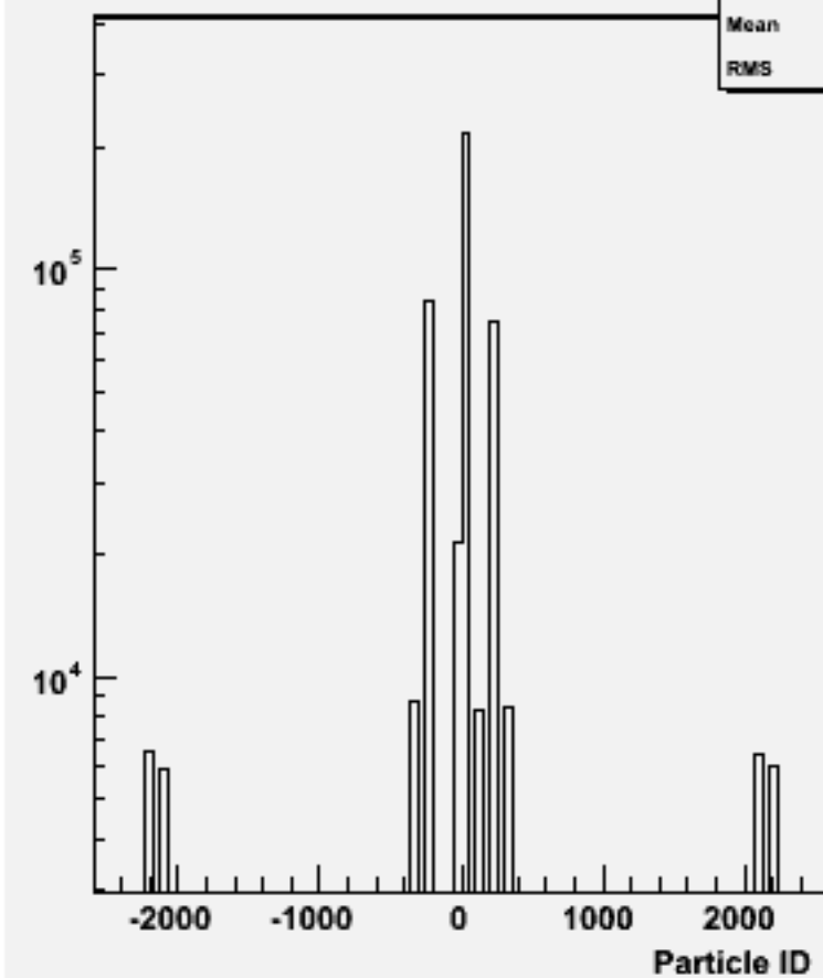
Particle ID : w102942 e1a_n1n1n1du_o
