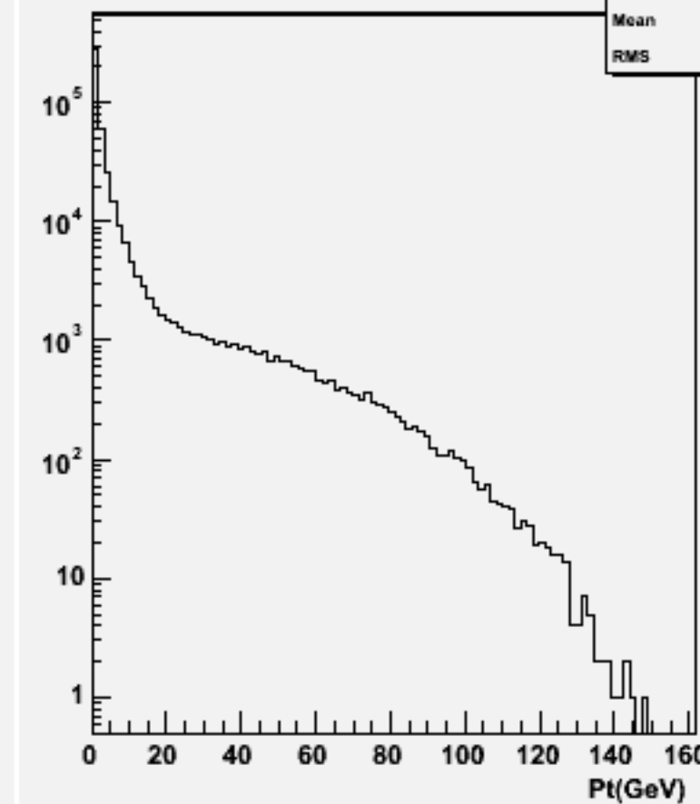
Particle Pt : w102942 e1a_n1n1n1du_o
