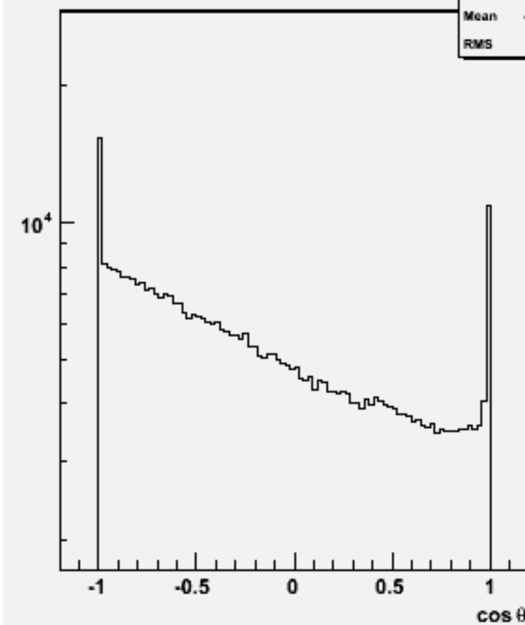
Particle cos \theta : w102942 e1a_n1n1n1du_o
