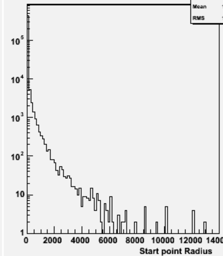
Start point R : w102942 e1a_n1n1n1du_o
