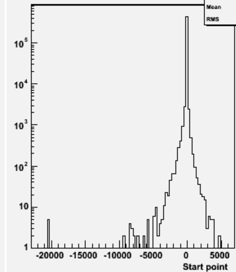
Start point Z : w102942 e1a_n1n1n1du_o
