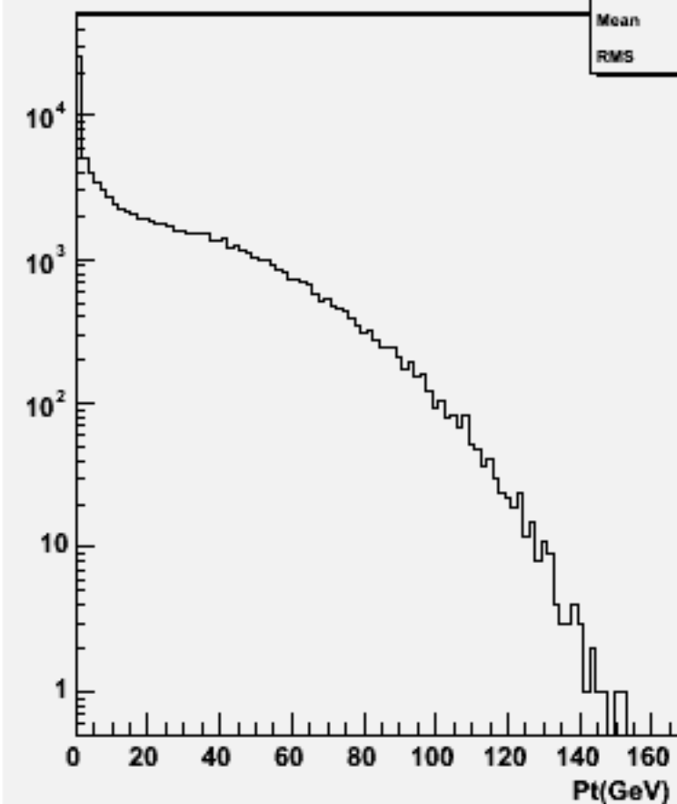
Particle Pt : w102938 e1a_n1n1n1e3n3_o
