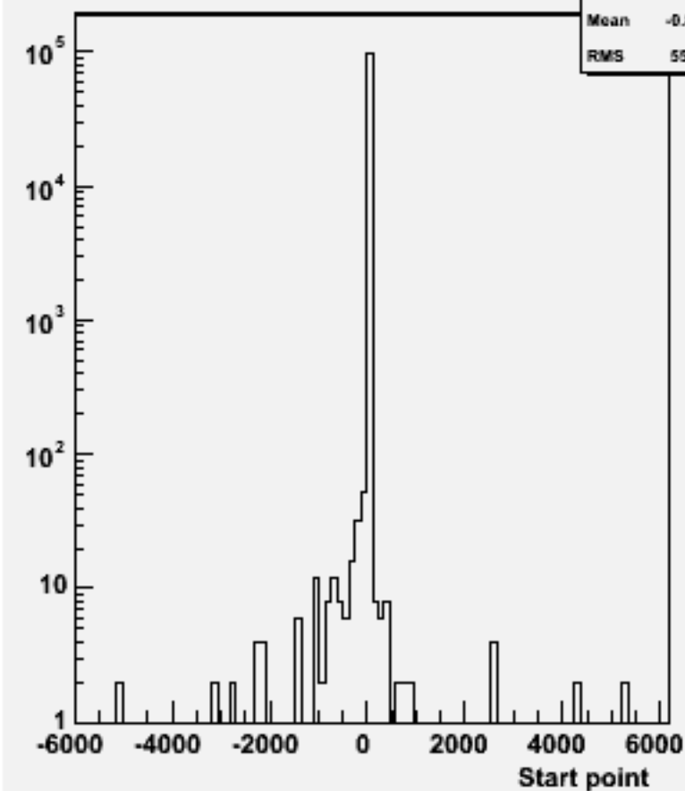
Start point Z : w102938 e1a_n1n1n1e3n3_o
