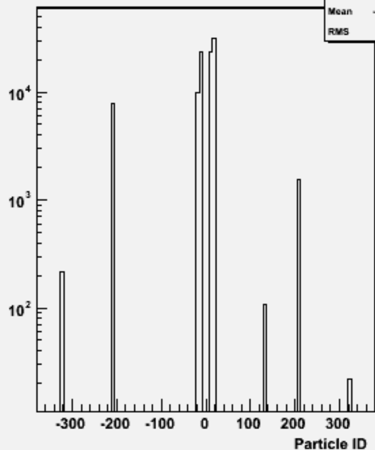
Particle ID : w102938 e1a_n1n1n1e3n3_o
