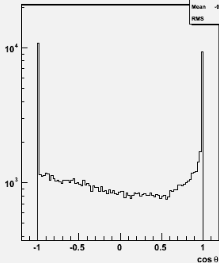
Particle cos \theta : w102938 e1a_n1n1n1e3n3_o
