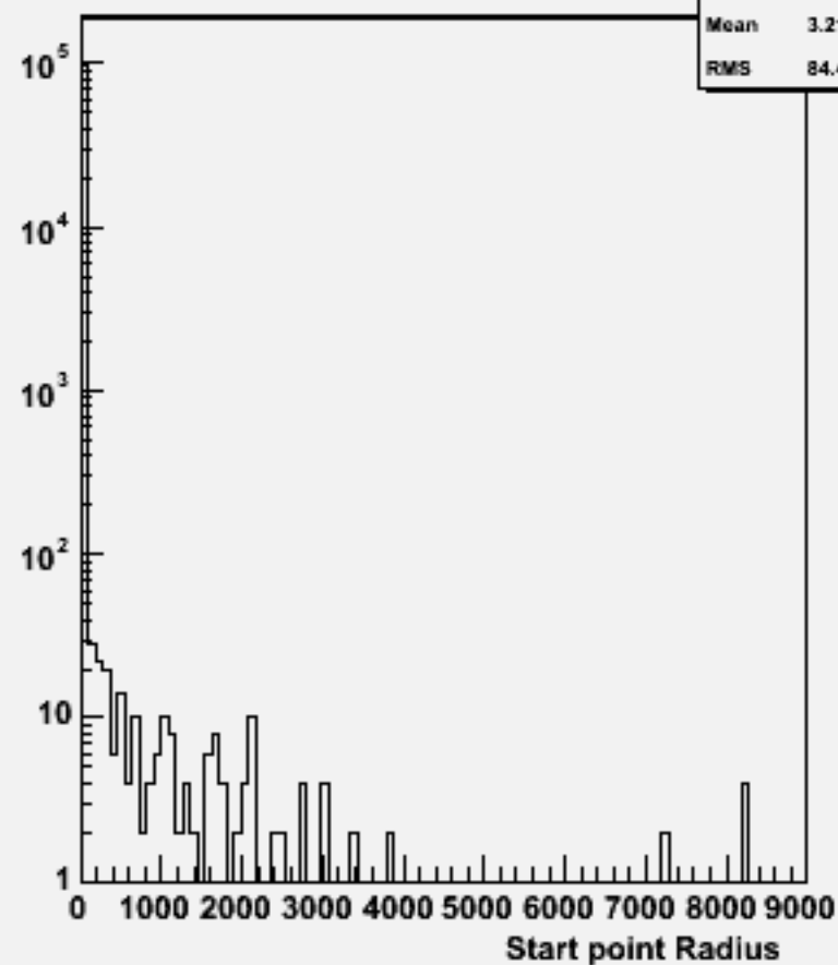
Start point R : w102938 e1a_n1n1n1e3n3_o
