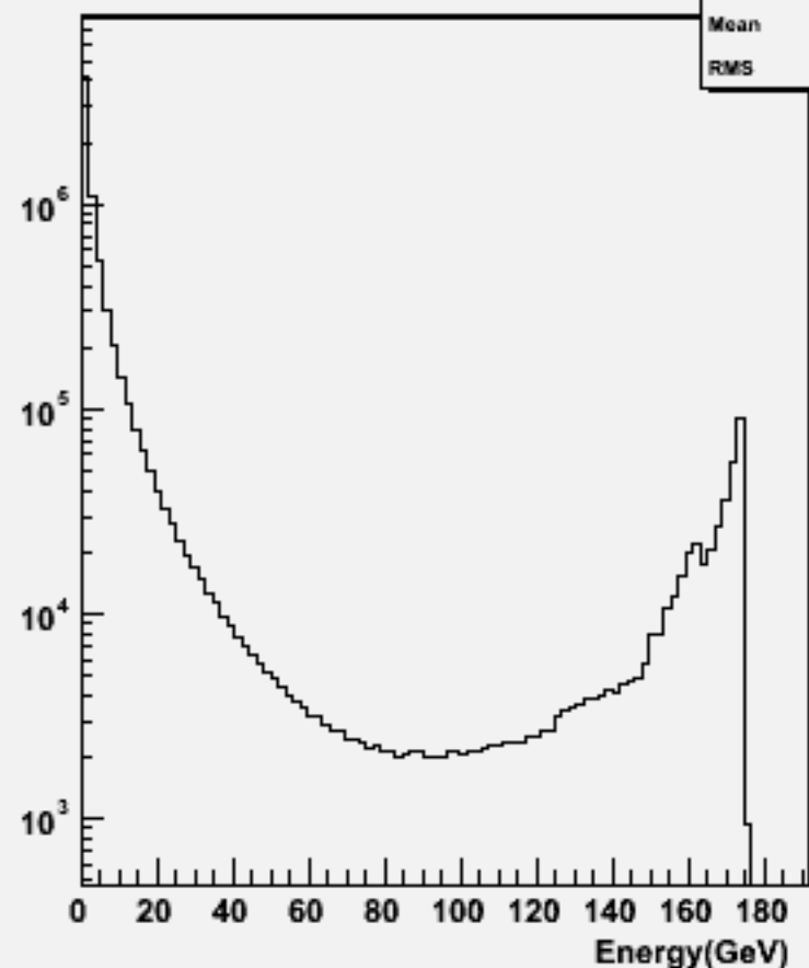
Particle Energy : w102855 e1a_e1dd_o
