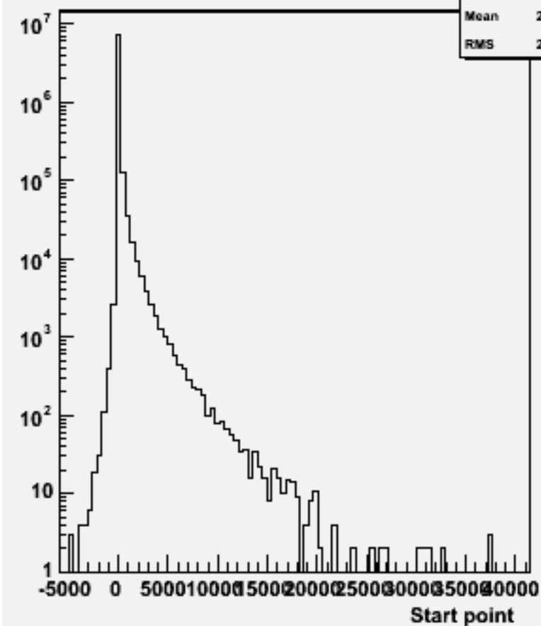
Start point Z : w102855 e1a_e1dd_o
