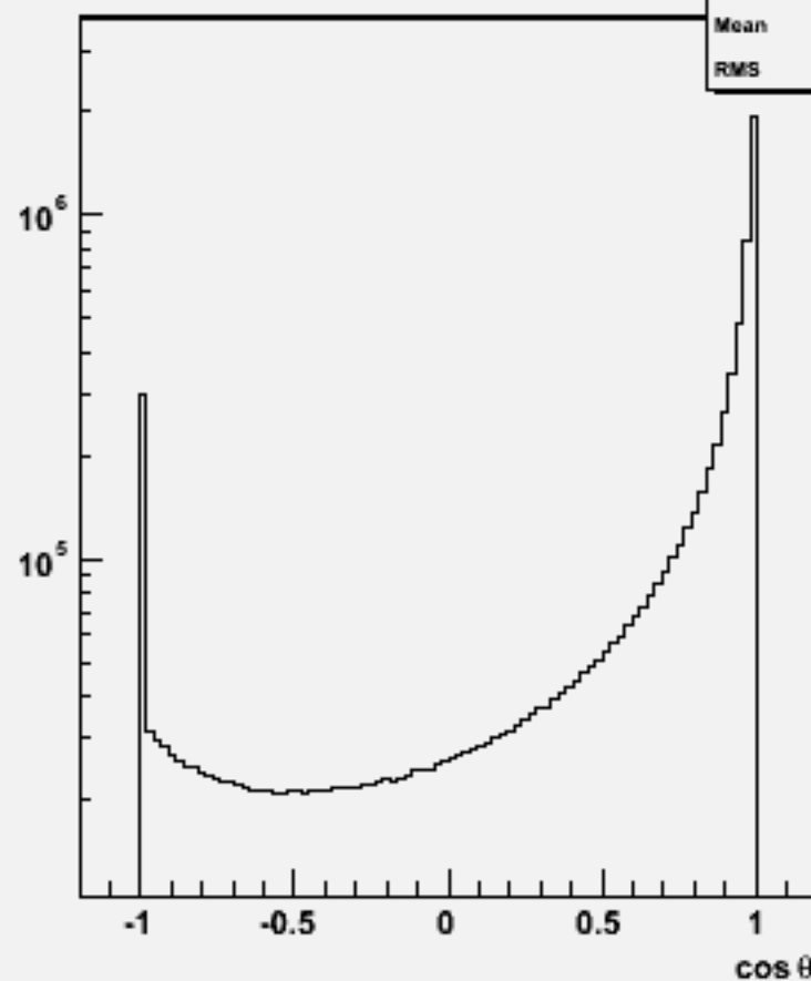
Particle cos \theta : w102855 e1a_e1dd_o
