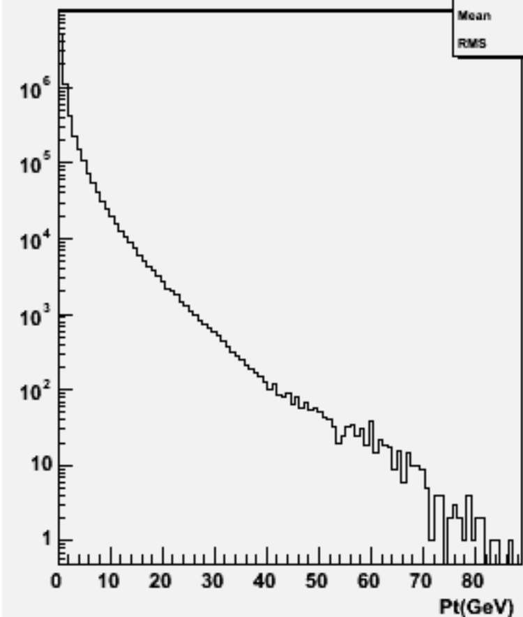
Particle Pt : w102855 e1a_e1dd_o
