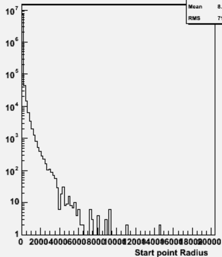
Start point R : w102855 e1a_e1dd_o
