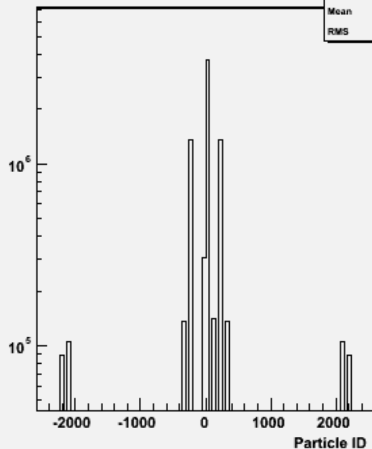
Particle ID : w102855 e1a_e1dd_o
