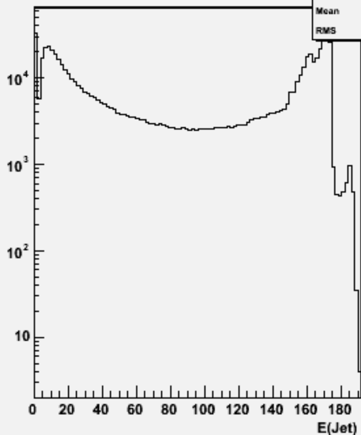
Jet energies(All jets)w102855 e1a_e1dd_o
