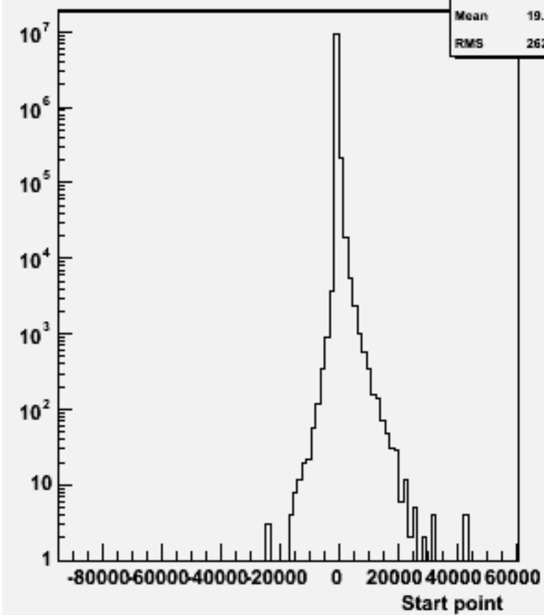
Start point Z : w102854 e1a_e1dd_o
