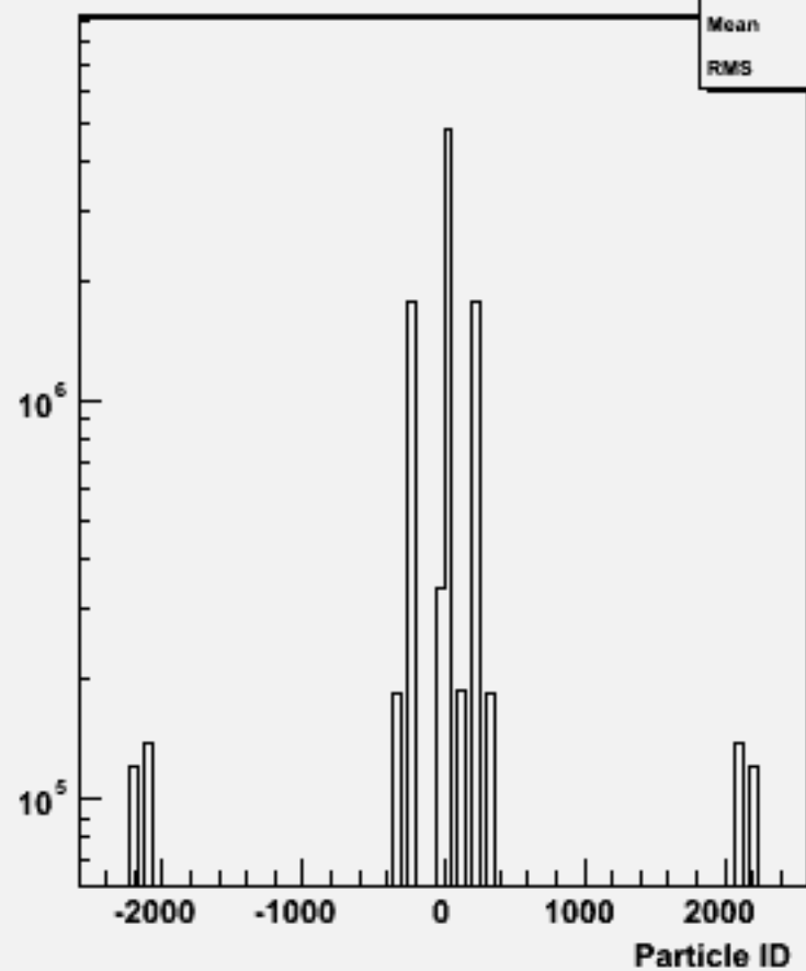
Particle ID : w102854 e1a_e1dd_o
