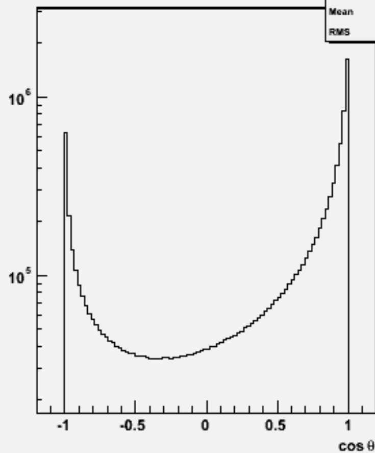
Particle cos \theta : w102854 e1a_e1dd_o
