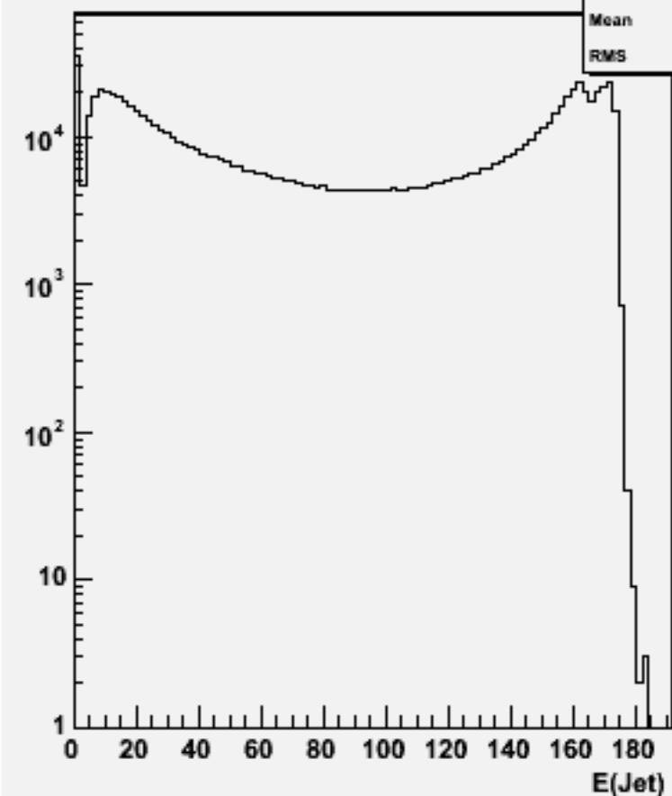
Jet energies(All jets)w102854 e1a_e1dd_o
