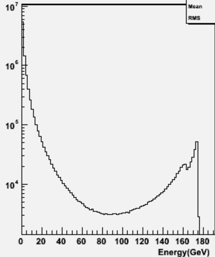
Particle Energy : w102854 e1a_e1dd_o
