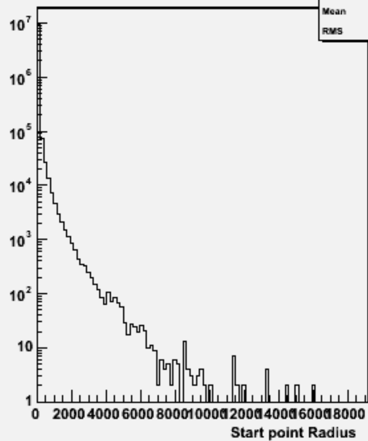
Start point R : w102854 e1a_e1dd_o
