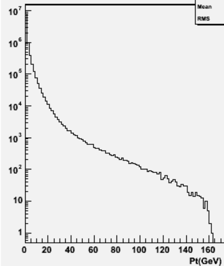
Particle Pt : w102854 e1a_e1dd_o
