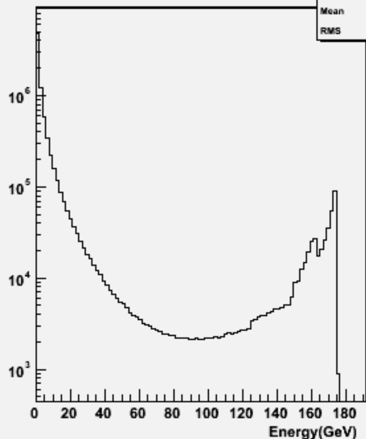
Particle Energy : w102853 e1a_e1dd_o
