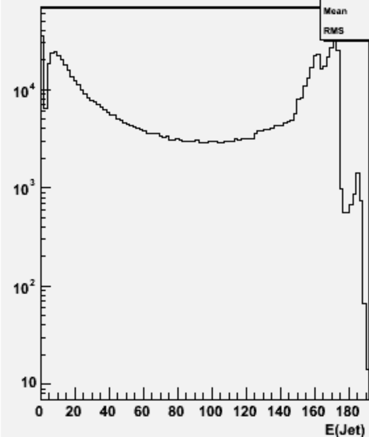
Jet energies(All jets)w102853 e1a_e1dd_o
