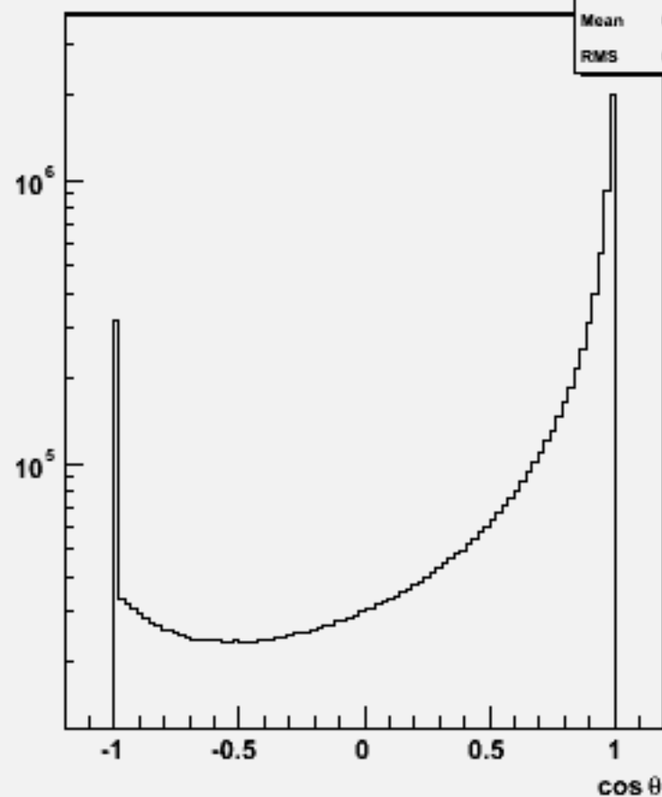
Particle cos \theta : w102853 e1a_e1dd_o
