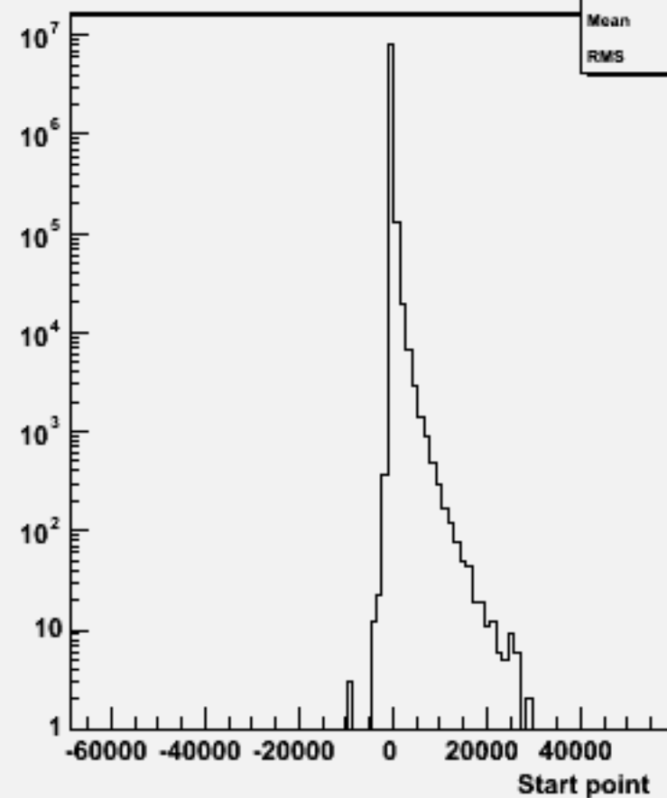
Start point Z : w102853 e1a_e1dd_o
