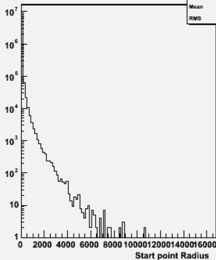
Start point R : w102853 e1a_e1dd_o
