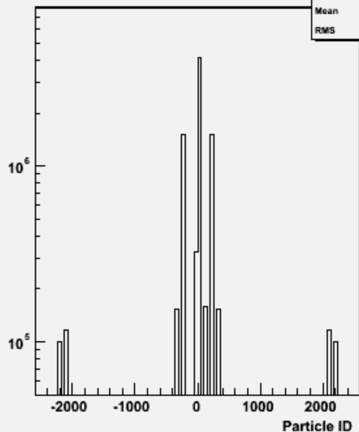
Particle ID : w102853 e1a_e1dd_o
