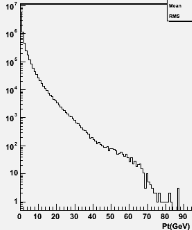
Particle Pt : w102853 e1a_e1dd_o
