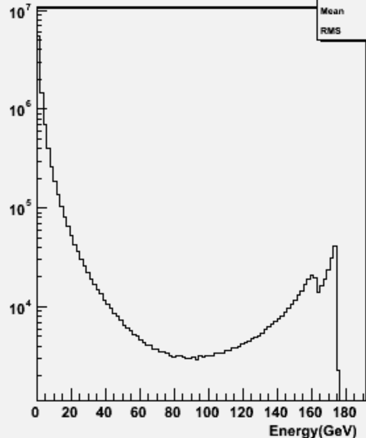
Particle Energy : w102852 e1a_e1dd_o
