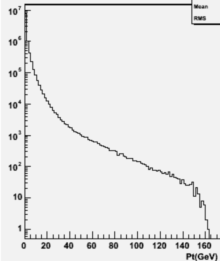
Particle Pt : w102852 e1a_e1dd_o
