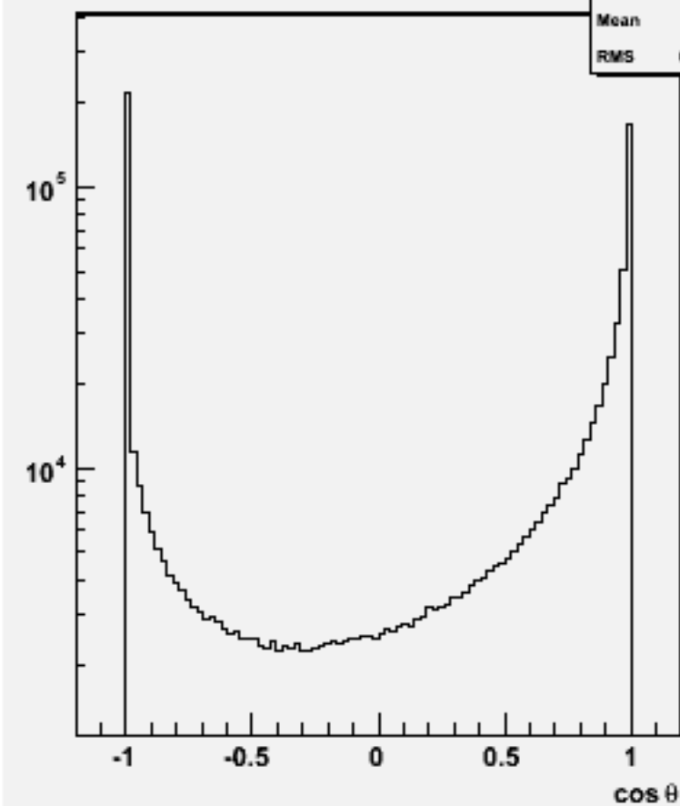
Jet cosθ (All jets)w102852 e1a_e1dd_o
