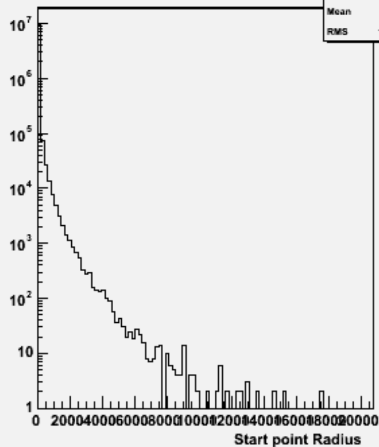
Start point R : w102852 e1a_e1dd_o
