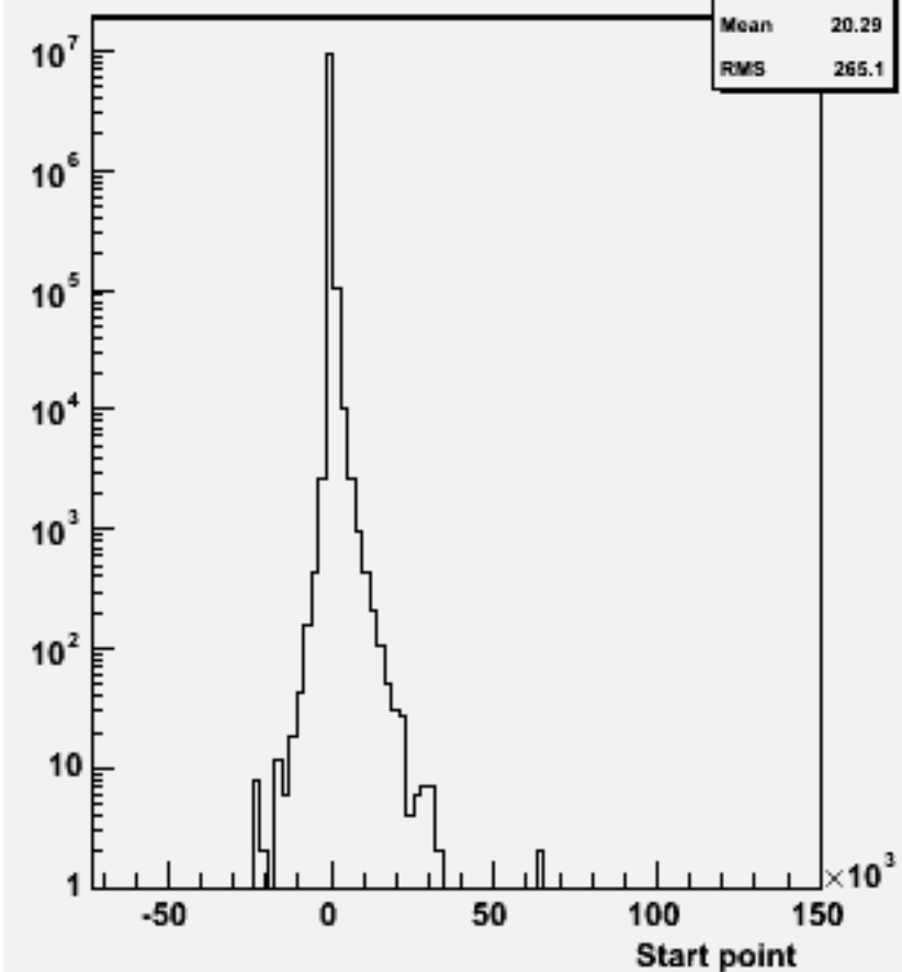
Start point Z : w102852 e1a_e1dd_o
