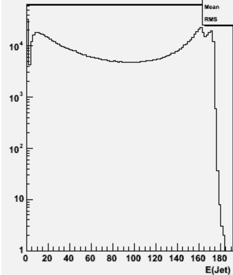
Jet energies(All jets)w102852 e1a_e1dd_o
