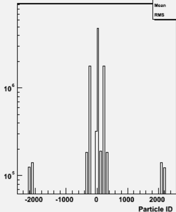
Particle ID : w102852 e1a_e1dd_o
