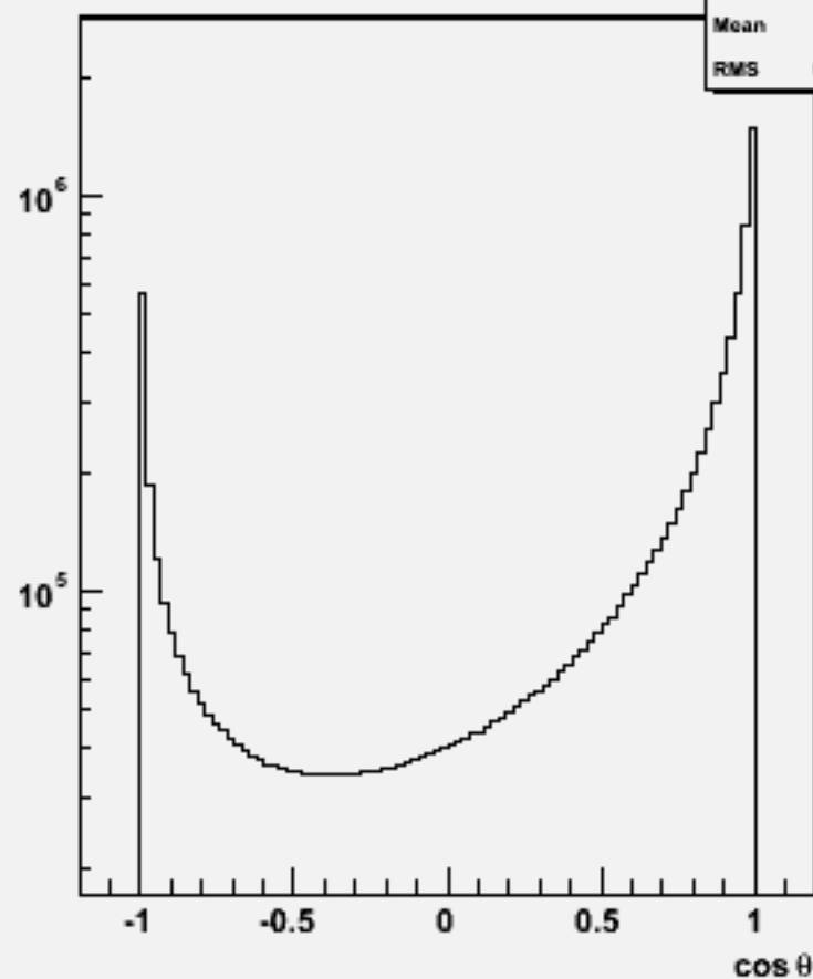
Particle cos \theta : w102852 e1a_e1dd_o
