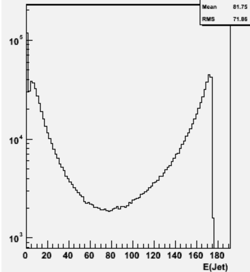
Jet energies(All jets)w102850 e1a_e1e3e3_o
