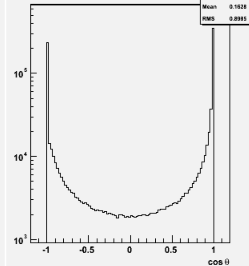
Jet cos \theta (All jets)w102850 e1a_e1e3e3_o
