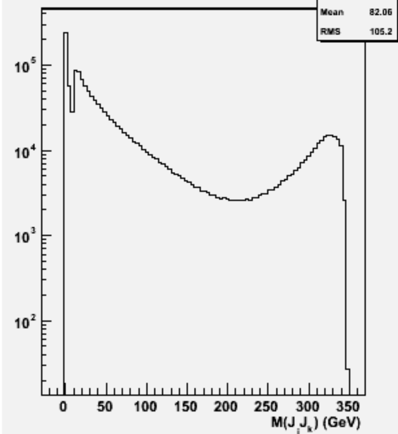
2jets mass(All comb)w102850 e1a_e1e3e3_o
