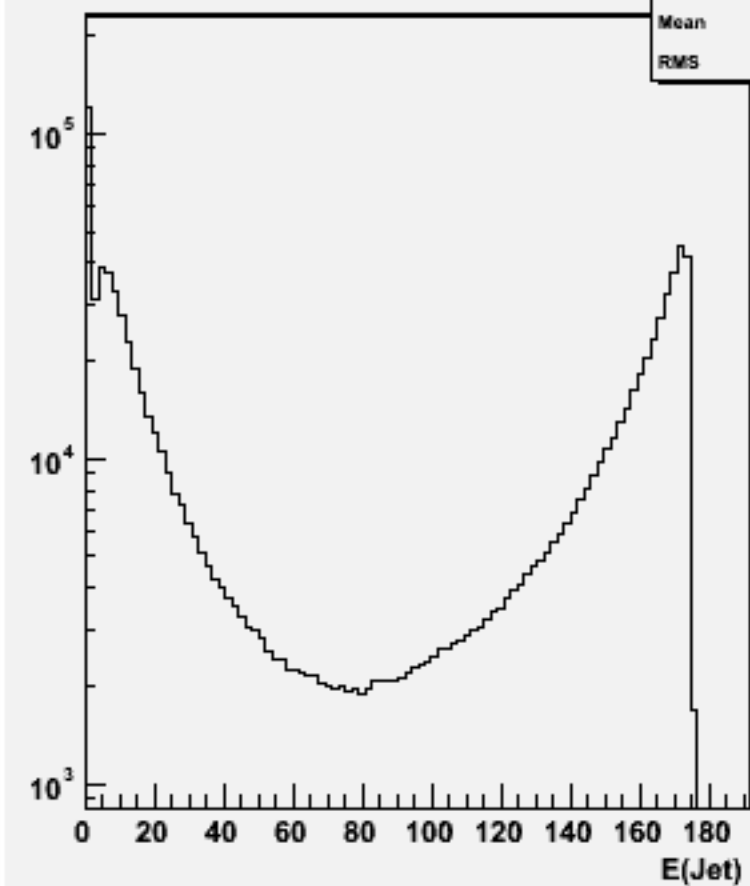
Jet energies(All jets)w102848 e1a_e1e3e3_o
