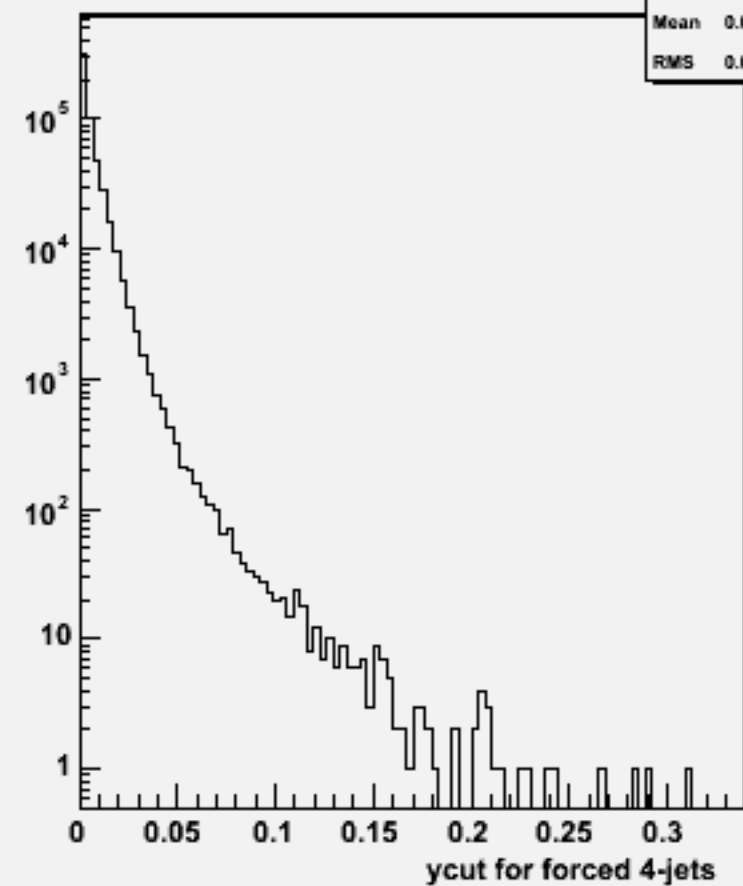
Ycut for 4-jets :w102846 e1a_e1e2e2_o
