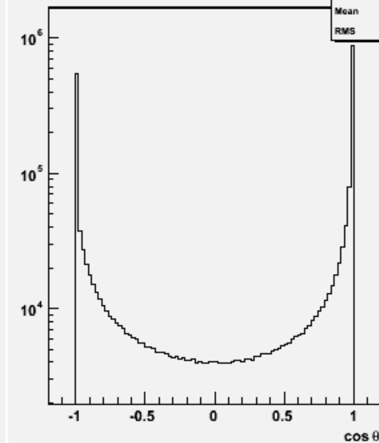
Jet cos \theta (All jets)w102846 e1a_e1e2e2_o
