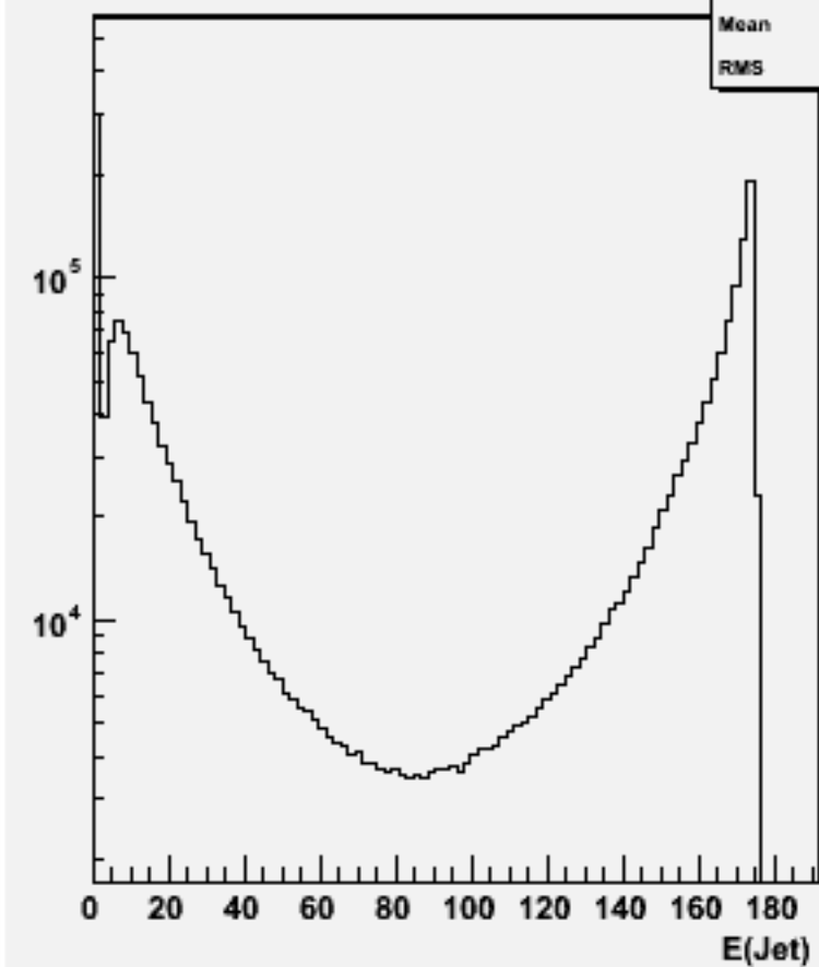
Jet energies(All jets)w102846 e1a_e1e2e2_o
