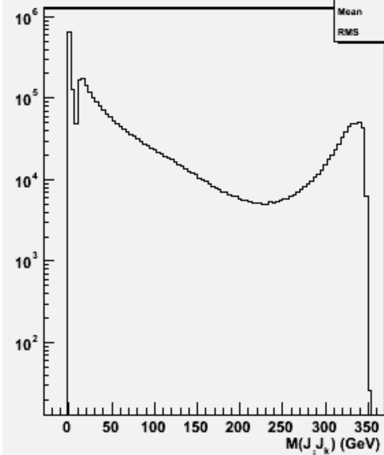
2jets mass(All comb)w102846 e1a_e1e2e2_o
