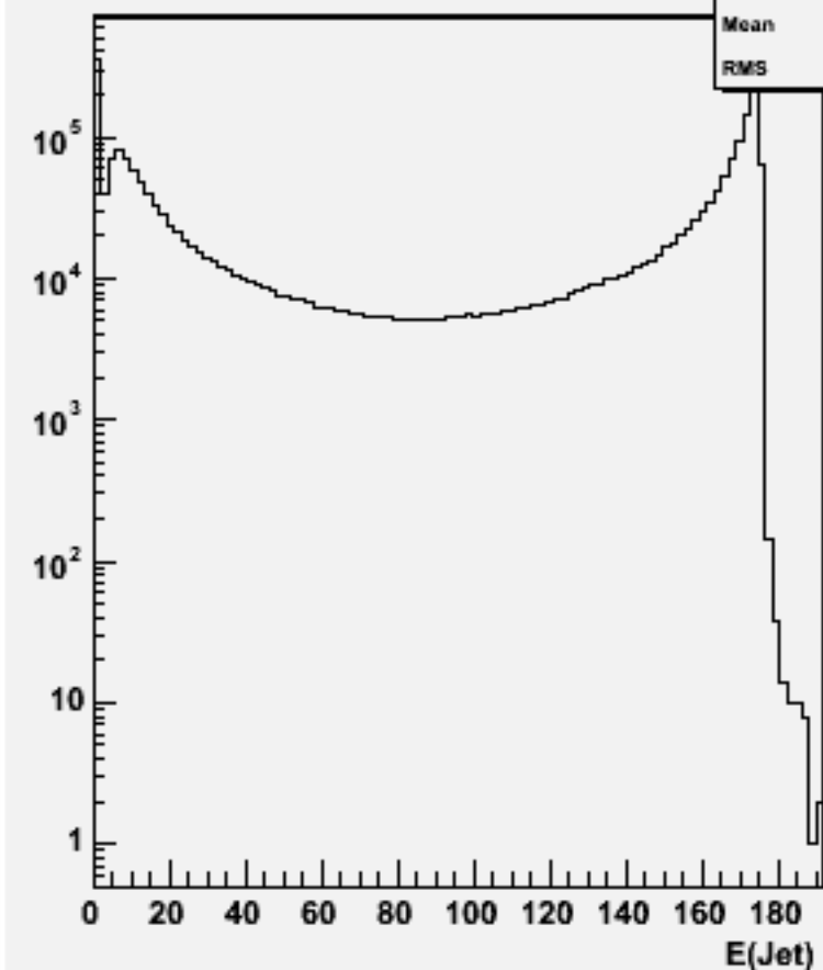
Jet energies(All jets)w102845 e1a_e1e2e2_o
