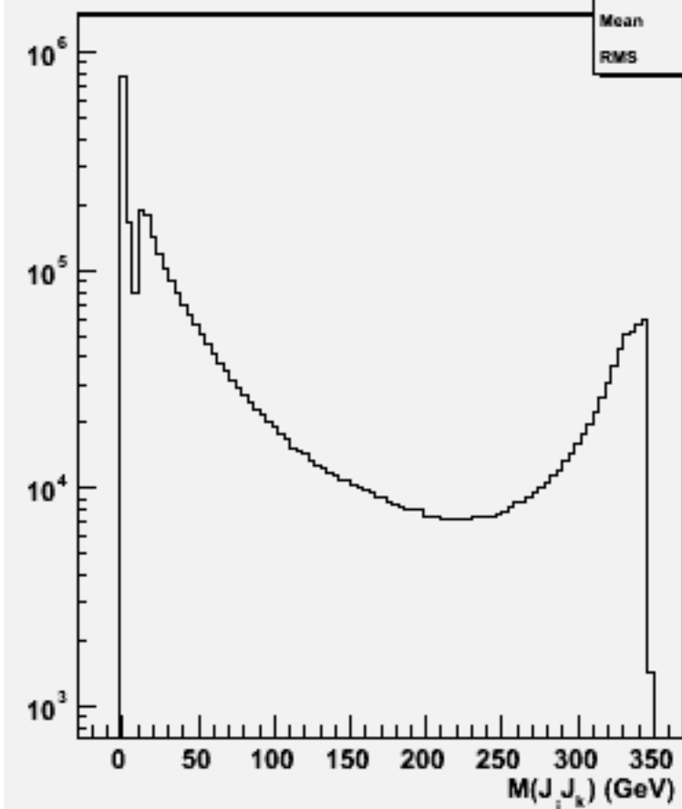
2jets mass(All comb)w102845 e1a_e1e2e2_o
