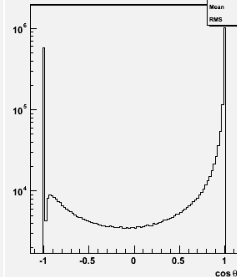
Jet cos \theta (All jets)w102845 e1a_e1e2e2_o
