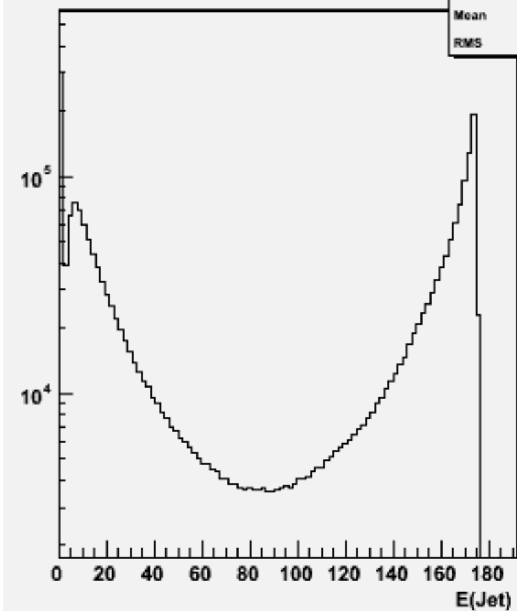
Jet energies(All jets)w102844 e1a_e1e2e2_o
