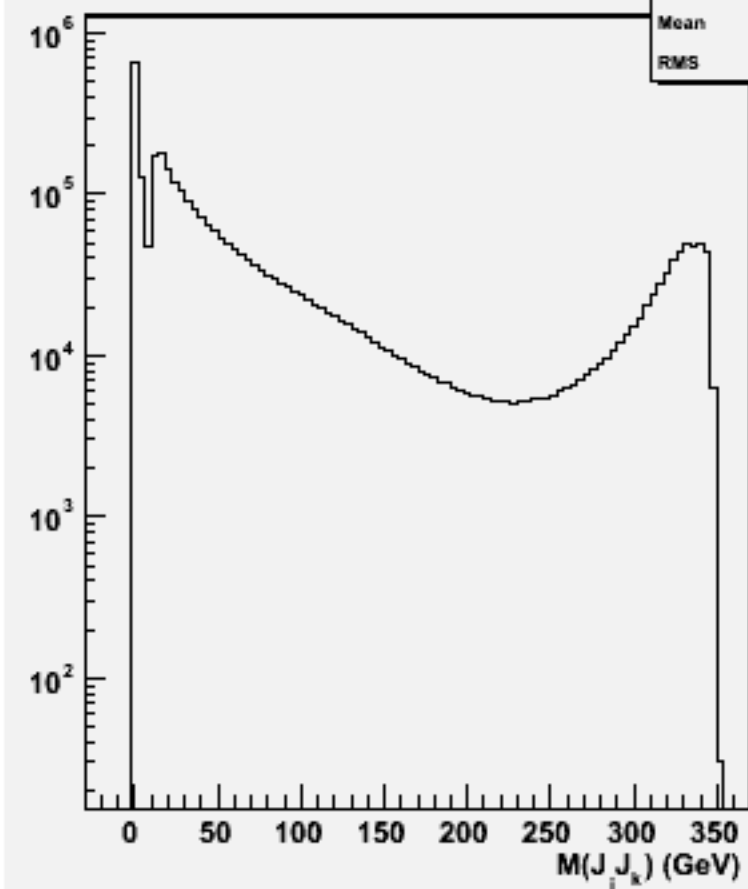
2jets mass(All comb)w102844 e1a_e1e2e2_o
