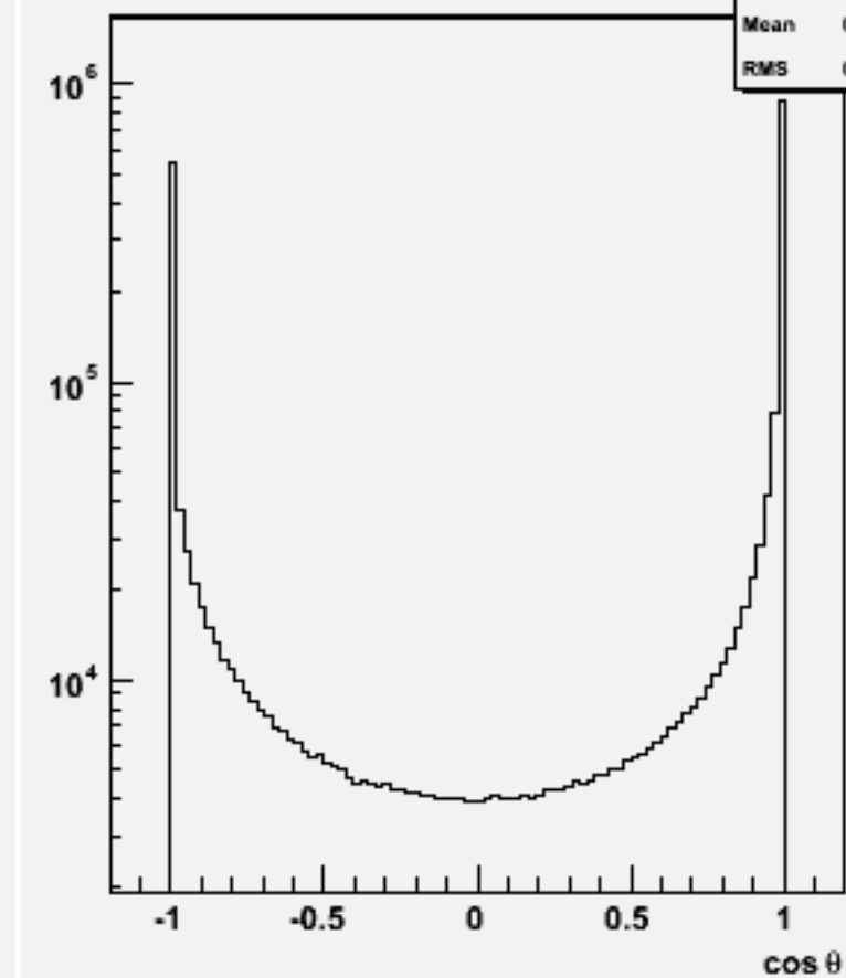
Jet cos \theta (All jets)w102844 e1a_e1e2e2_o
