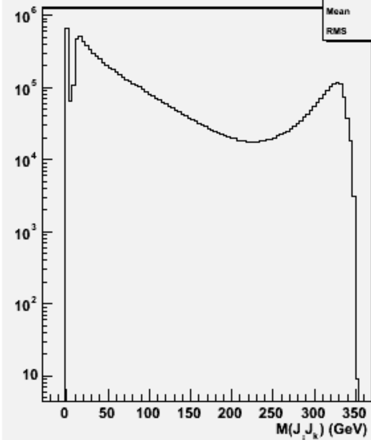
2jets mass(All comb)w102840 e1a_e1e1e1_o
