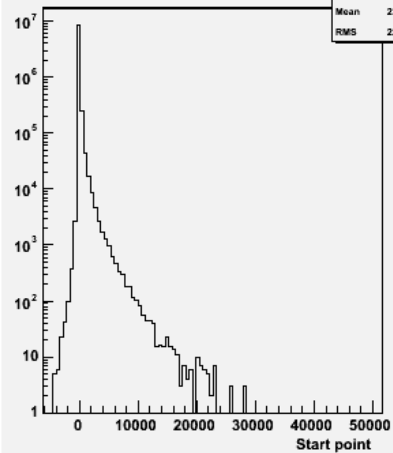
Start point Z : w102839 e1a_e1cc_o
