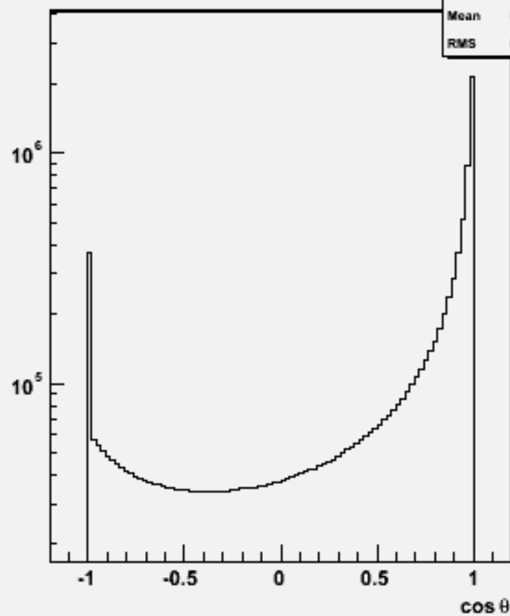
Particle cosθ : w102839 e1a_e1cc_o
