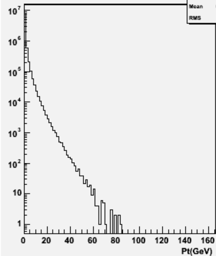
Particle Pt : w102839 e1a_e1cc_o
