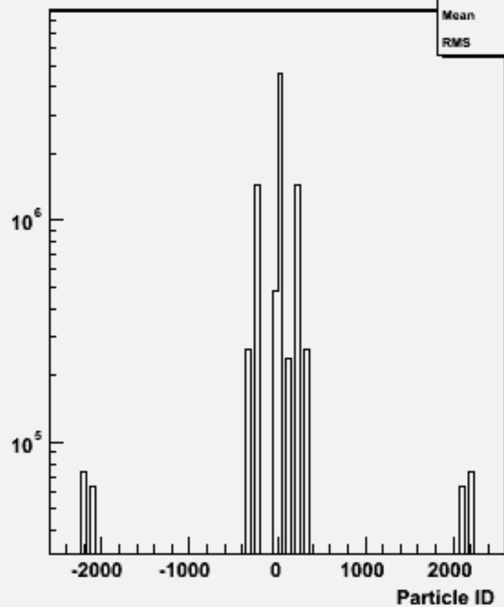
Particle ID : w102839 e1a_e1cc_o
