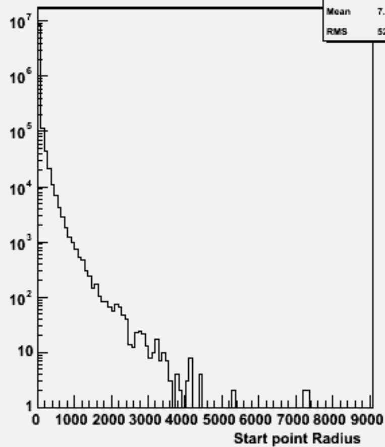
Start point R : w102839 e1a_e1cc_o
