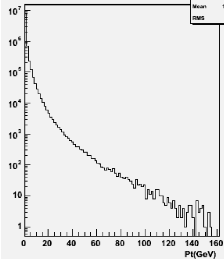
Particle Pt : w102838 e1a_e1cc_o
