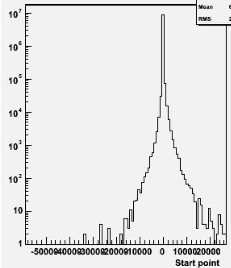
Start point Z : w102838 e1a_e1cc_o
