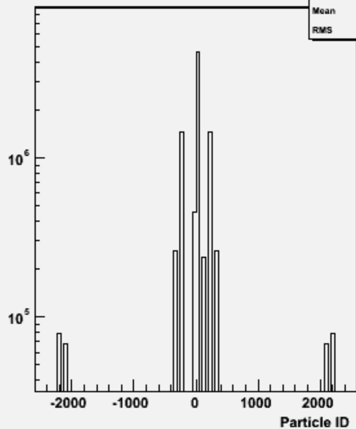
Particle ID : w102838 e1a_e1cc_o
