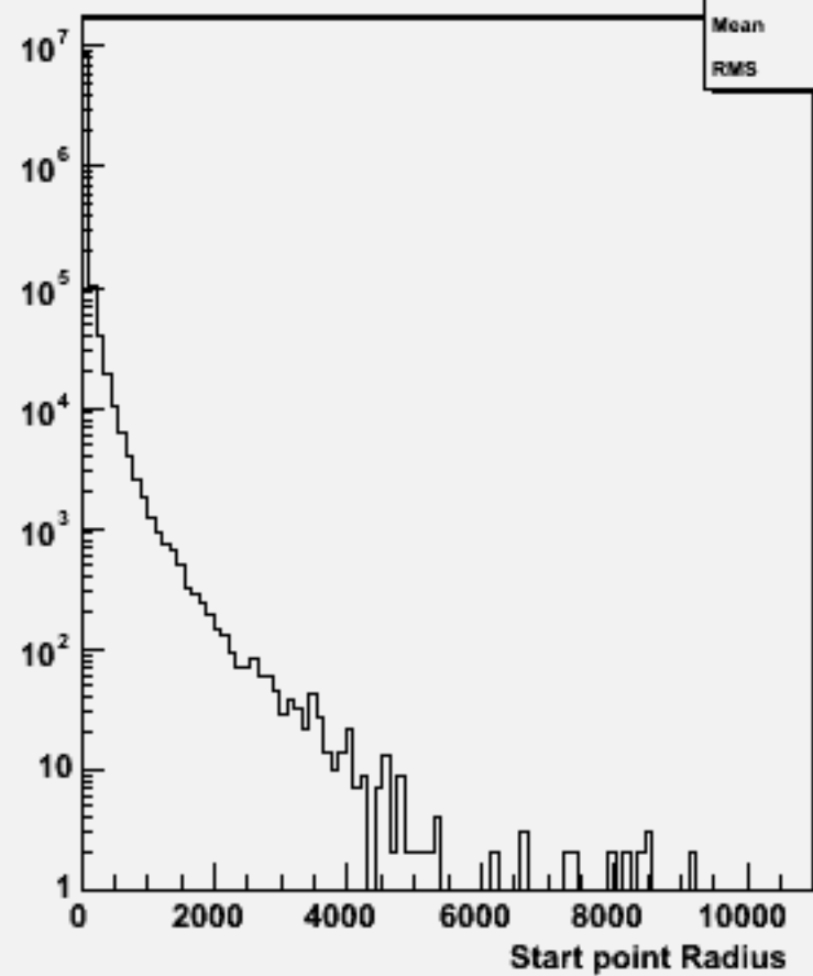
Start point R : w102838 e1a_e1cc_o
