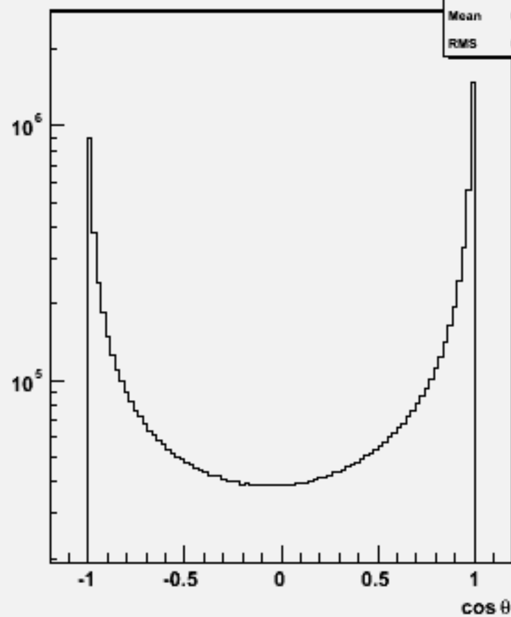
Particle cos \theta : w102838 e1a_e1cc_o
