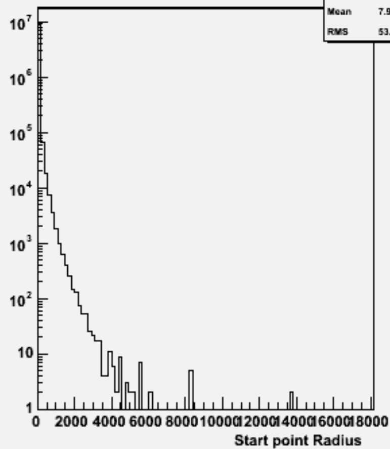
Start point R : w102837 e1a_e1cc_o
