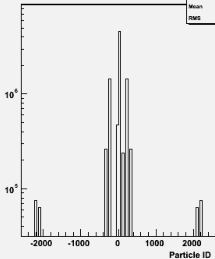
Particle ID : w102837 e1a_e1cc_o
