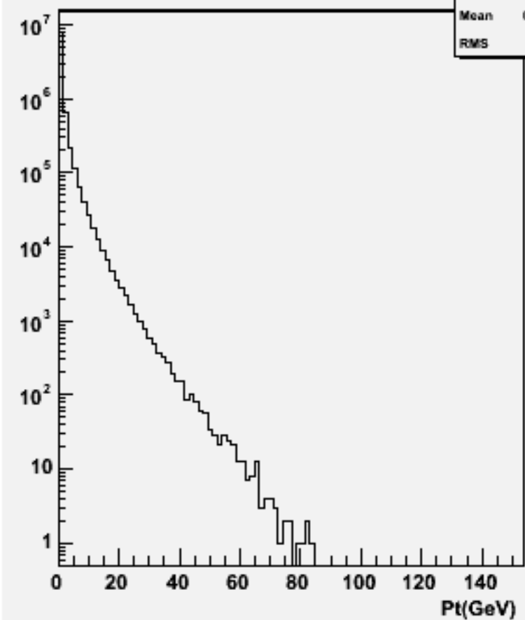
Particle Pt : w102837 e1a_e1cc_o
