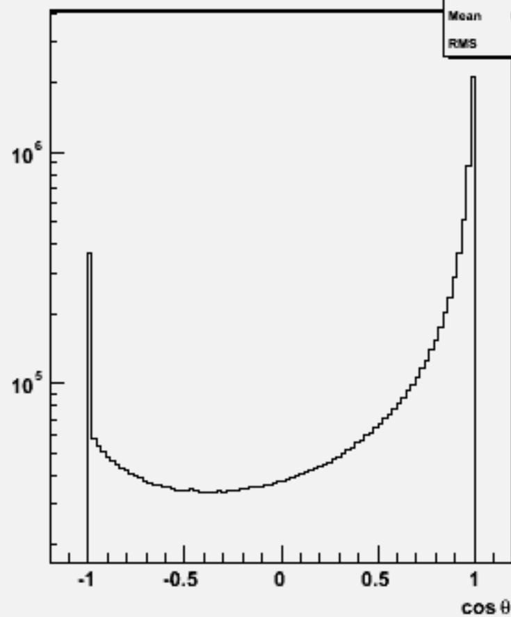
Particle cosθ : w102837 e1a_e1cc_o
