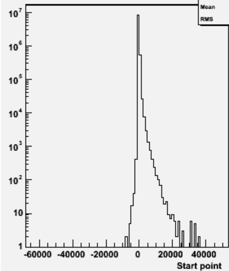
Start point Z : w102837 e1a_e1cc_o
