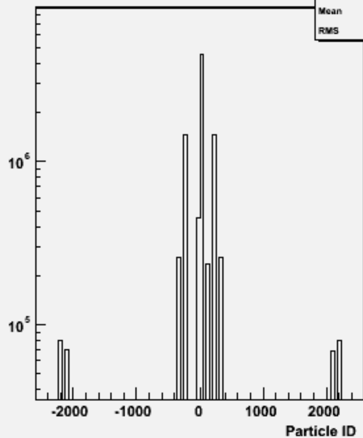
Particle ID : w102836 e1a_e1cc_o
