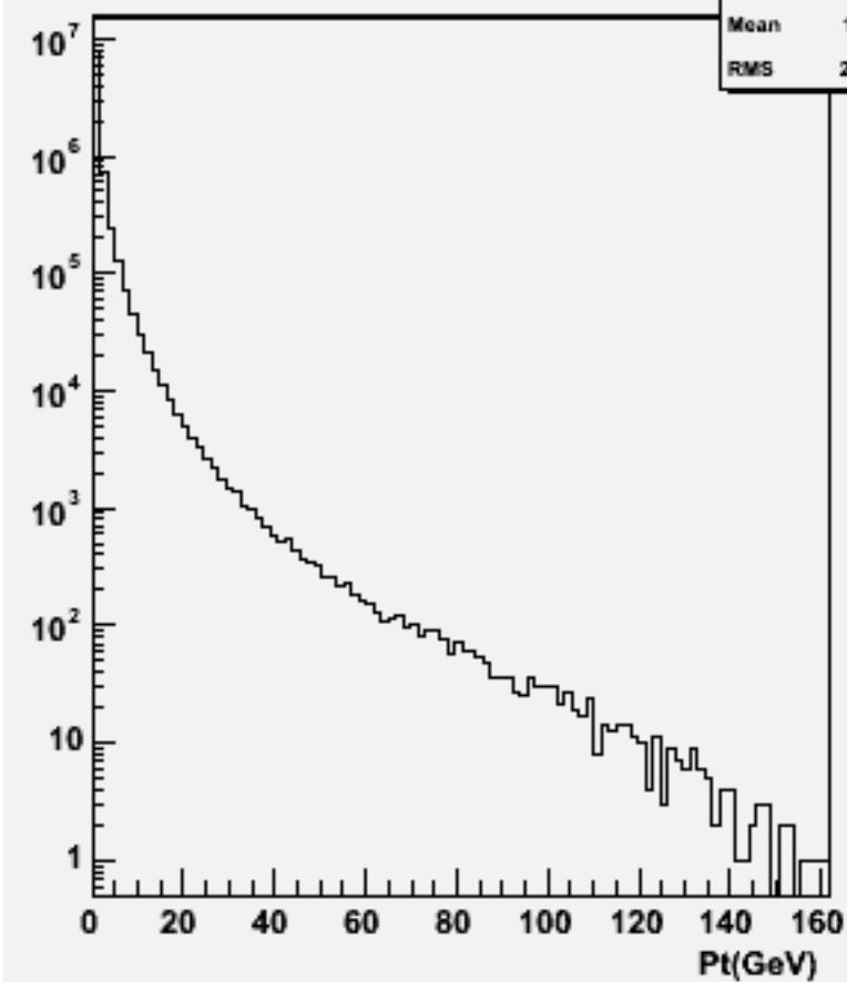
Particle Pt : w102836 e1a_e1cc_o
