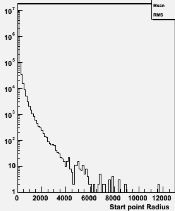
Start point R : w102836 e1a_e1cc_o
