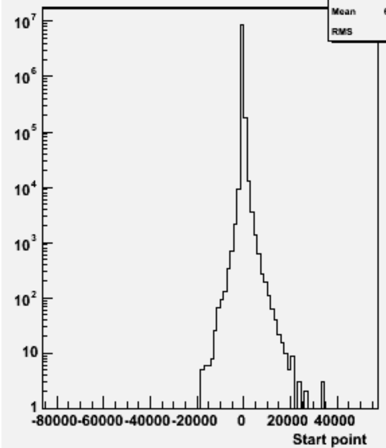
Start point Z : w102836 e1a_e1cc_o
