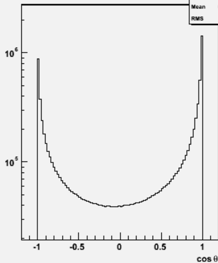
Particle cos \theta : w102836 e1a_e1cc_o
