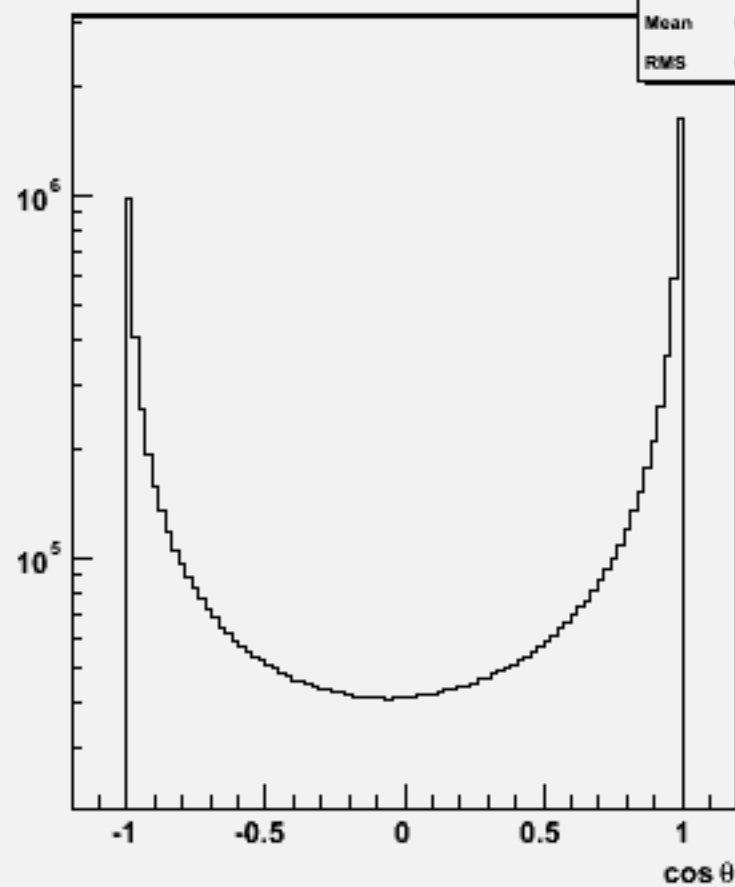
Particle cos \theta : w102834 e1a_e1uu_o
