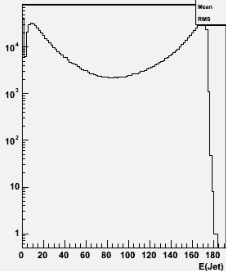
Jet energies(All jets)w102834 e1a_e1uu_o
