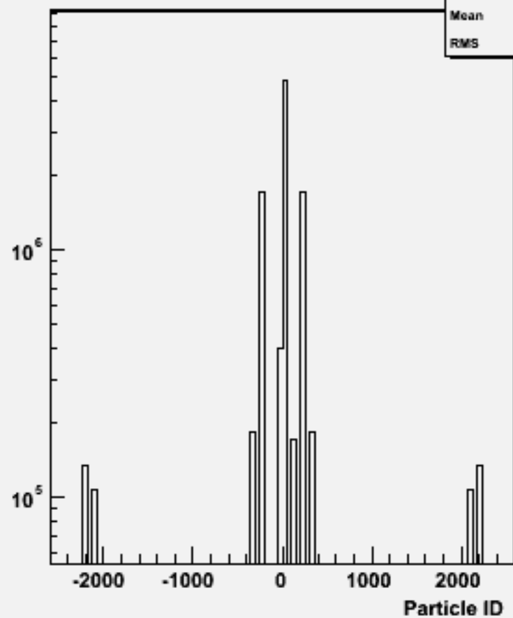
Particle ID : w102834 e1a_e1uu_o
