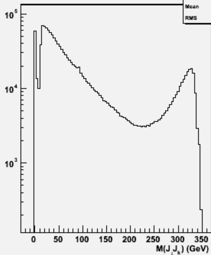
2jets mass(All comb)w102834 e1a_e1uu_o
