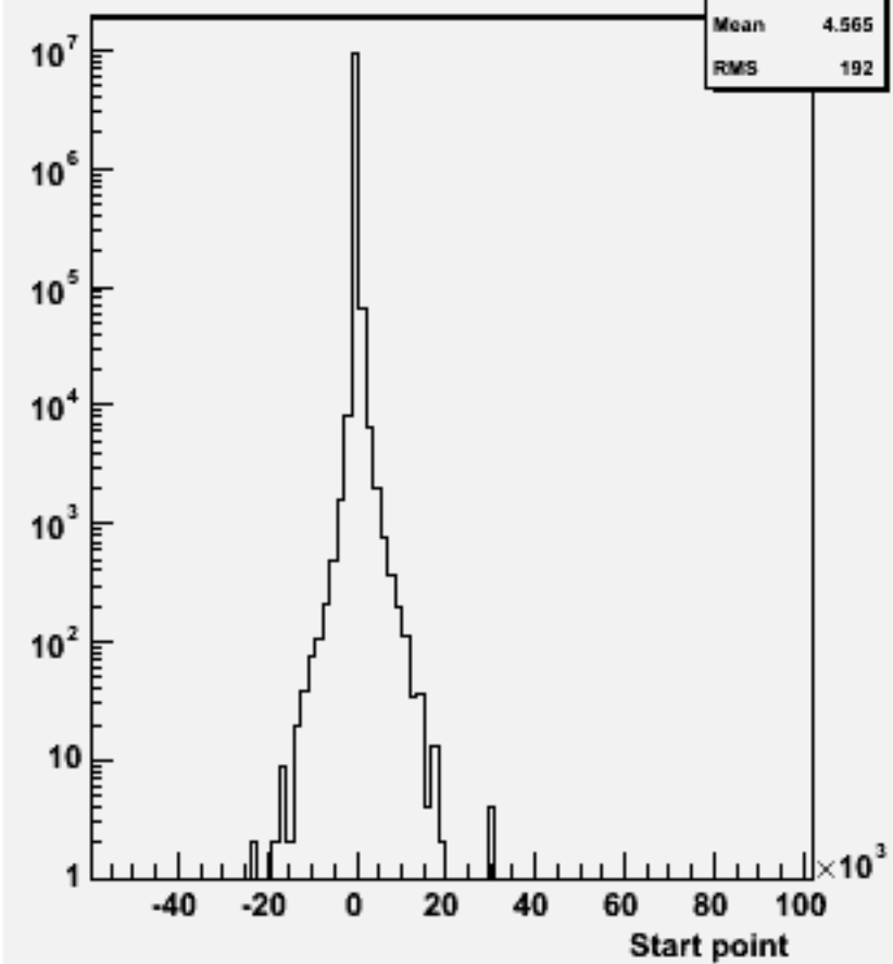
Start point Z : w102834 e1a_e1uu_o
