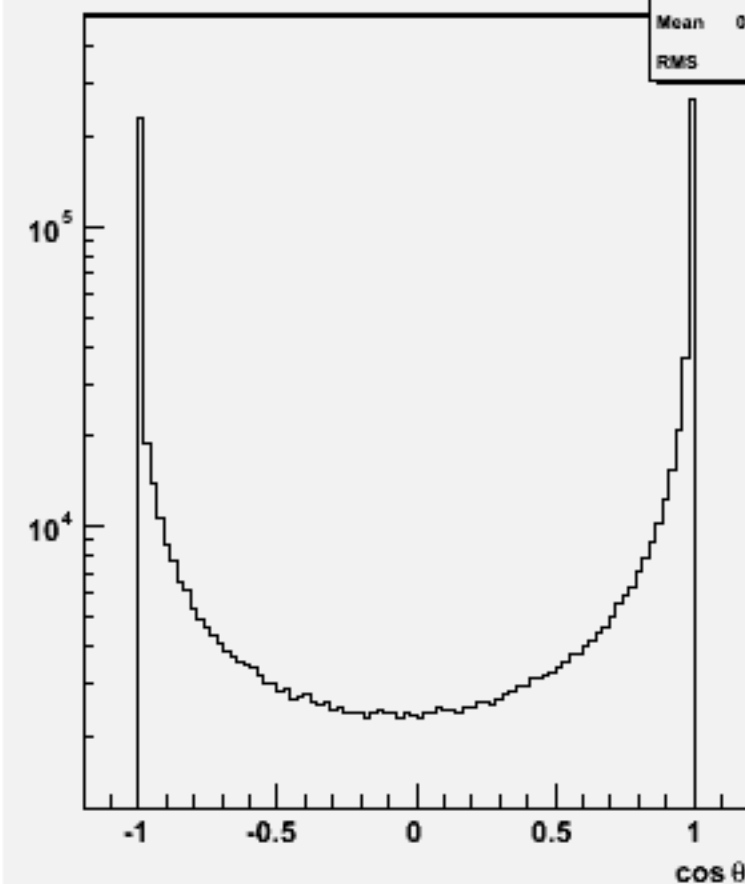
Jet cosθ (All jets)w102834 e1a_e1uu_o
