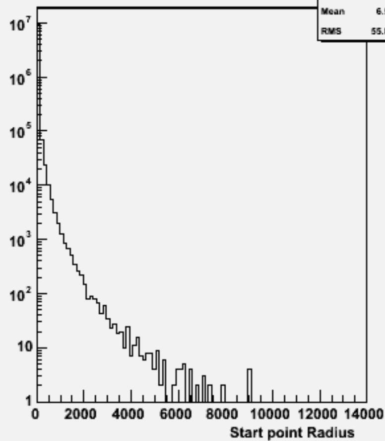
Start point R : w102834 e1a_e1uu_o
