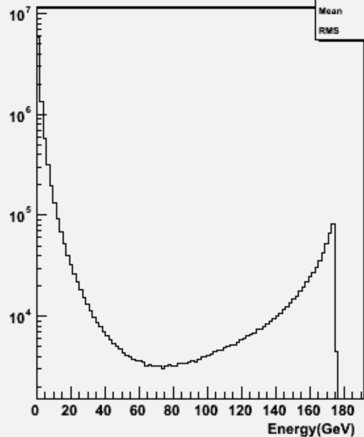
Particle Energy : w102834 e1a_e1uu_o
