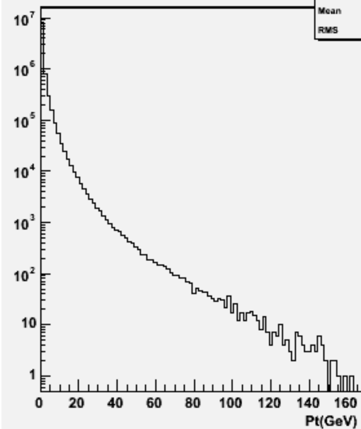
Particle Pt : w102834 e1a_e1uu_o
