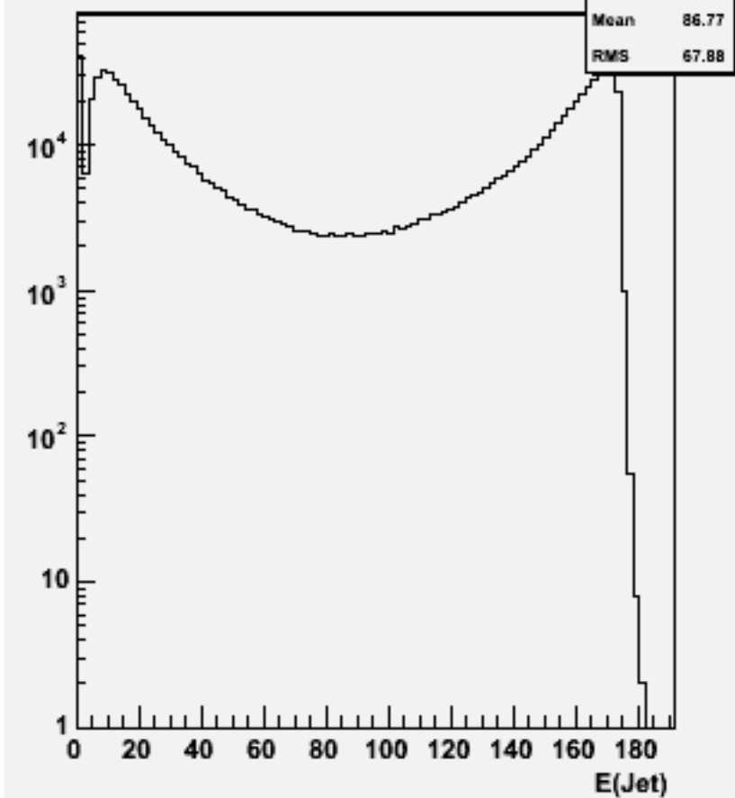
Jet energies(All jets)w102832 e1a_e1uu_o
