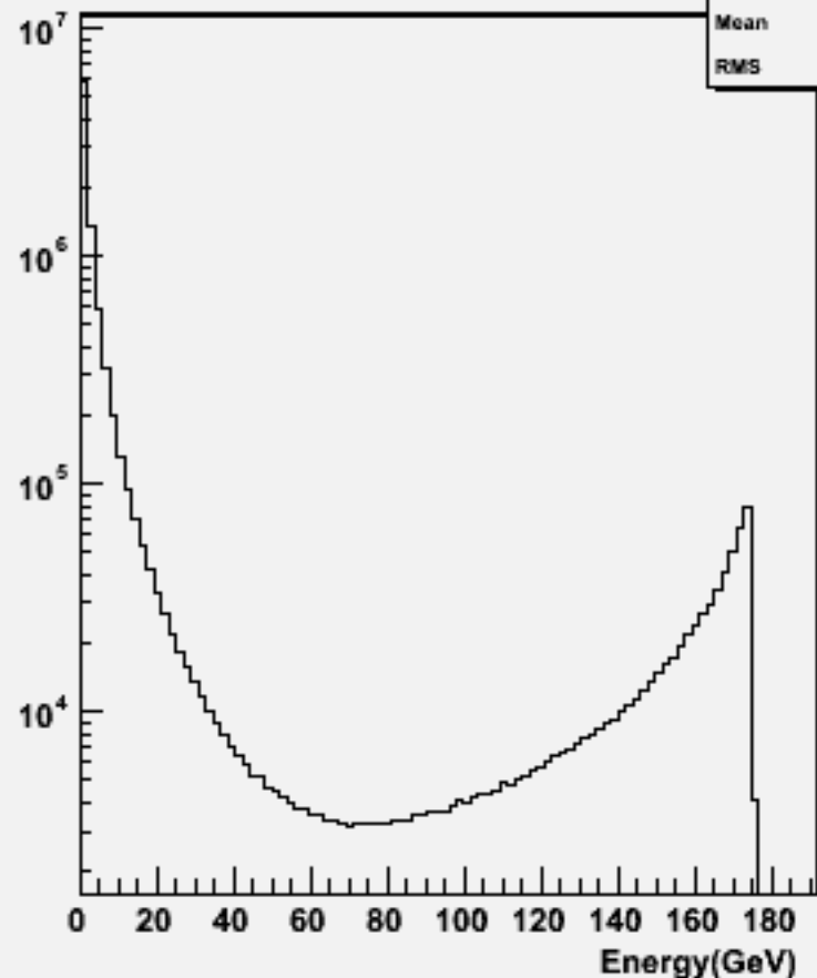
Particle Energy : w102832 e1a_e1uu_o
