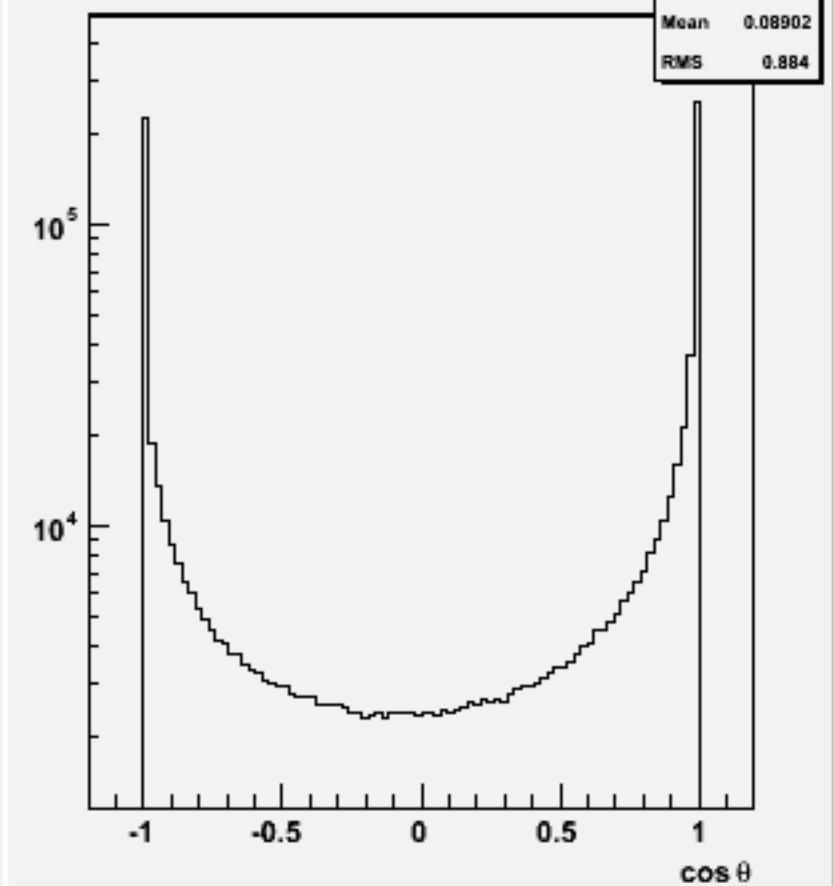
Jet cosθ (All jets)w102832 e1a_e1uu_o
