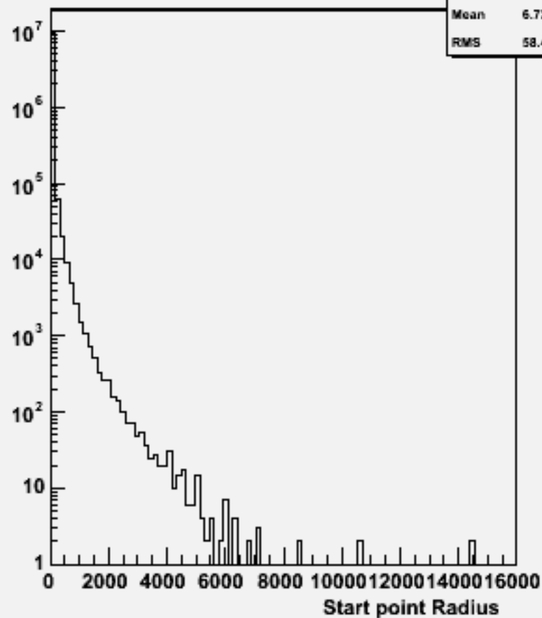
Start point R : w102832 e1a_e1uu_o
