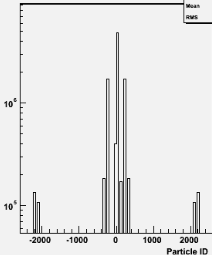
Particle ID : w102832 e1a_e1uu_o
