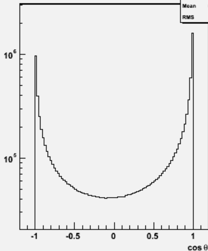
Particle \cos \theta : w102832 e1a_e1uu_o
