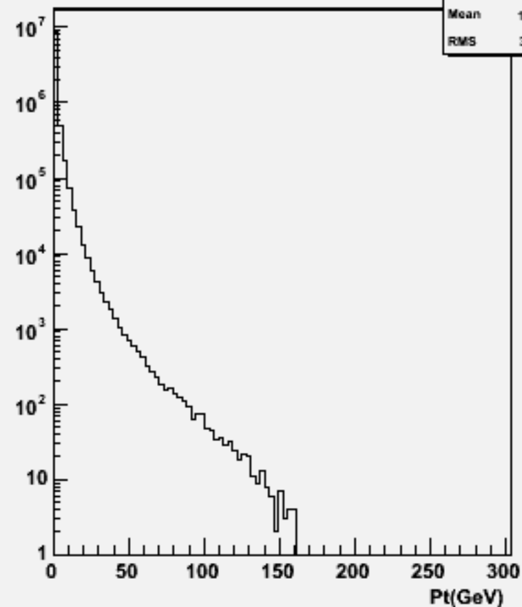
Particle Pt : w102832 e1a_e1uu_o
