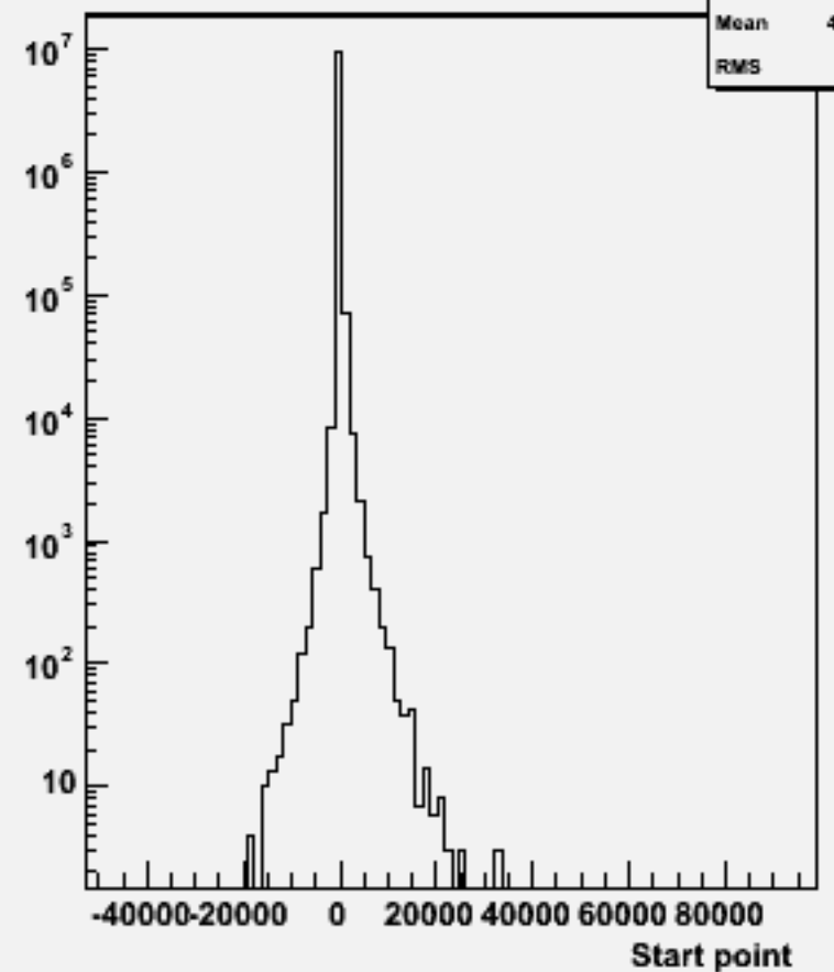
Start point Z : w102832 e1a_e1uu_o
