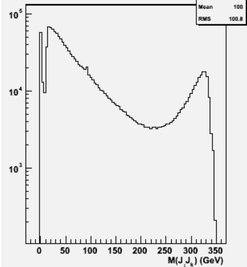
2jets mass(All comb)w102832 e1a_e1uu_o
