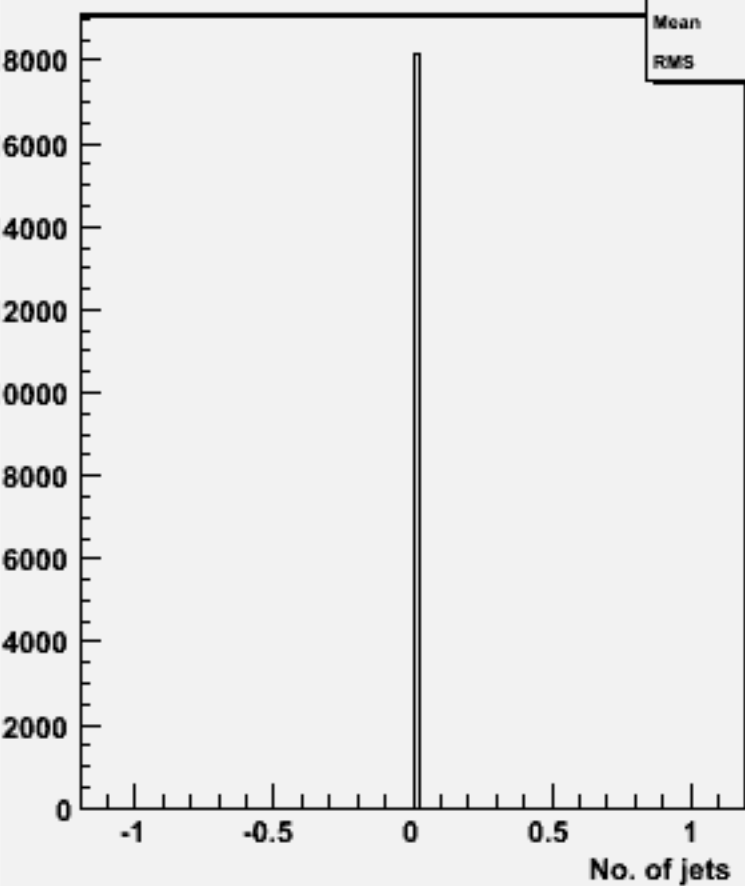
No. jets (ycut=0.001) : w102831 e1a_e1n3n3_o
