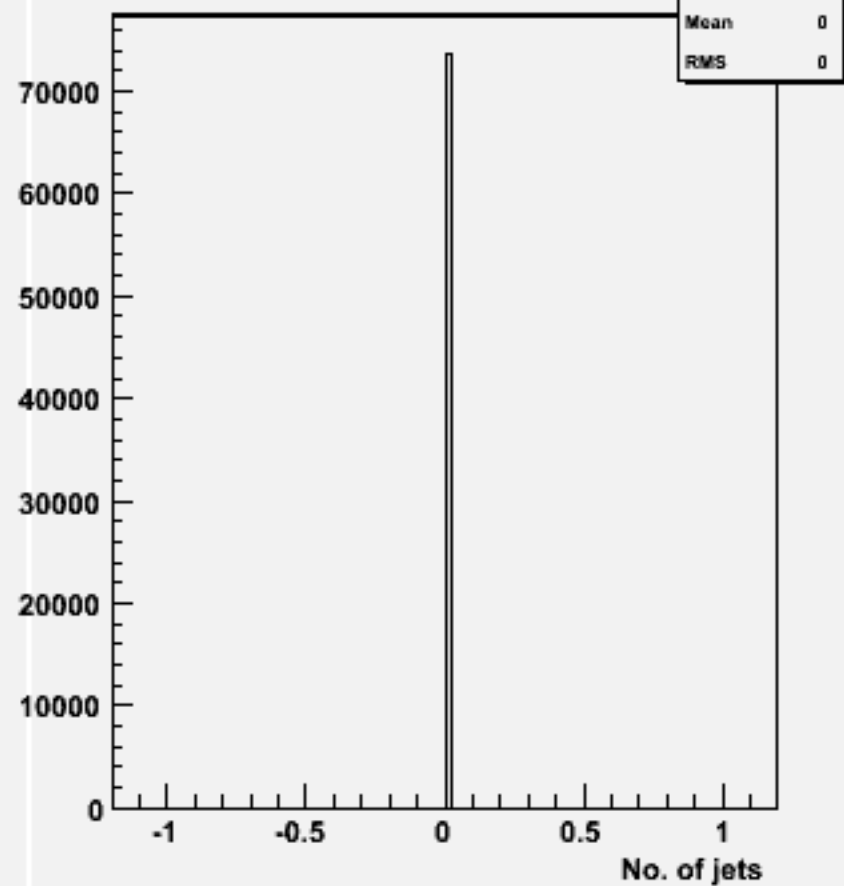
No. jets (ycut=0.001) : w102828 e1a_e1n3n3_o
